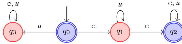
Figure 4.9 – Un exemple d'états sûrs / non-sûrs
