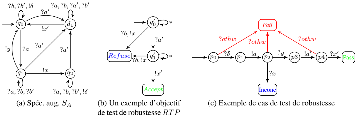
Figure 2.6 – Génération de cas de test de robustesse
