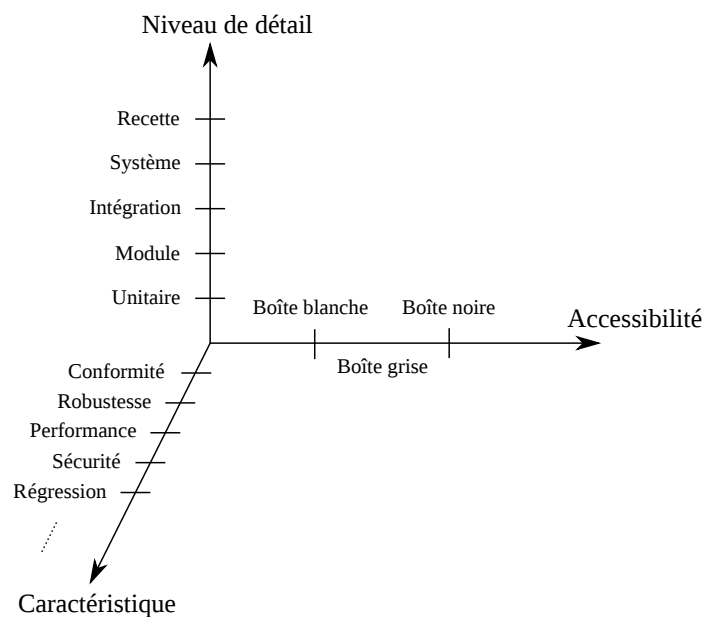
Figure 1.2 – Classification des différents types de test actif (inspirée de Tretmans)
