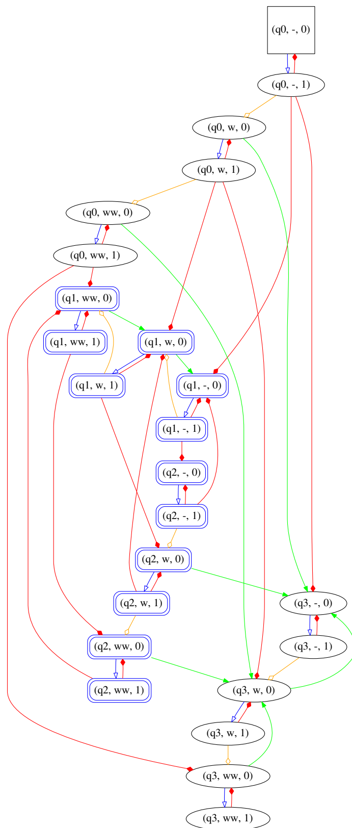
Figure 4.11 – Graphe de jeu associé à la propriété \varphi_4
