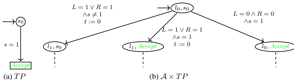
Figure 2.12 – Exemple partiel de produit synchronisé entre deux VDTA
