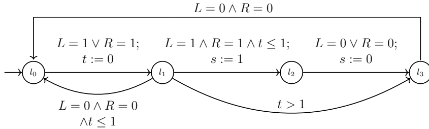
Figure 2.9 – VDTA modélisant la commande bi-manuelle
