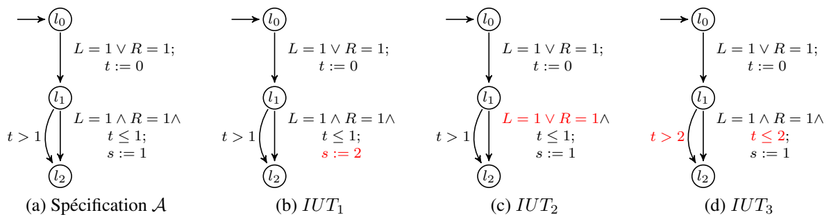
Figure 2.10 – tvco par l'exemple.
