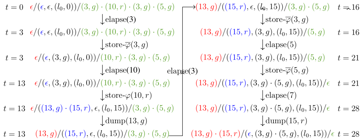
Figure 4.7 – Evolution de l' EM avec la séquence d'entrée \sigma = (3, g) \cdot (10, r) \cdot (3, g) \cdot (5, g) pour \varphi_3
