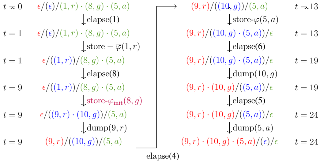
Figure 4.5 – Evolution de l'EM de co-safety avec la séquence d'entrée (1, r) \cdot (8, g) \cdot (5, a) pour \varphi_2
