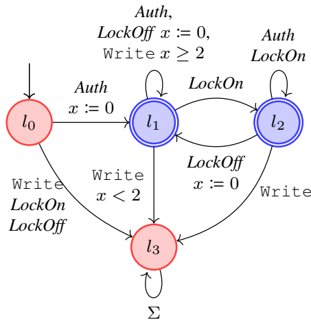
Figure 4.13 – Propriété \varphi_5 modélisée par le TA \mathcal{A}_{\varphi_5}
