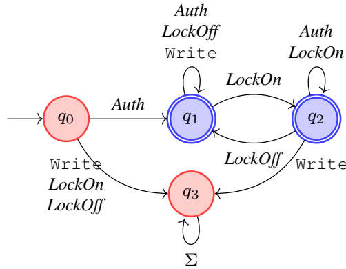
Figure 4.8 – Automate \mathcal{A}_{\varphi_4} modélisant la propriété \varphi_4
