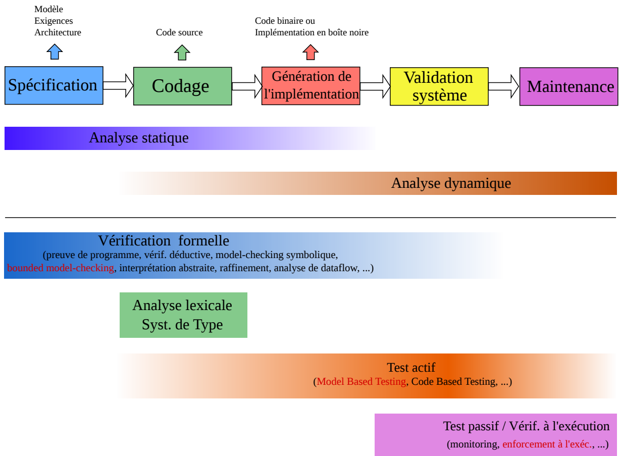
Figure 1.1 – Positionnement des principales méthodes de vérification / test (et de mes contributions (en caractères rouges sur la figure))
