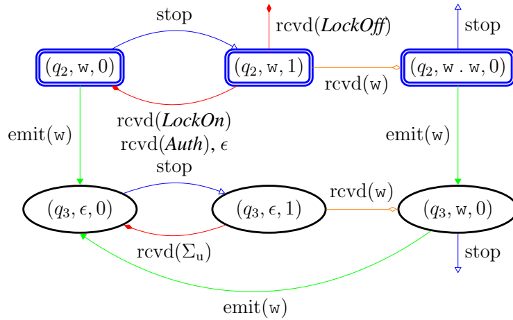
Figure 4.12 – Zoom sur certains nœuds et certaines arrêtes du graphe de jeu associé à \varphi_4
