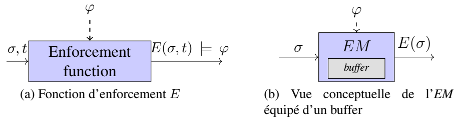
Figure 4.2 – Vues conceptuelle et fonctionnelle d'un EM
