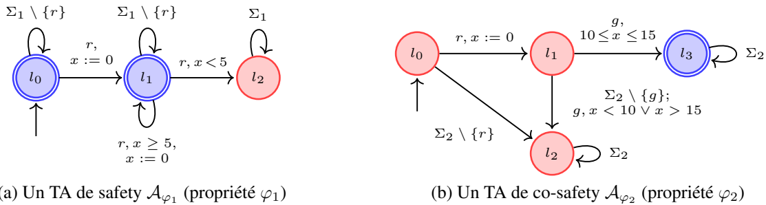
Figure 4.3 – Exemples de propriétés temporisées
