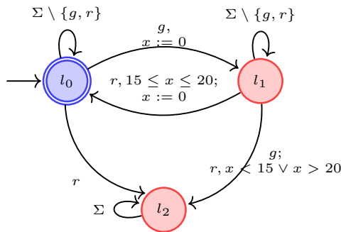
Figure 4.6 – Un TA quelconque \mathcal{A}_{\varphi_3} (propriété \varphi_3 régulière).
