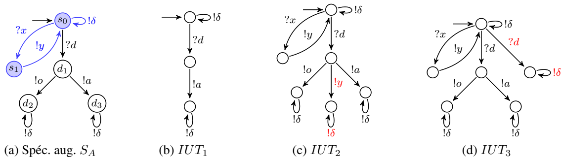
Figure 2.7 – relation robust par l'exemple.
