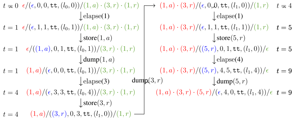
Figure 4.4 – Evolution de l'EM de safety avec la séquence d'entrée (1, a) \cdot (3, r) \cdot (1, r) pour \varphi_1
