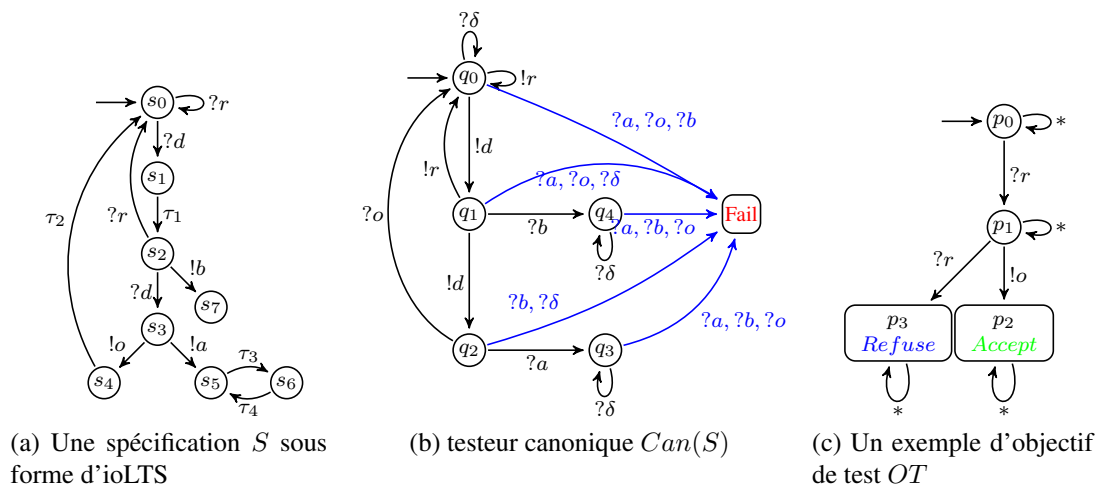
Figure 2.3 – Quelques éléments utilisés dans les méthodes de test à base d'ioLTS
