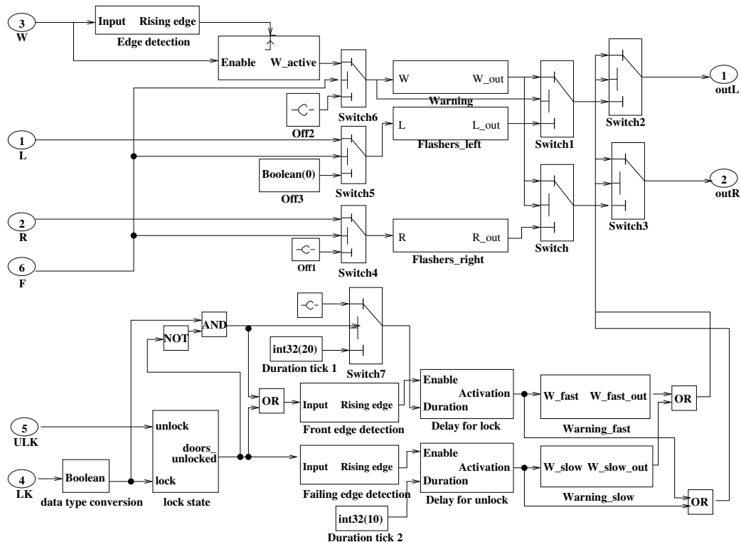
Figure 3.4 – Modèle Simulink détaillé du FlashManager
