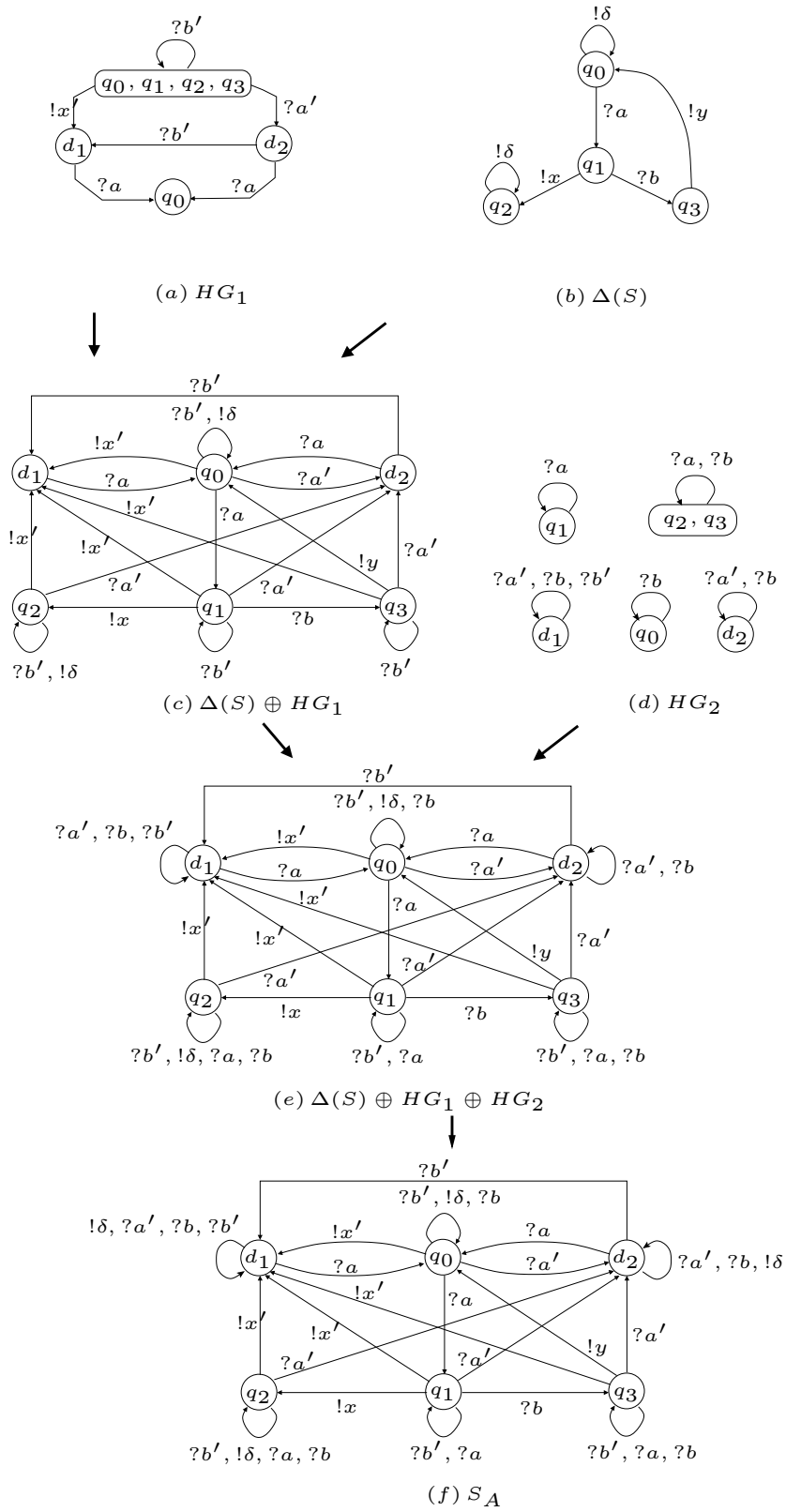
Figure 2.5 – Exemple de construction de spécification augmentée (extrait de [C10])
