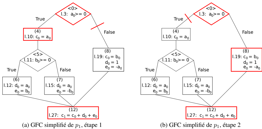
Figure 3.2 – Chemins explorés par la stratégie de recherche dynamique en backjump pour la propriété p_1
