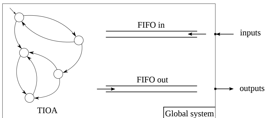
Figure 2.15 – Principe de la sémantique asynchrone
