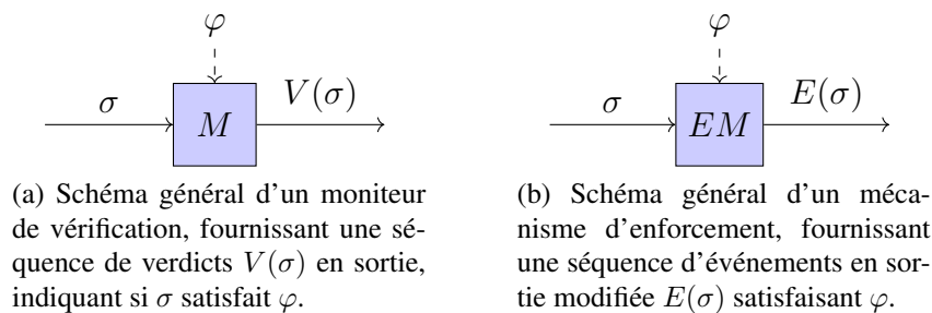
Figure 4.1 – Schéma montrant la différence conceptuelle entre un moniteur de vérification M et un mécanisme d'enforcement EM .
