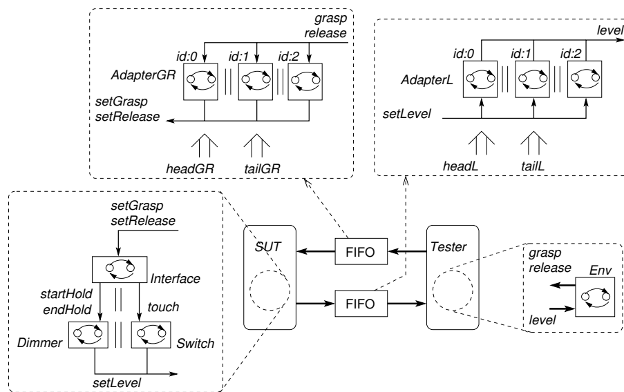
Figure 2.16 – Schéma de test pour l'exemple du "Light Controller"
