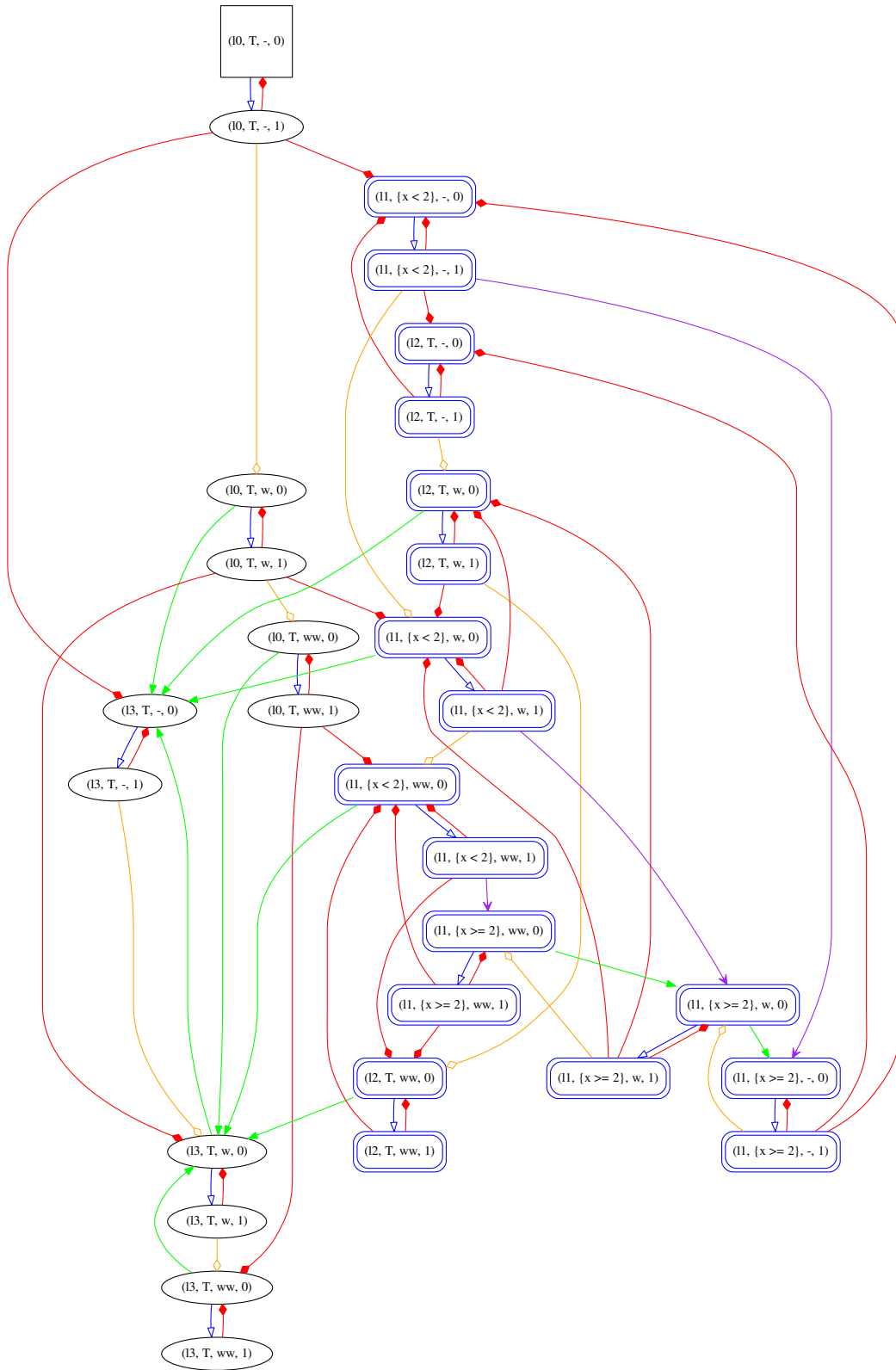
Figure 4.14 – Graphe de jeu associé à la propriété \varphi_5
