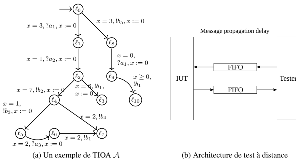
Figure 2.14 – Test à distance dans un cadre temporisé
