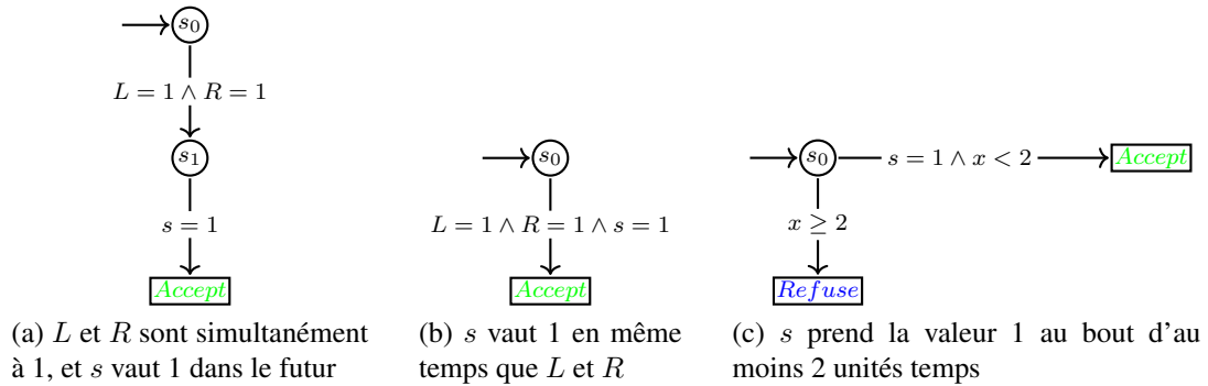
Figure 2.11 – Exemples d'objectifs de test
