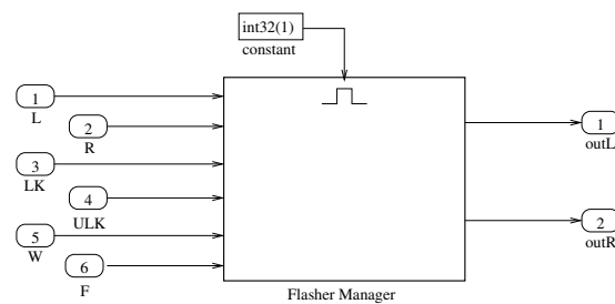
Figure 3.3 – Modèle Simulink simplifié du FlashManager
