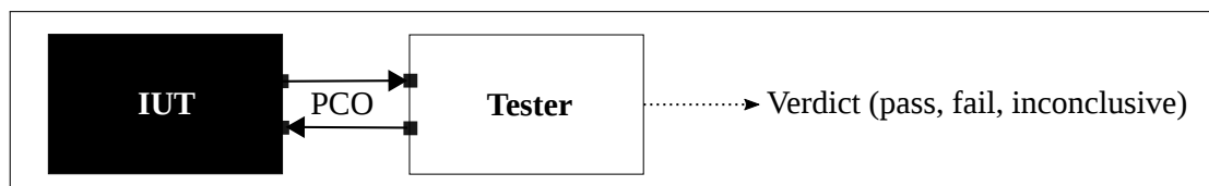
Figure 2.2 – Principe du test boîte noire
