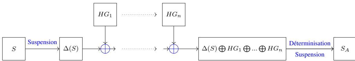
Figure 2.4 – Construction de la spécification augmentée
