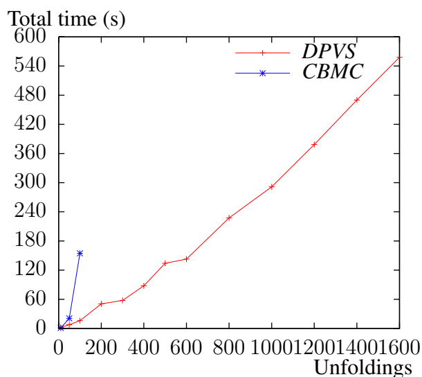
Figure 3.6 – Temps total nécessaire (en secondes) pour vérifier la propriété 4 en fonction du nombre de dépliages
