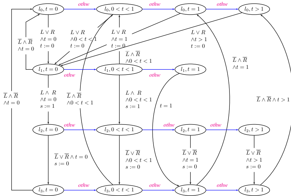
Figure 2.13 – Le TAG correspondant au VDTA de la figure 2.9
