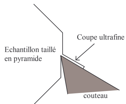
Figure II- 6 : principe de l'ultramicrotomie.
