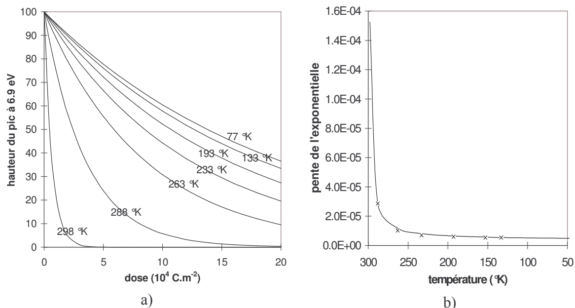
Figure IV- 7 : a) évolution de la hauteur du pic \pi \rightarrow \pi^* du PS à 6.9 eV en fonction de la température de l'échantillon. Les valeurs expérimentales ont été ajustées en première approximation par une exponentielle décroissante. b) évolution de la pente de l'exponentielle en fonction de la température de l'échantillon. Microscope Philips EM420/PEELS. Taille de sonde : 100 nm. Dispersion en énergie 0.1 eV/canal.
