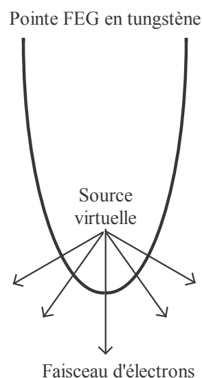
Figure V- 1 : extraction des électrons d'une pointe FEG perpendiculairement à la courbure de la pointe. Les électrons semblent émis d'une source virtuelle quasi-ponctuelle.
