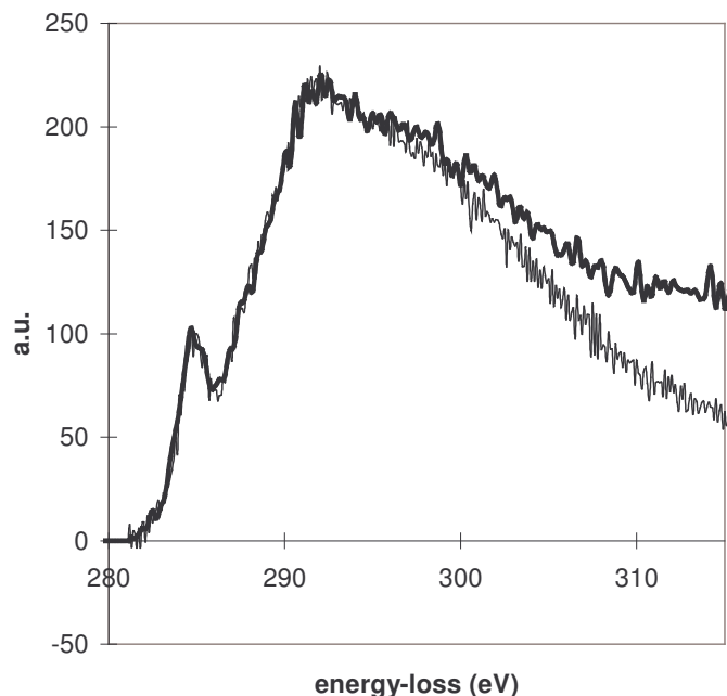
Figure IV- 10 : seuils K du carbone pour le PB haut-cis (trait gras) et le PB bas-cis (trait fin), pour une dose de 1.6 \cdot 10^4 \text{ C.m}^{-2} . La comparaison des spectres à dose identique montre que la dégradation ne permet pas de différencier les isomères du PB. Microscope Philips EM420. Taille de sonde : 100 nm ; dispersion en énergie : 0.1 eV / canal. Température : -180 \text{ }^\circ\text{C} .
