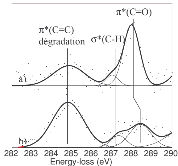
Figure V- 2 : seuils K du carbone du PMMA avec : a) le microscope JEOL 2010F. Taille de sonde : 2.4 nm. Température : -180 °C. Dose estimée : 10^7 C.m -2 . b) le microscope Philips EM420. Taille de sonde : 100 nm. Température : -180 °C. Dose estimée : 500 C.m -2 . Noter que la dégradation est moindre en mode nano-analyse.
