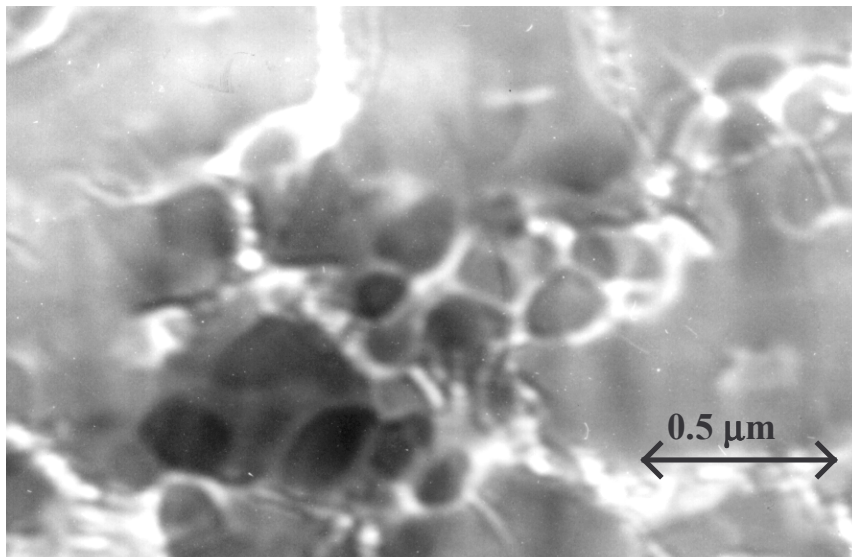
Figure IV- 4 : photo CTEM d'un échantillon de PS choc dans lequel les fissures se sont propagées le long des interfaces. Les fissures ont été provoquées par l'accumulation de charges électrostatiques à la surface du film et peuvent être évitées soit en plaçant un film de carbone à trous assurant un maintien mécanique et l'évacuation des charges, soit en plaçant un diaphragme objectif.
