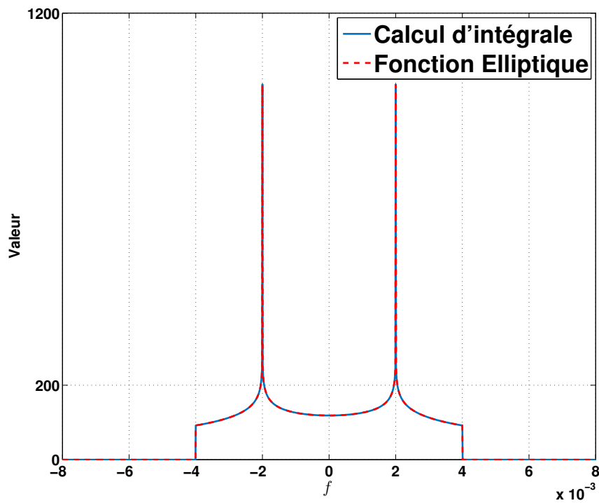
FIGURE I.4 – DSP de GC pour f_1T = 10^{-3} et f_2T = 3 \times 10^{-3} .
