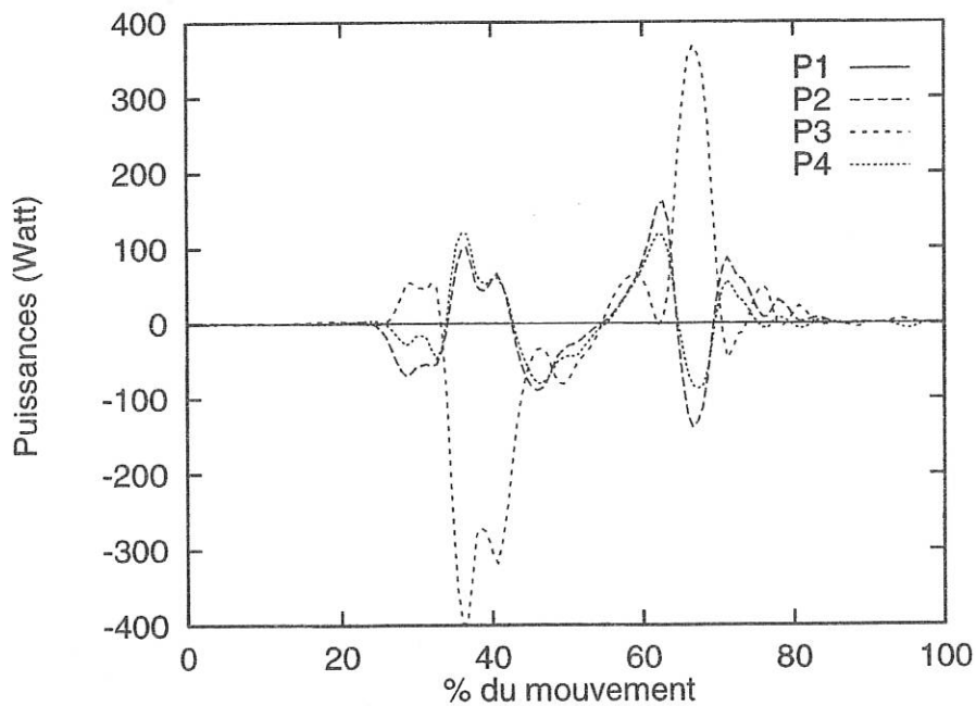
FIGURE III.4- Evolution des puissances articulaires P_i au cours du mouvement de flexion-extension
