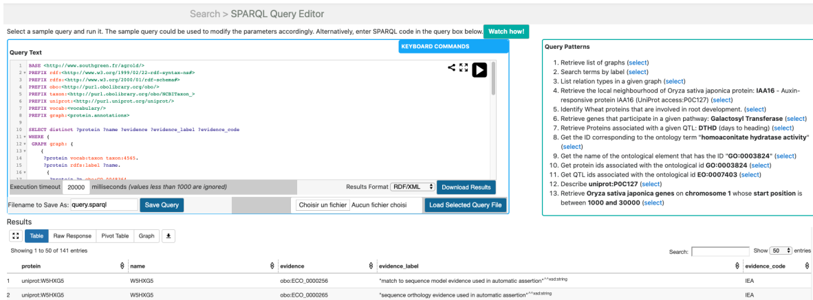
FIGURE 4.6 – Résultat de SPARQLEditor
