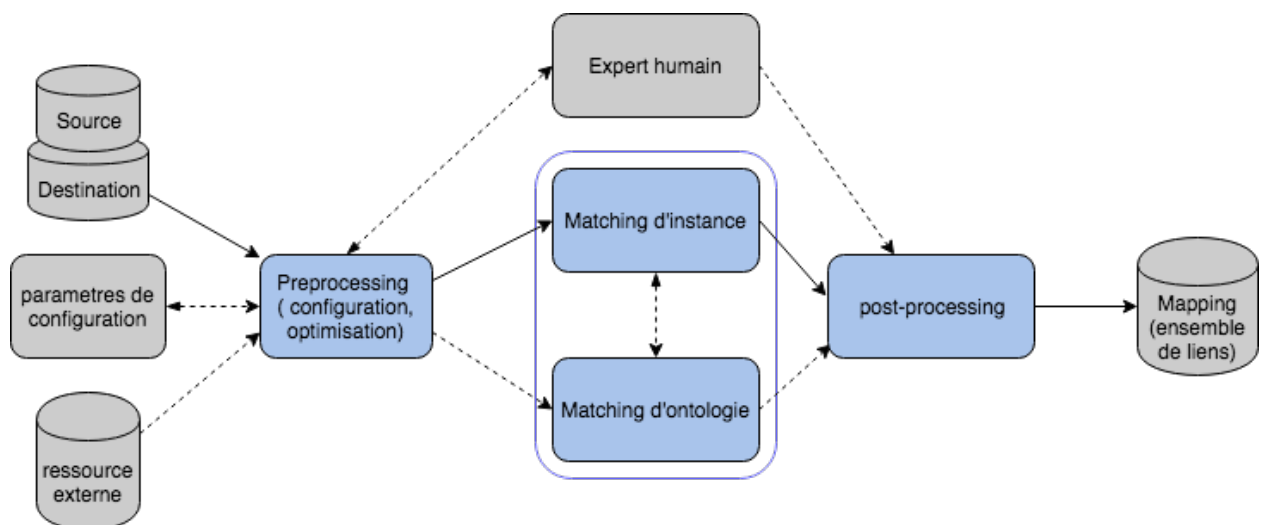
FIGURE 5.3 – Workflow général du processus de liage de données adapté de Achichi et al, 2018 [106]
