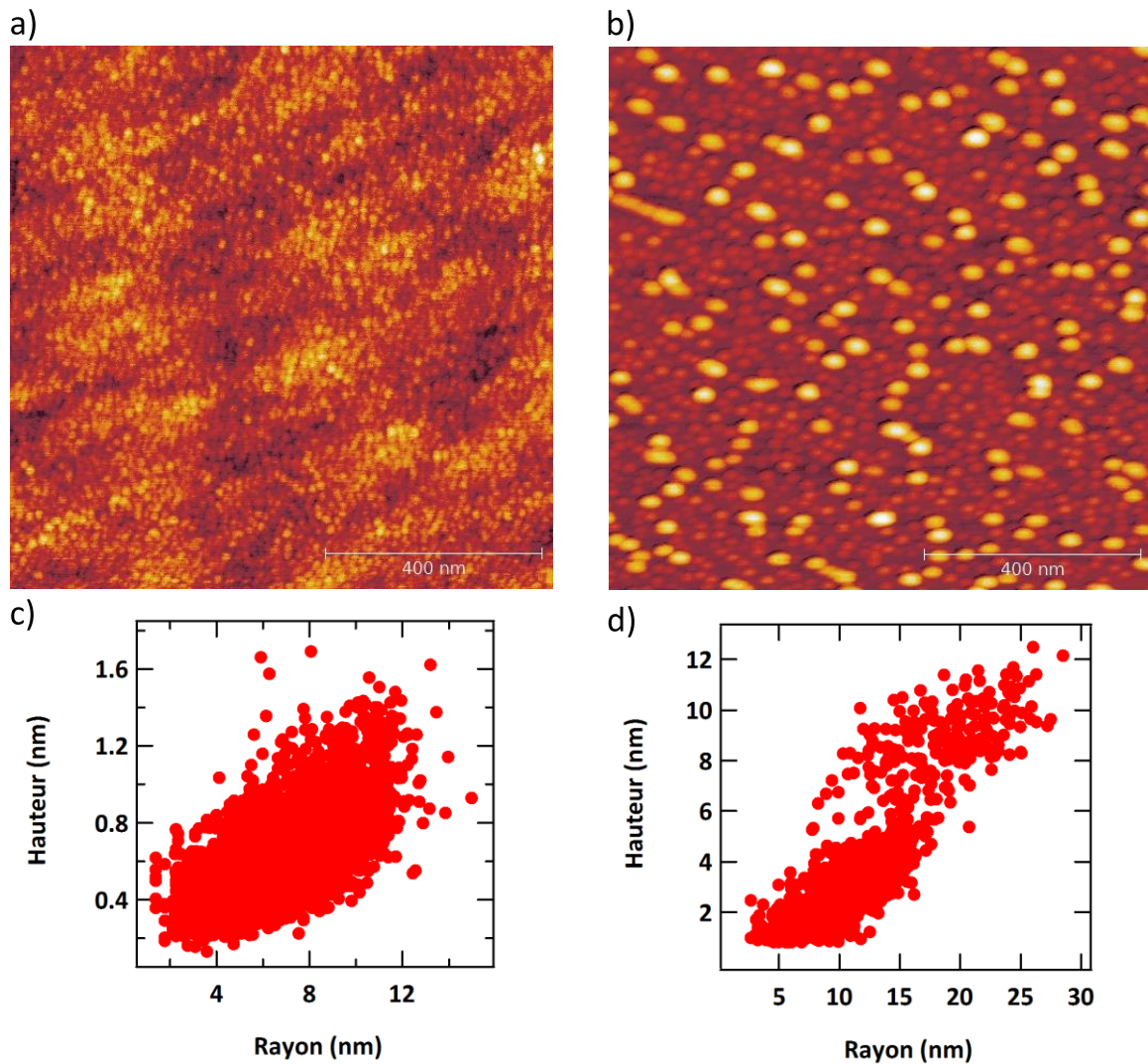
Fig. 3.14 Images AFM 1 \times 1 \mu\text{m}^2 et diagrammes hauteurs/rayons extraits pour les échantillons de QDs (In,Ga)As/GaP avec a) et c) 10% d'In (S1883) et b) et d) 35% d'In (S1826) réalisés à 500 \text{ }^\circ\text{C} .
