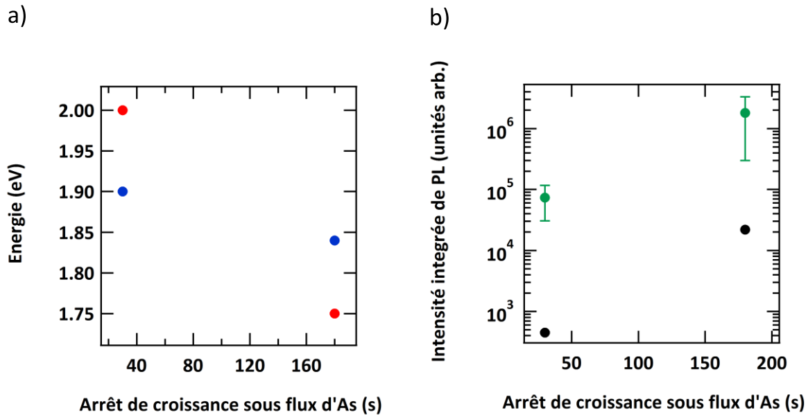
Fig. 3.34 a) Evolution de l'énergie à 10 K des transitions X_{xy}(\text{In,Ga})\text{As} (en rouge) et X_{z\text{GaP}} (en bleu) en fonction de l'arrêt de croissance sous flux d'As et b) intensité intégrée correspondante à 10 K (en vert) et 300 K (en noir) pour des QDs (In,Ga)As/GaP contenant 30 % d'In réalisées à 550 °C. L'épaisseur d'(In ,Ga)As déposée est de 3 ML. Les échantillons correspondants sont S1562 (30 s) et S1631 (180 s).
