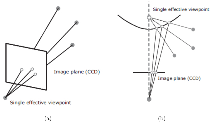
FIGURE 2.6 – Système vérifiant la condition de point de vue unique. (a) dans le cas d’une caméra perceptives. (b) dans le cas d’une caméra catadioptrique avec un miroir hyperbolique
