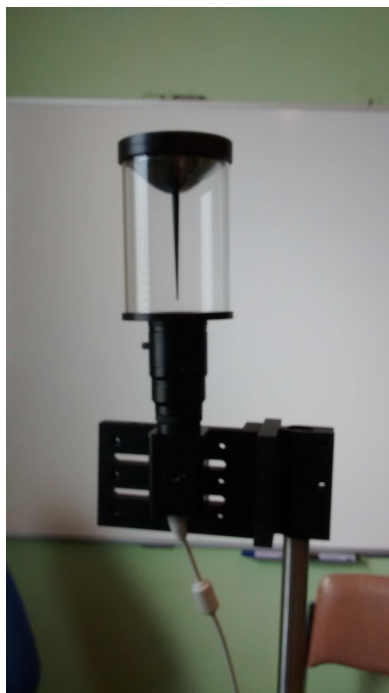
FIGURE 3.16 – La caméra catadioptrique avec un miroir hyperbolique de notre protocole expérimental.
