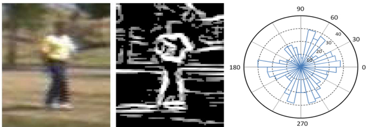
FIGURE 3.2 – Exemple des caractéristiques EOH
