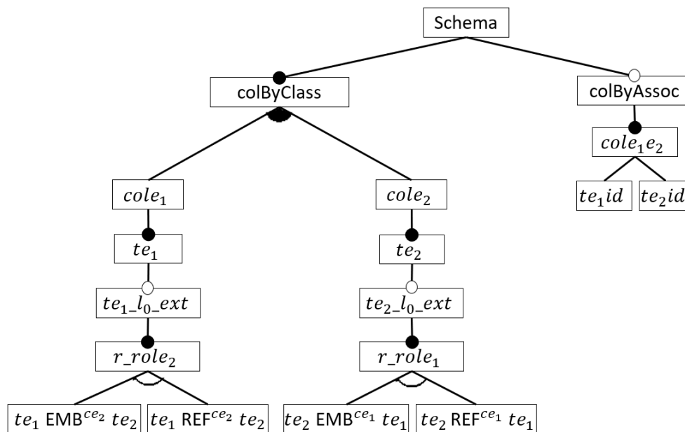
FIGURE 6.10: Modèle de caractéristiques d'une association UML
