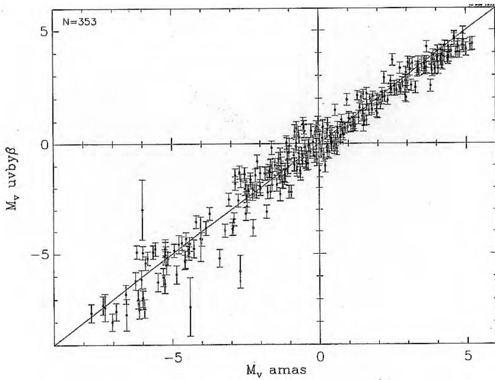
FIG. 2.2: Comparaison des magnitudes absolues obtenues par la photométrie uvby-β et par le module de distance d'amas
