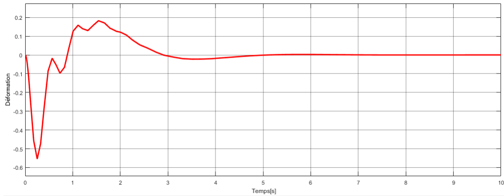
FIGURE 5.21 – Convergence de la déformation avec CSM
