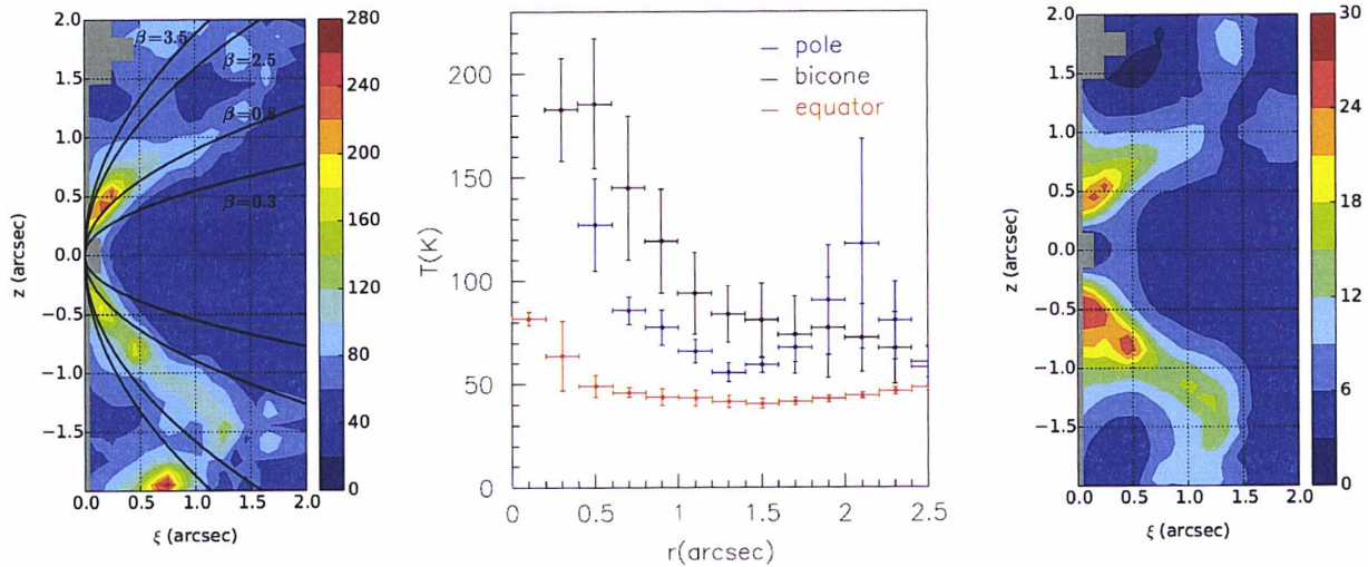
Figure 4: Rectangle Rouge. A gauche: carte des températures dans le demi-plan méridien de l'étoile, obtenu à partir de la densité effective. Au centre: distribution de la température du gaz, moyennée sur trois différents secteurs angulaires de latitude stellaire, en fonction de la distance r à l'étoile: les points rouges sont pour la région équatoriale, les points noirs sur le bicône à l'interface et les points bleus pour les régions polaires. Les barres d'erreur indiquent la dispersion dans chaque bin. A droite: densité du monoxyde de carbone (en molécules par \text{cm}^3 ) multipliée par r^2 (en \text{arcsec}^2 ).
