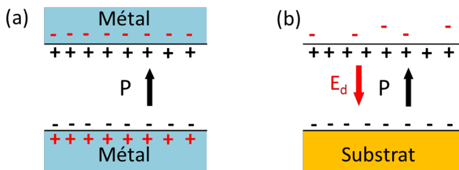
Figure I-20. Schéma d'un film ferroélectrique pour différentes conditions aux limites : (a) structure de type MIM ; les charges de polarisation sont parfaitement écrantées et (b) ferroélectrique déposé sur un substrat semi-conducteur ou isolant sans électrode supérieure ; l'écrantage incomplet des charges génère un champ dépolarisant E_d .
