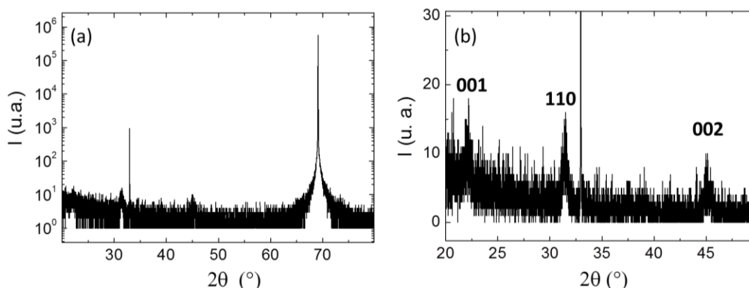
Figure VI-6. (a) Diagramme de diffraction des rayons X hors plan de l'échantillon #3 et (b) zoom sur la région entre 20 et 50°
