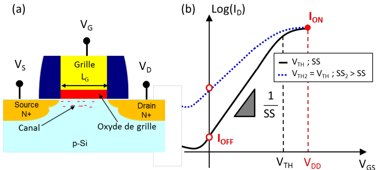
Figure I-14. (a) Représentation schématique d'un transistor n-MOSFET et (b) caractéristique de sortie I_D(V_{GS}) .
