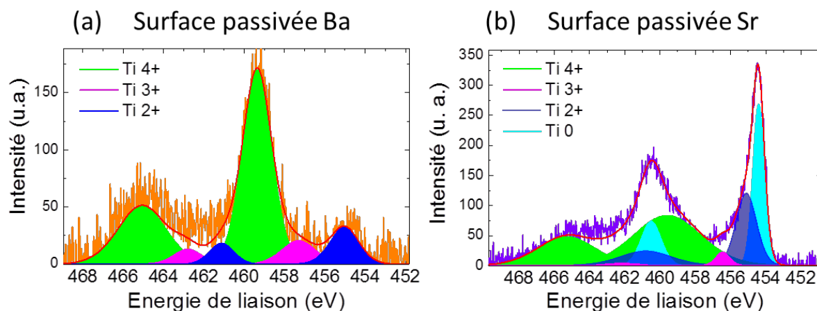
Figure V-30. Comparaison des spectres XPS Ti 2p des substrats Si 0,8 Ge 0,2 passivés avec du baryum (a) et du strontium (b) après la croissance de 2 monocouches de BaTiO 3 (étape 5).
