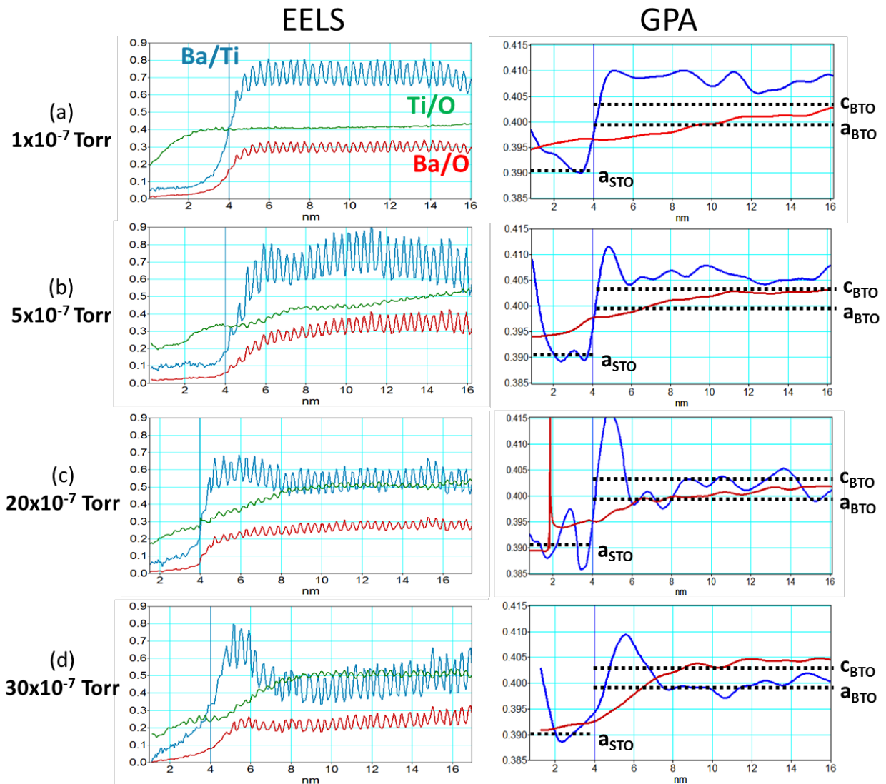
Figure III-21. Graphes de gauche : Profils des rapports de concentration élémentaires Ba/Ti (en bleu) Ti/O (en vert) et Ba/O (en rouge) extraits des mesures EELS pour les échantillons élaborés à différentes pressions d'oxygène. Graphes de droite : Profils des paramètres de mailles extraits des mesures GPA des mêmes échantillons.
