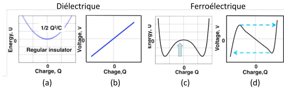
Figure I-17. (a) Profil d'énergie et (b) dérivée dU/dQ pour une capacité avec un matériau diélectrique classique. (c) Profil d'énergie dans une capacité ferroélectrique et (d) dérivée dU/dQ associée - Graphes extraits de la référence [30].
