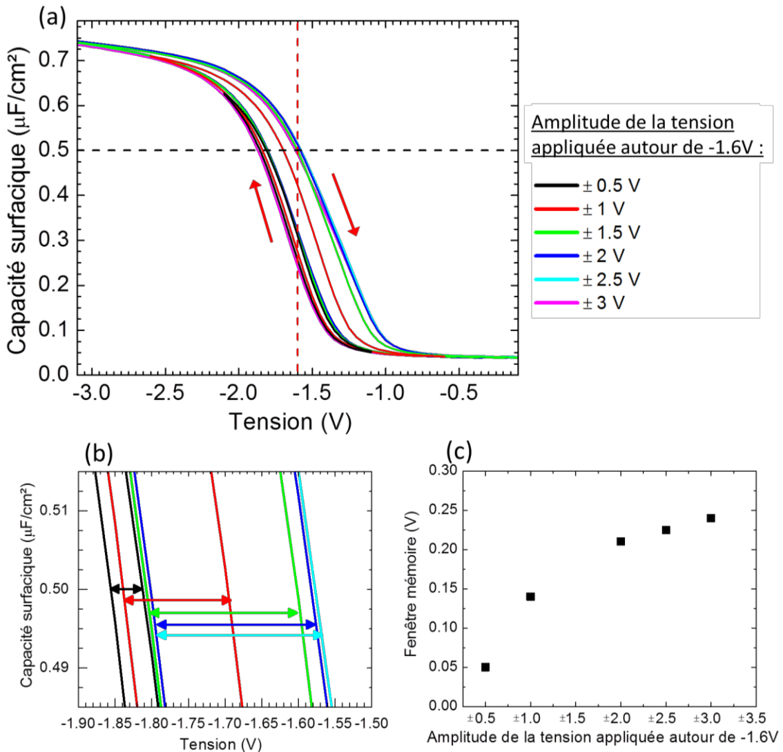
Figure VI-13. (a) Caractéristiques C-V d'une capacité \text{TiN}/\sim 11\text{ nm BaTiO}_3/\sim 2\text{ nm SrTiO}_3/\text{SiO}_2/\text{Si}(001) de taille 75 \times 75\text{ }\mu\text{m}^2 en fonction de la tension appliquée (b) Zoom des courbes C-V (c) Fenêtre mémoire extraite à 0.45\text{ }\mu\text{F}/\text{cm}^2 en fonction de la tension appliquée.
