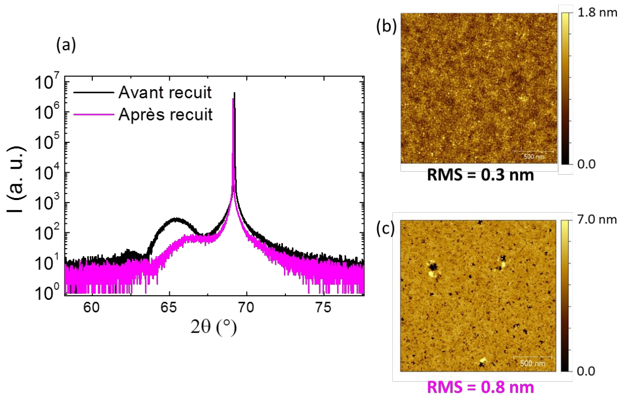
Figure V-6. (a) Diagrammes de diffraction des rayons X hors plan du substrat de SiGe W75-30s avant et après recuit ; (b-c) Images AFM 2 \times 2 \mu\text{m}^2 de la couche (b) avant recuit et (c) après recuit à 760°C pendant 20 minutes.
