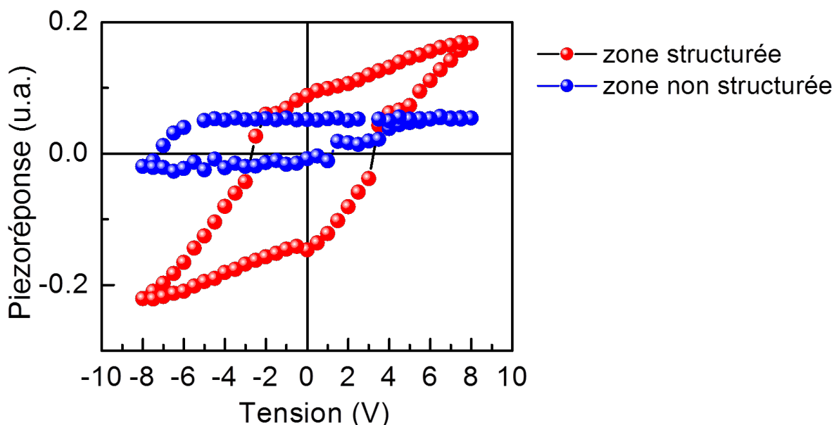
Figure VI-23. Comparaison des cycles d'hystérésis piézoréponse rémanents mesurés par PFM dans une zone structurée (courbe bleue) et une zone non structurée (courbe rouge) de l'échantillon #6 (11 nm BaTiO 3 /~2 nm SrTiO 3 /SiO 2 /Si) sans électrode de TiN.
