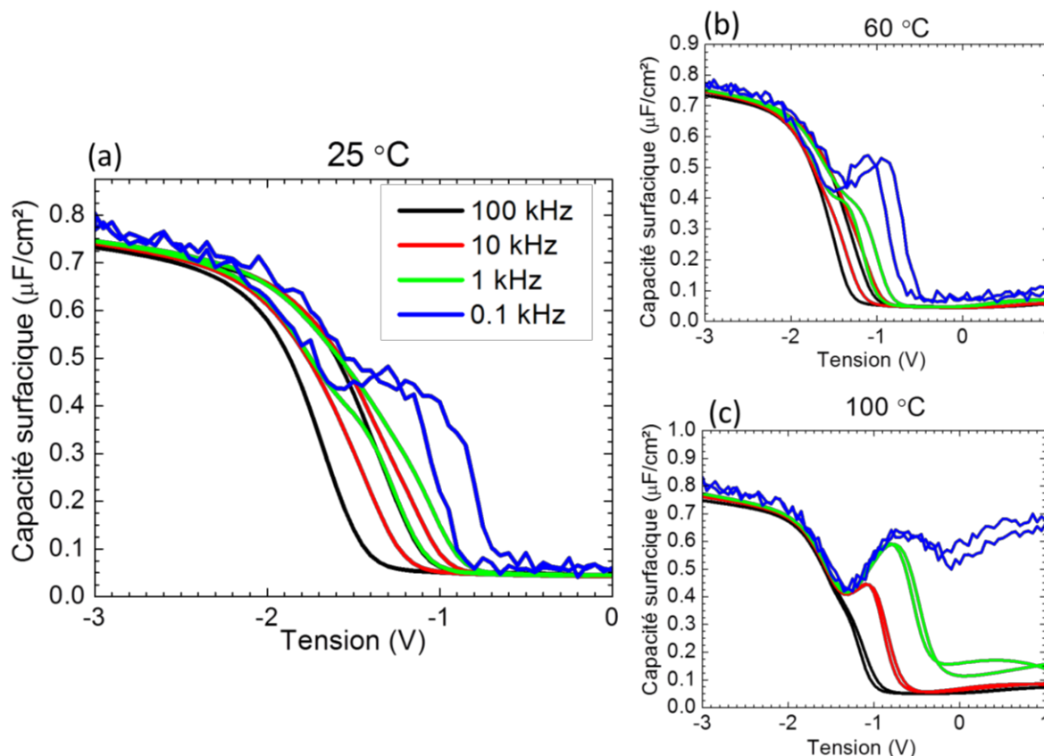
Figure VI-19. Caractéristiques C-V mesurées sur une capacité \text{TiN}/\sim 11\text{ nm BaTiO}_3/\sim 2\text{ nm SrTiO}_3/\text{SiO}_2/\text{Si}(001) de taille 75 \times 75\ \mu\text{m}^2 en fonction de la fréquence (a) à 25^\circ\text{C} (b) à 60^\circ\text{C} (c) à 100^\circ\text{C} .
