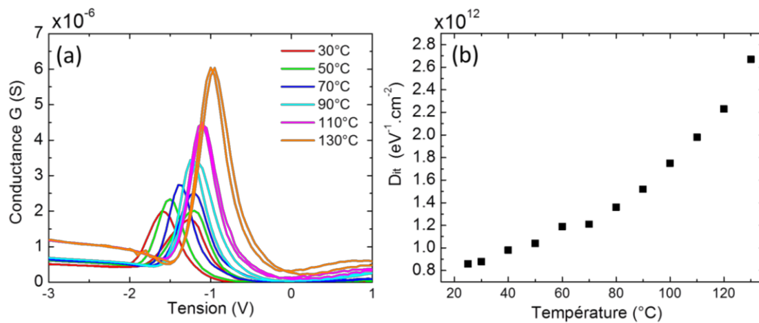
Figure VI-18. (a) Courbes de conductance mesurées sur une capacité TiN/\sim 11 nm BaTiO_3/\sim 2 nm SrTiO_3/SiO_2/Si(001) de taille 75 \times 75 \mu m^2 en fonction de la tension, pour différentes températures (b) Evolution de la densité d'états d'interface D_{it} en fonction de la température.
