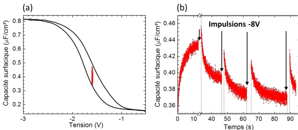
Figure VI-21. (a) Caractéristique C-V mesurée sur une capacité \text{TiN}/\sim 11 \text{ nm BaTiO}_3/\sim 2 \text{ nm SrTiO}_3/\text{SiO}_2/\text{Si}(001) de taille 20 \times 20 \mu\text{m}^2 (b) mesure de la capacité en fonction du temps après l'application d'impulsions de tension de -8V pendant 0.2 ms.
