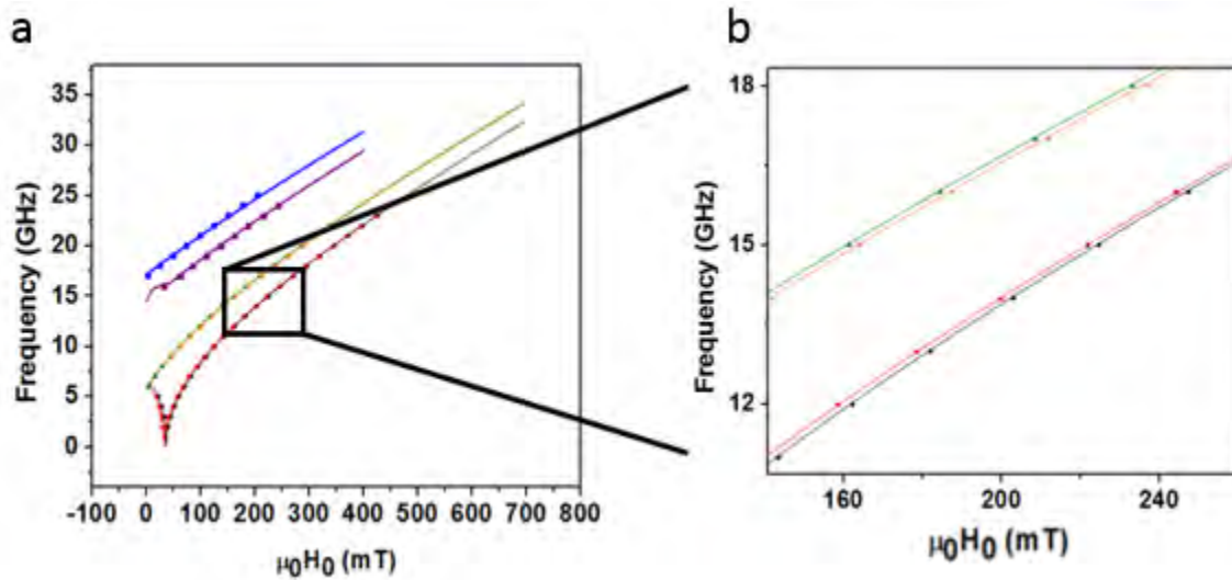
Figure 14: a) relation de dispersion F_{res} vs. \mu_0 H_0 pour l'échantillon de référence pour un champ appliqué dans le plan de la couche. A droite, zoom sur les deux modes délimitées par la boîte noire en a).
