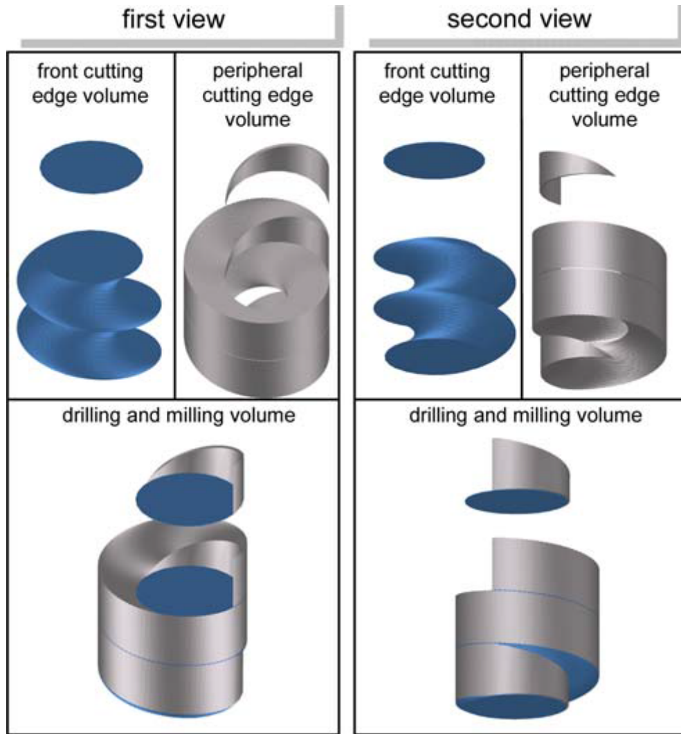
FIGURE 1.49 – Volumes des différents enlèvements de matière en perçage orbital [Brinksmeier et al., 2008]
