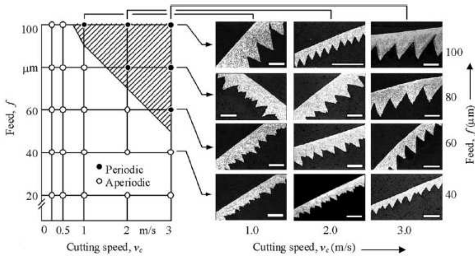
FIGURE 1.4 – Morphologie du copeau du Ti6Al4V en fonction de la vitesse de coupe et de l'avance en coupe orthogonale (échelles de 100 \mu\text{m} ) [Barry et al., 2001]
