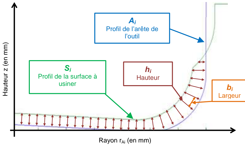
FIGURE 2.15 – Discretisation de la section de copeau pour un angle \varphi_i donné
