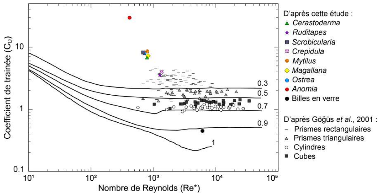
Figure II.12. Coefficient de traînée C_D en fonction du nombre de Reynolds de grain ( Re^* ). Les courbes noires représentent les facteurs de formes obtenus par Alger et Simons (1968) sur des particules de type graviers. Les valeurs pour différentes formes géométriques obtenues par Gögüs et al. (2001) ont également été ajoutées.
