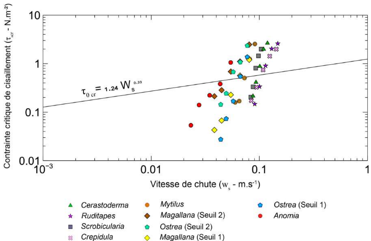
Figure II.33. Contraite critique de cisaillement en fonction de la vitesse de chute des particules bioclastiques. La relation empirique obtenue par Collins et Rigler (1982) est reportée sur le graphique (ligne noire).
