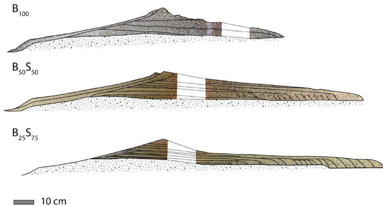
Figure III.46. Comparaison de l'architecture interne des modèles B_{100} , B_{50} S_{50} et B_{25} S_{75} sans le cas des stades 1 et 3. Les barrières sont centrées par rapport à leur crête la plus élevée.
