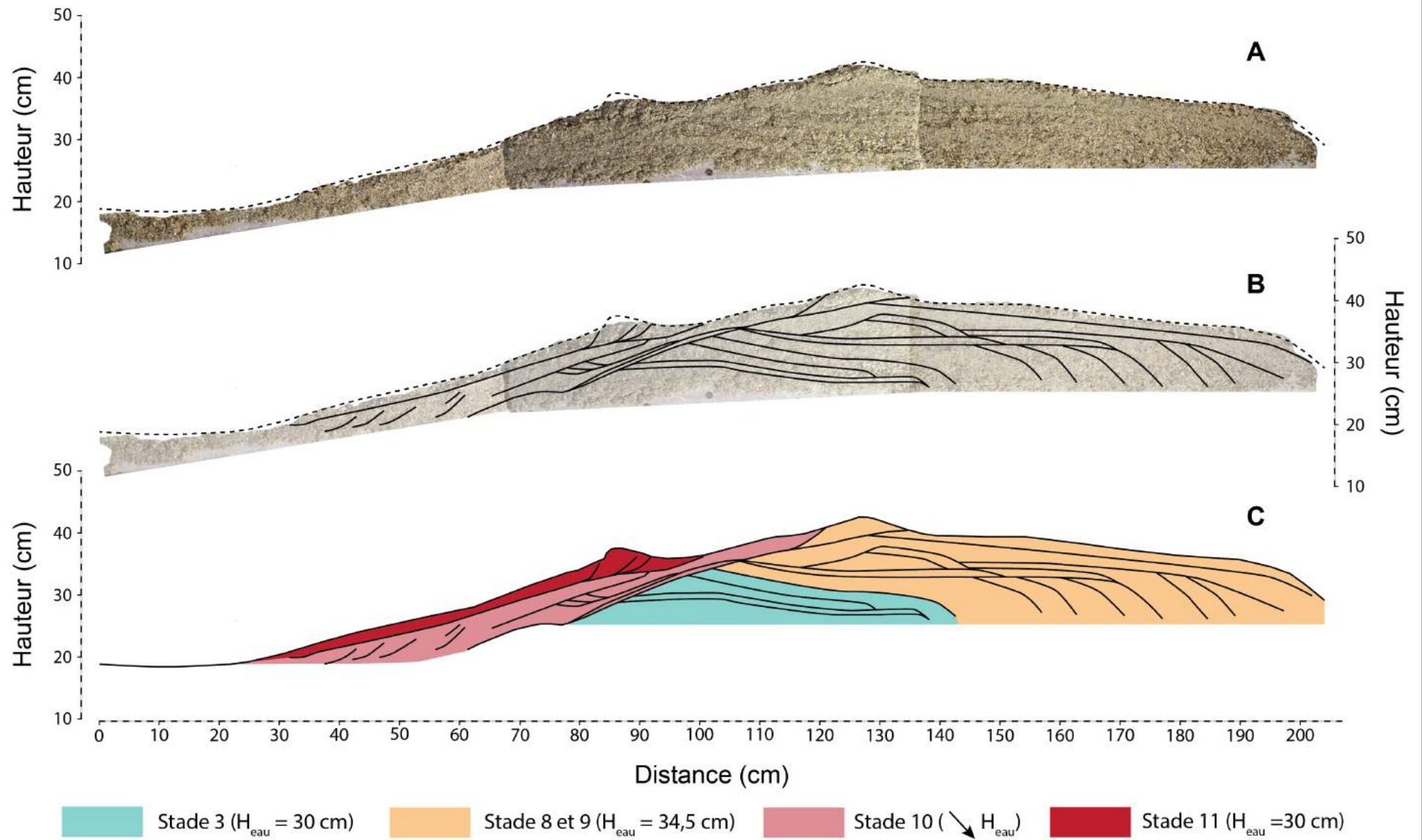
Figure III.29. Architecture sédimentaire du stade final (stade 11) du modèle B_{100} : (A) Epoxy-peel, (B) interprétation. Version au format A3 dans le livret en annexe.
