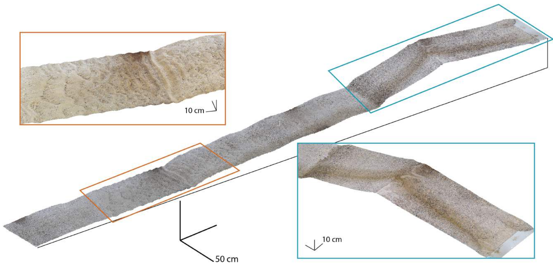
Figure III.32. Modèle photogrammétrique du stade 3 ( H_{eau} = 30 cm).
