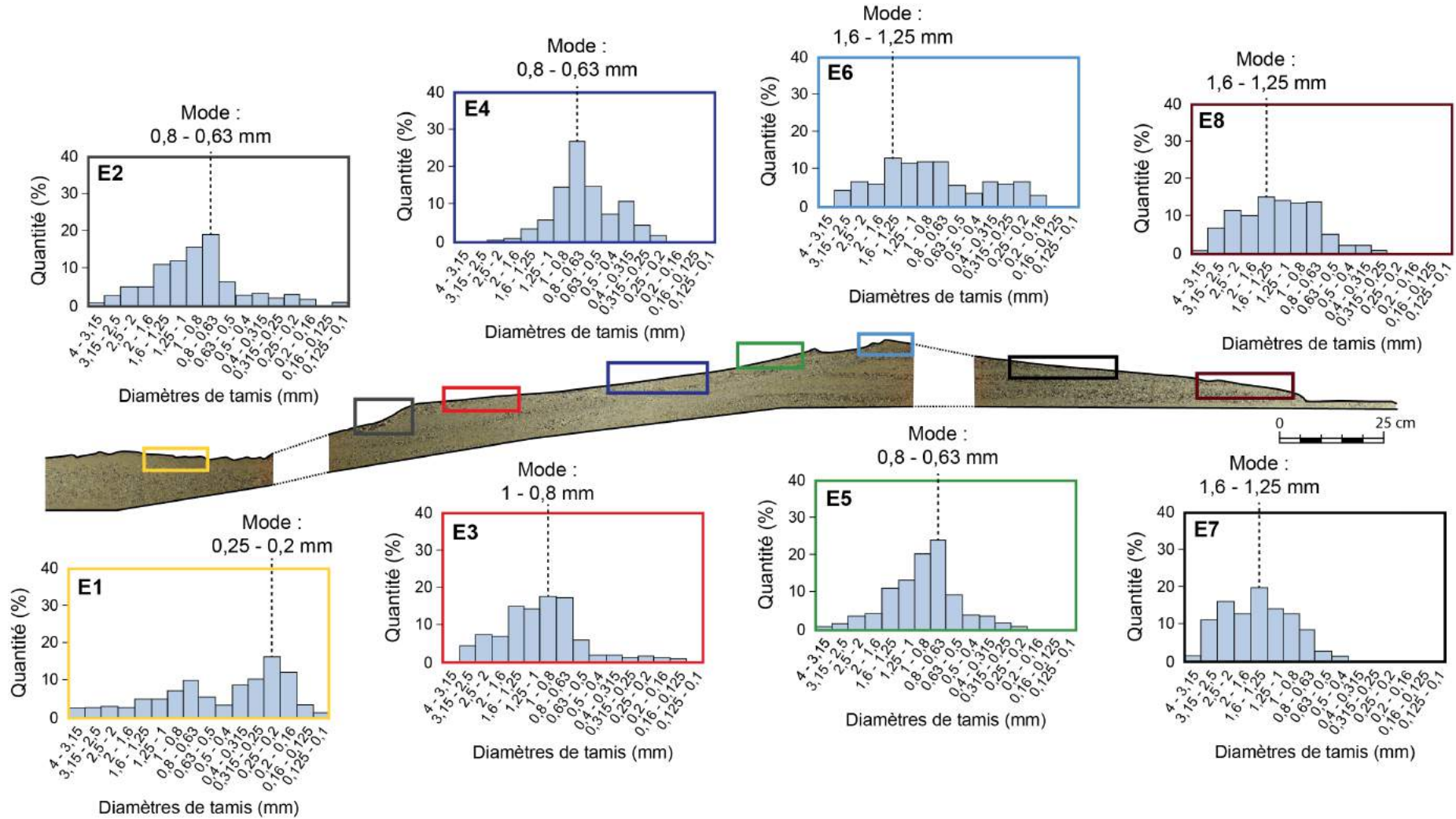
Figure III.36. Évolution de la granulométrie de surface le long de la barrière finale.
