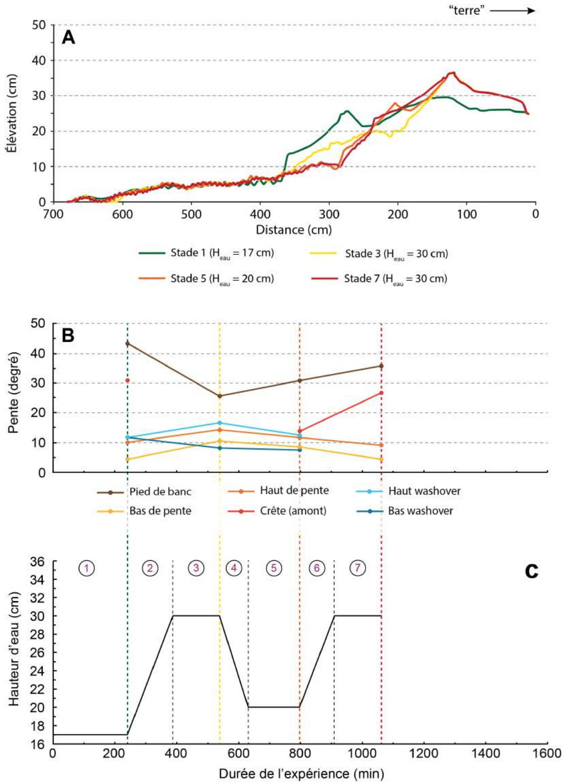
Figure III.37. Évolution du niveau d'eau moyen au cours du temps dans le cas du mélange B_{25}S_{75} . Les différentes étapes de montée, stabilisation et diminution de la hauteur sont délimitées et numérotées.
