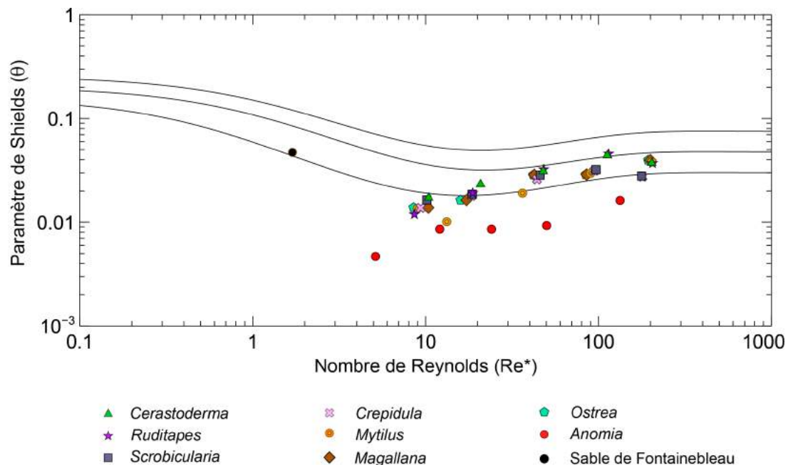
Figure II.34. Évolution du paramètre de Shields en fonction du nombre de Reynolds. Les courbes de Shields ont été redessinées à partir de Paphitis (2001). Seul le second seuil de mise en mouvement de Magallana et Ostrea a été tracé. Le sable quartzique (sable de Fontainebleau) a été utilisé pour valider les expériences.
