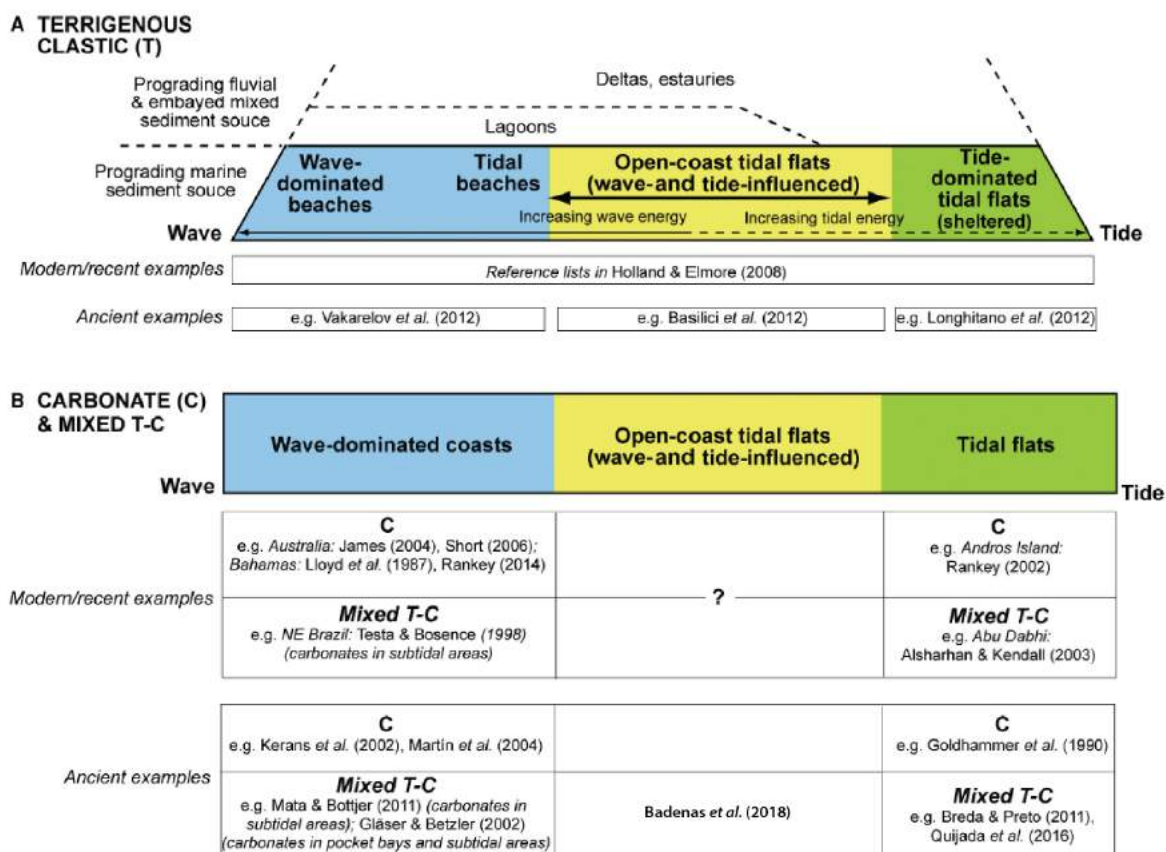
Figure I.4. Classification des différents littoraux en fonction du système binaire marée - houle, dans le cas des domaines sédimentaires mixtes silico-clastiques carbonatés. Figure modifiée d'après Bádenas et al. , 2018.
