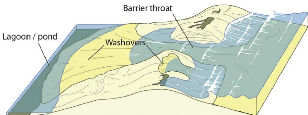
Figure III.1. Régime d'overwash en contexte transgressif : formation d'une brèche dans la barrière littorale et dépôt des sédiments sous forme de washover dans la lagune (d'après Goslin et Clemmensen (2017)).
