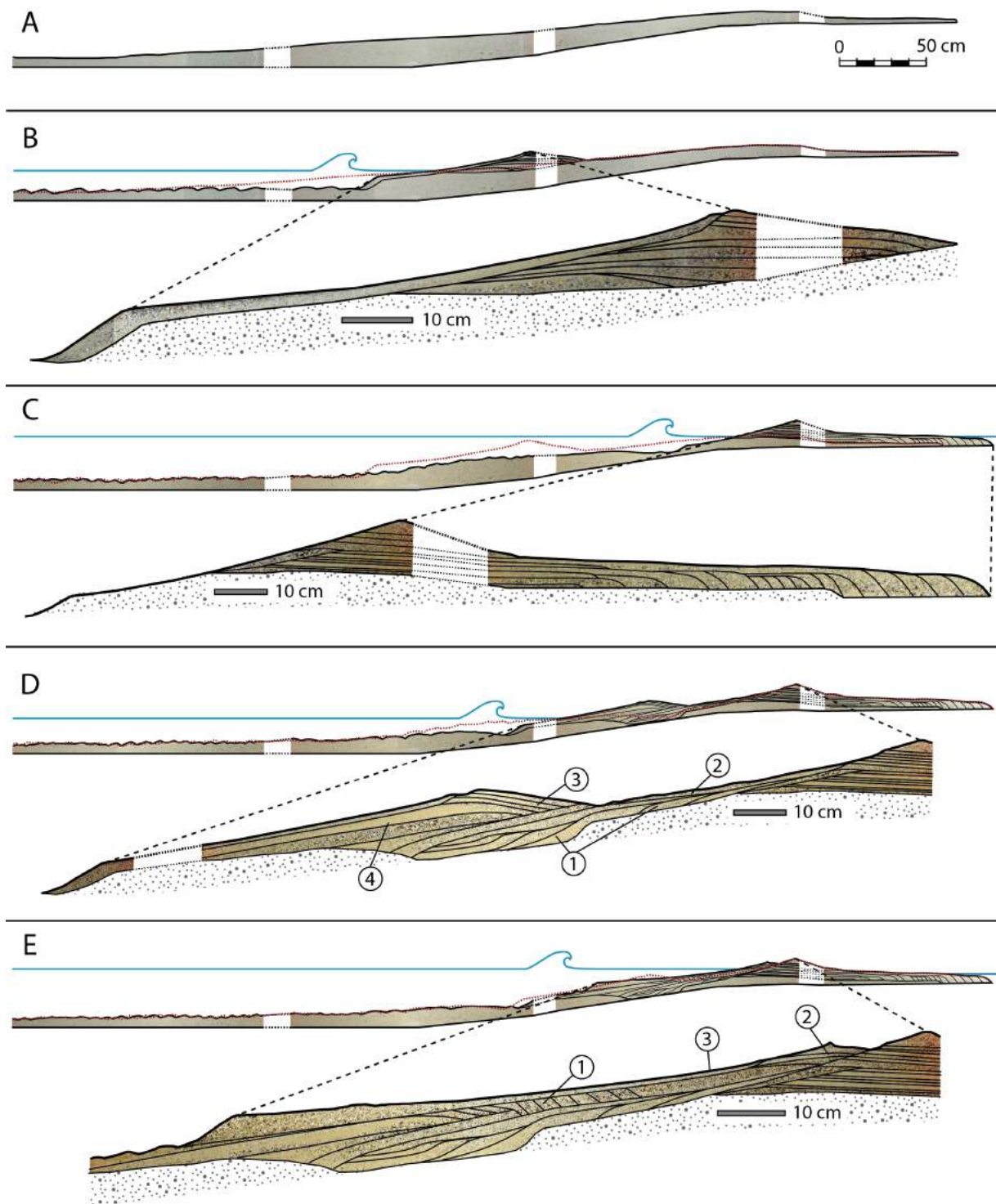
Figure III.42. Évolution de l'architecture interne de la barrière B 25 S 75 par suivi photographique le long des parois du canal. Pour chaque stade, un rappel de l'état d'équilibre du stade précédent est tracé (pointillés rouge). Version au format A3 dans le livret en annexe.
