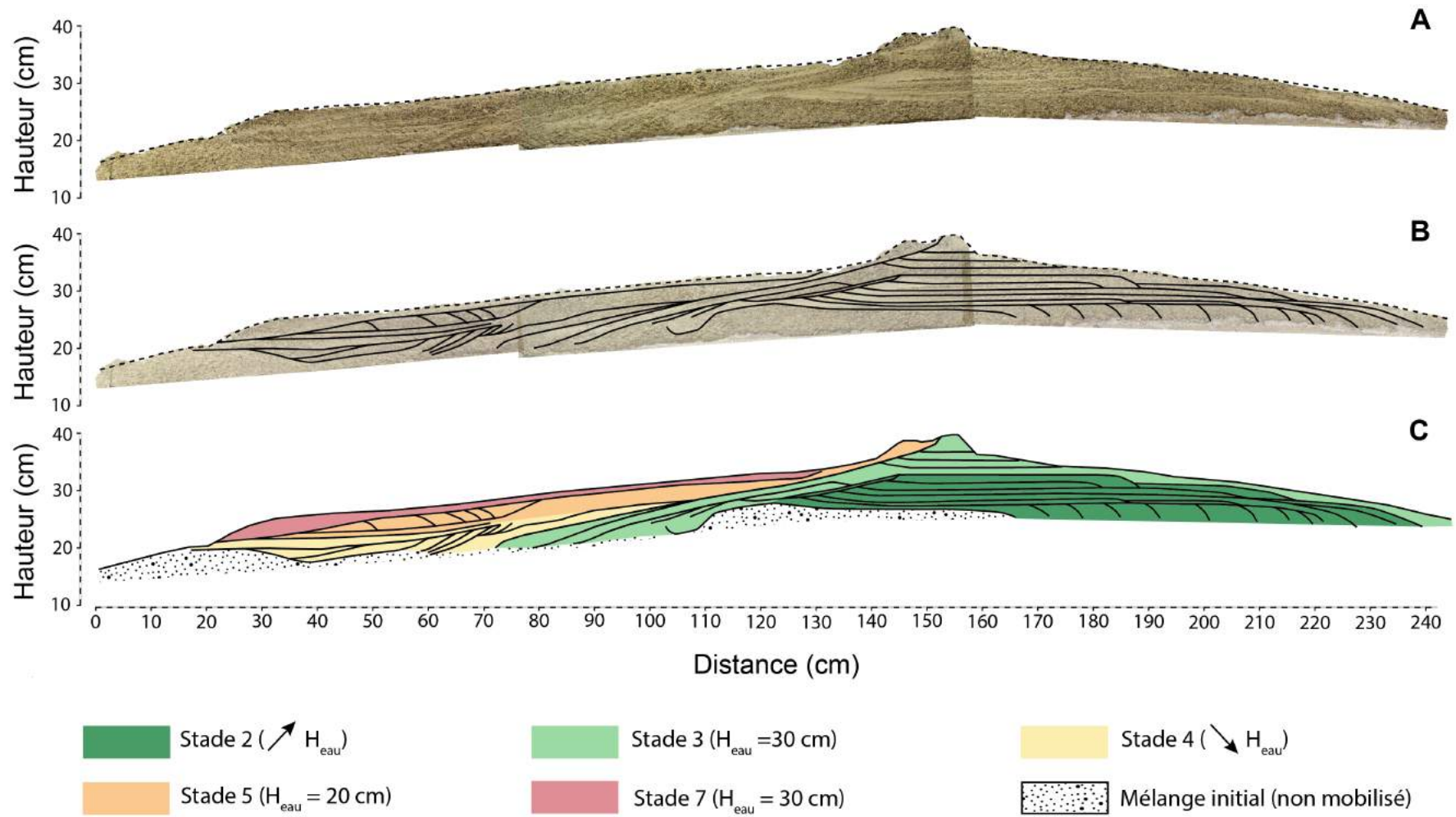
Figure III.35. Architecture sédimentaire du stade final (stade 7) du modèle B_{50} S_{50} : (A) Epoxy-peel, (B) interprétation. Version au format A3 dans le livret en annexe.
