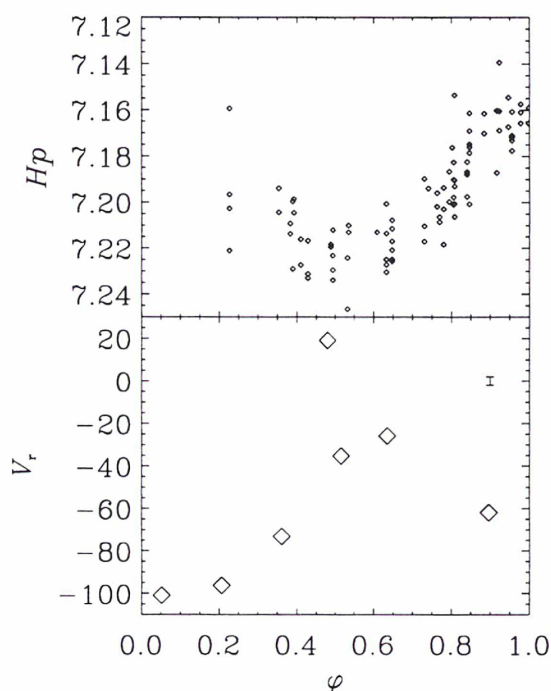
FIG. 3.19 - Courbe de lumière de HIP 37232 en magnitude H_p d'après les données Hipparcos et courbe de vitesse radiale repliée sur la période photométrique \varphi = 6^{\text{d}}.458 . La barre d'erreur des vitesses radiales est indiquée dans le panneau du bas
