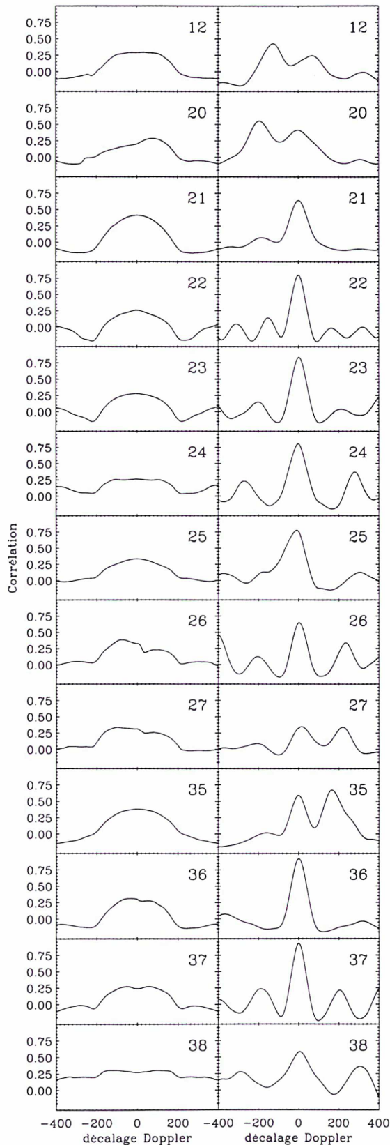
FIG. 3.11 - Corrélation séparée des ordres: la colonne de gauche représente la corrélation entre deux spectres synthétiques de T_{\text{eff}} = 10000 \text{ K} et de v \sin i 10 et 200 \text{ km s}^{-1} ; la colonne de droite représente la corrélation de deux spectres synthétiques de même v \sin i ( 25 \text{ km s}^{-1} ) et de température effective différente (10000 et 15000 K). On y remarque la variation de l'allure suivant le domaine spectral où est effectué la corrélation croisée (le chiffre dans le coin droit indique le numéro de l'ordre, cf. Table 3.2)
