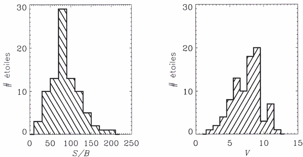
FIG. 3.1 - Distribution des rapports signal-sur-bruit S/B et des magnitudes apparentes visuelles V pour l'échantillon observé
