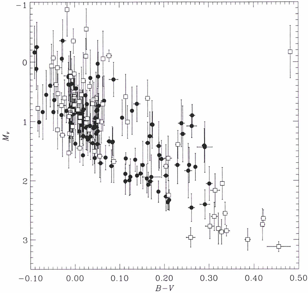
FIG. 2.6 - Diagramme H-R des étoiles non détectées binaires, de classe V, ayant une erreur relative \frac{\sigma_{\pi}}{\pi} < 0.1 . \square : v \sin i < 50 \text{ km s}^{-1} , \bullet : v \sin i > 200 \text{ km s}^{-1}
