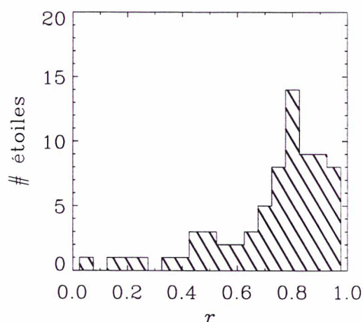
FIG. 3.14 - Distribution des coefficients de corrélation pour les étoiles observées figurant dans la table 3.9
