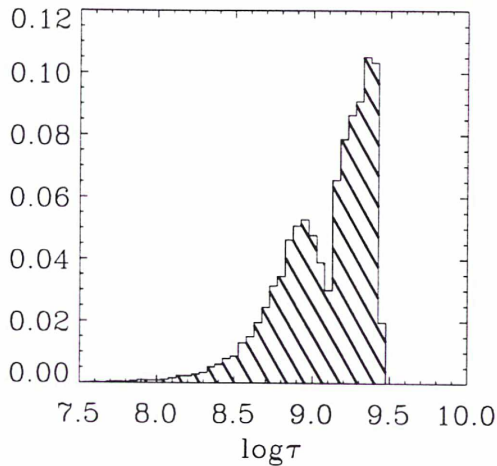
FIG. 5.4 - Distribution normalisée des âges des étoiles candidates évoluées sélectionnées suivant leurs âge, gravité et masse
