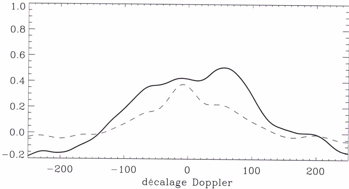
FIG. 3.18 - Pics de corrélation de HIP 37232 à la date julienne 50530.33280 avec un masque synthétique T_{\text{eff}} = 11000 \text{ K} , v \sin i = 5 \text{ km s}^{-1} . Le pic en train plein est obtenu après soustraction sur le spectre de HIP 37232 d'une composante de type G0 correspondant au pic principal du tracé en tirets
