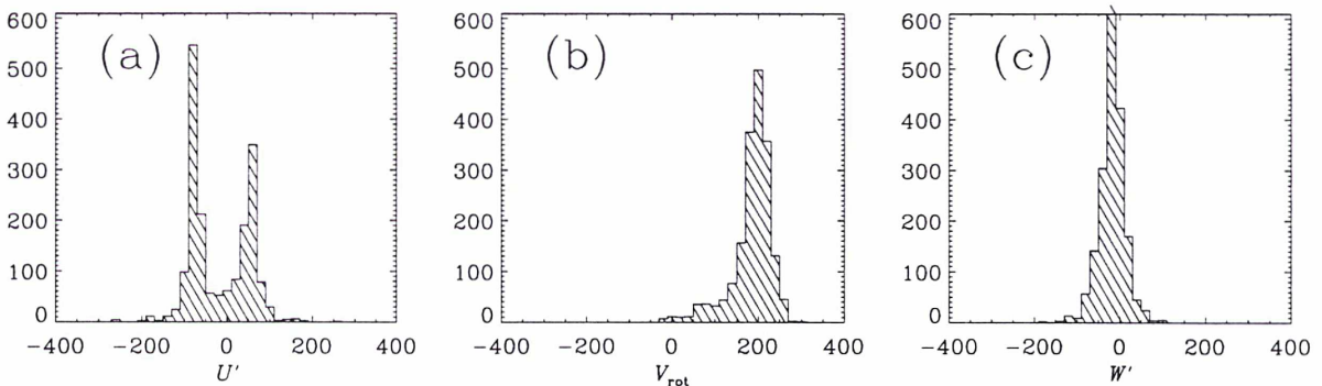
FIG. 5.9 - Échantillon d'étoiles à grande vitesse sélectionnées: (a,b,c) Distributions des vitesses spatiales U' , V_{\text{rot}} , W' pour les 1 827 étoiles
