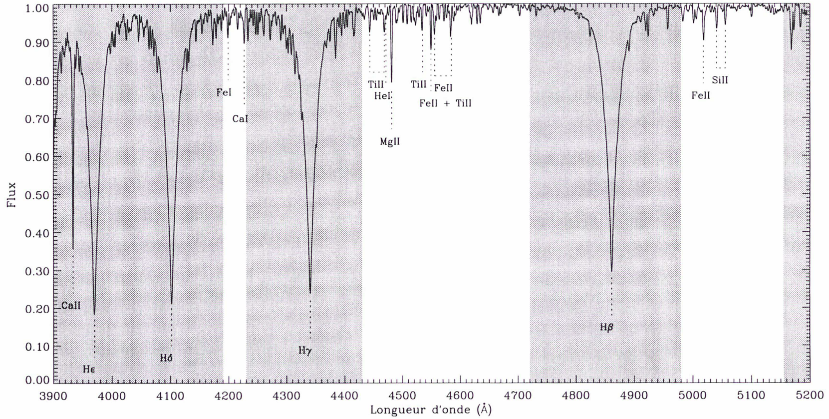
FIG. 3.3 - Domaine spectral utilisé (zones blanches) dans la corrélation (spectre calculé pour T_{\text{eff}} = 9200 \text{ K} et v \sin i = 100 \text{ km s}^{-1} )
