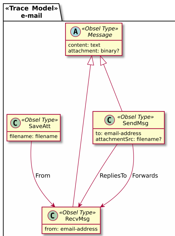
Fig. 2.1 An example trace-model (Champin, Mille, and Prié 2013).
