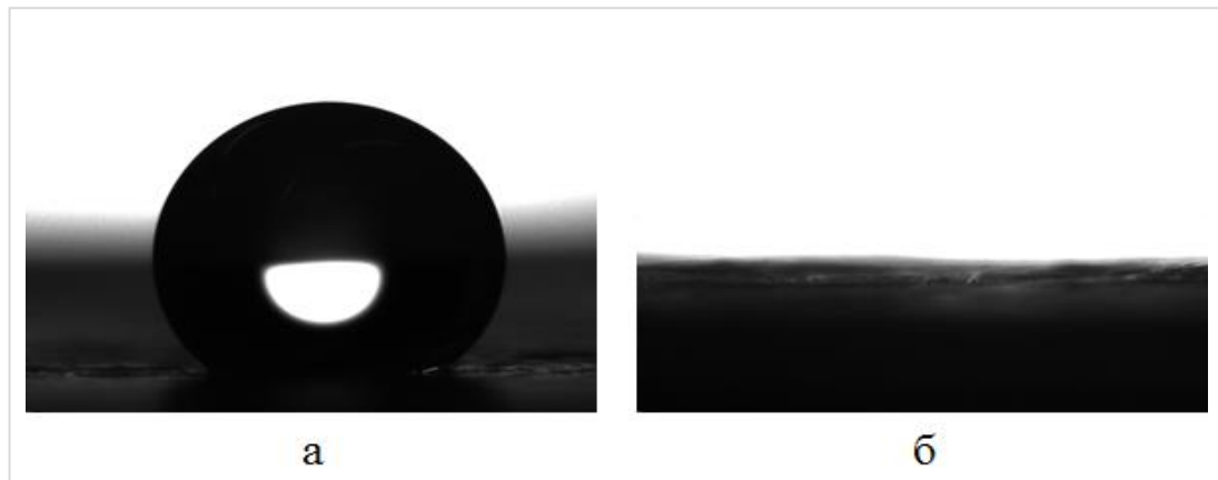
Рисунок 3.30 Визуализация краевого угла смачивания микроволоконистых каркасов на основе ПКЛ (а) без ПАВ и (б) с плуроником F-127. Световая микроскопия
