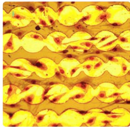
Дно каждой лунки планшета iCELLigence на 80% занимает золотой электрод (биосенсор)
