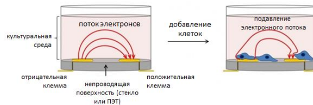
Рисунок 2.10 Принципиальная схема цитометрии в режиме реального времени на основе измерения электрического импеданса
