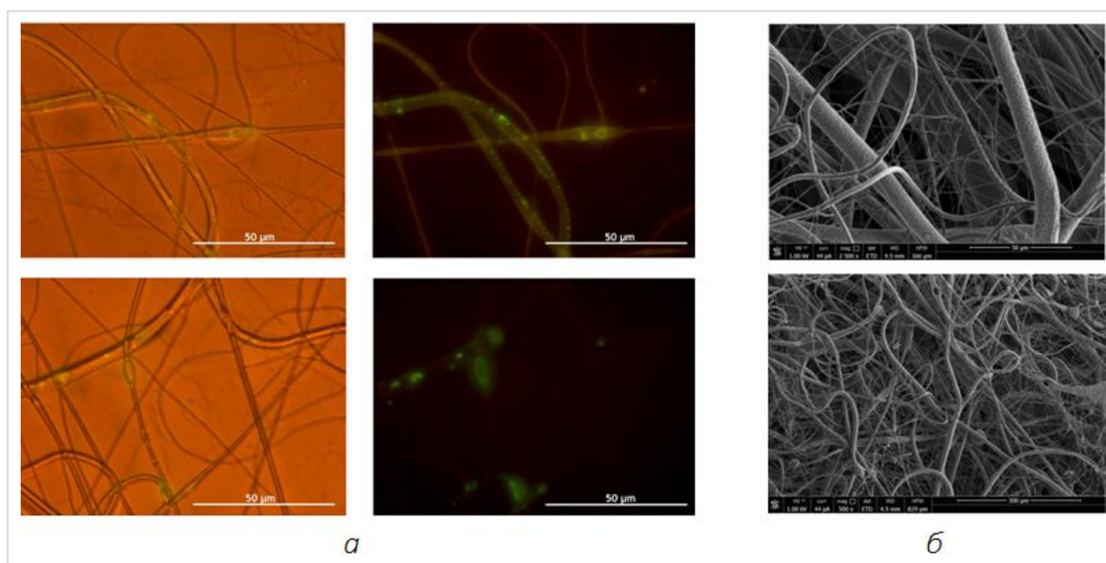
Рисунок 3.29 Микрофотографии: (а) волокна ПКЛ, содержащие флуоресцентную метку GFP; (б) морфология поверхности образцов волокнистого ПКЛ ( d_{\text{ср}}=2,1 мкм)
