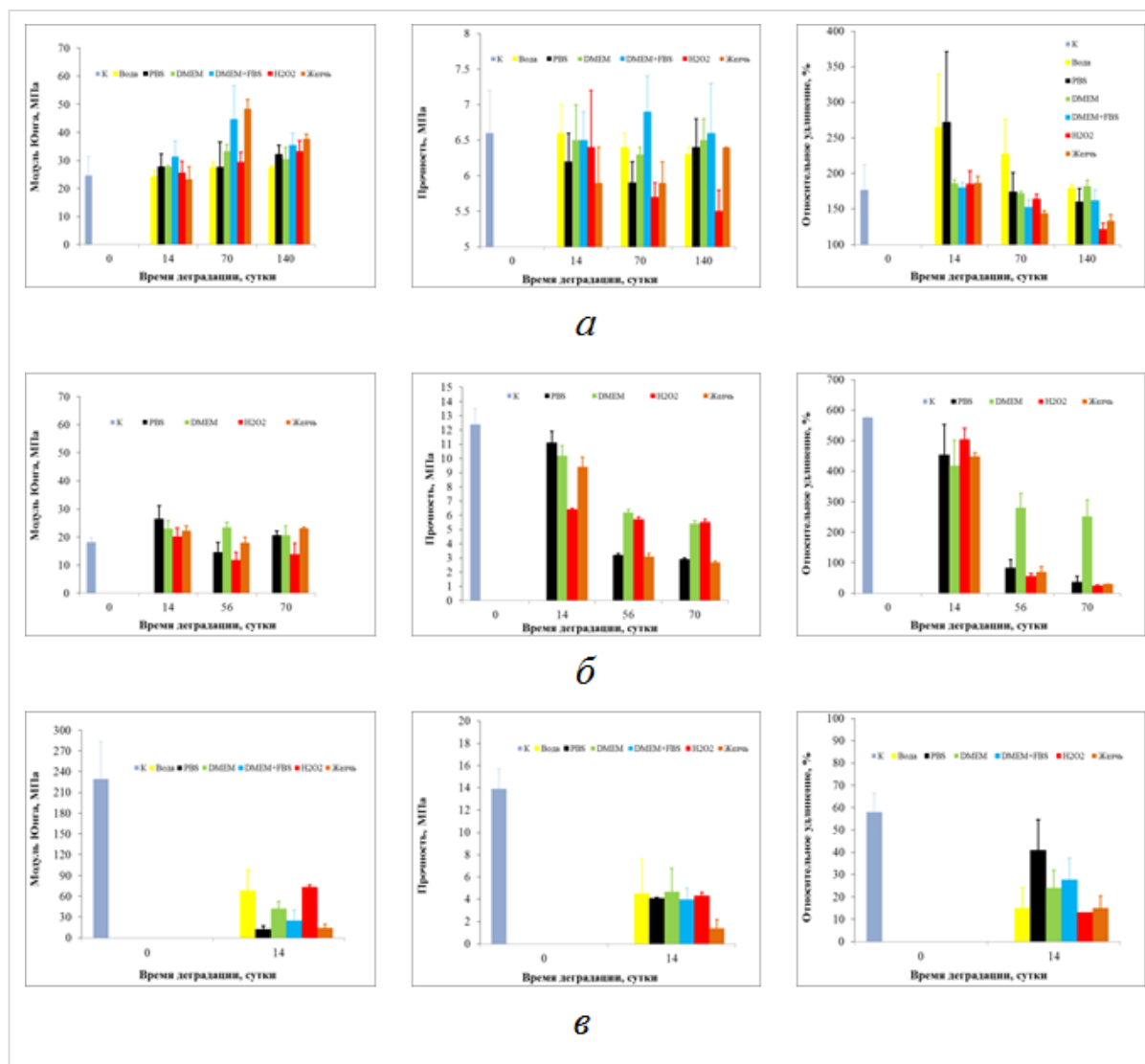
Рисунок 3.26 Зависимость изменения от условий деградации модуля упругости, прочности и разрывной деформации биосовместимых каркасов на основе: а – ПКЛ; б – PLCL; в – ПДЛГА. Контроль (К) – механические свойства исходных образцов
