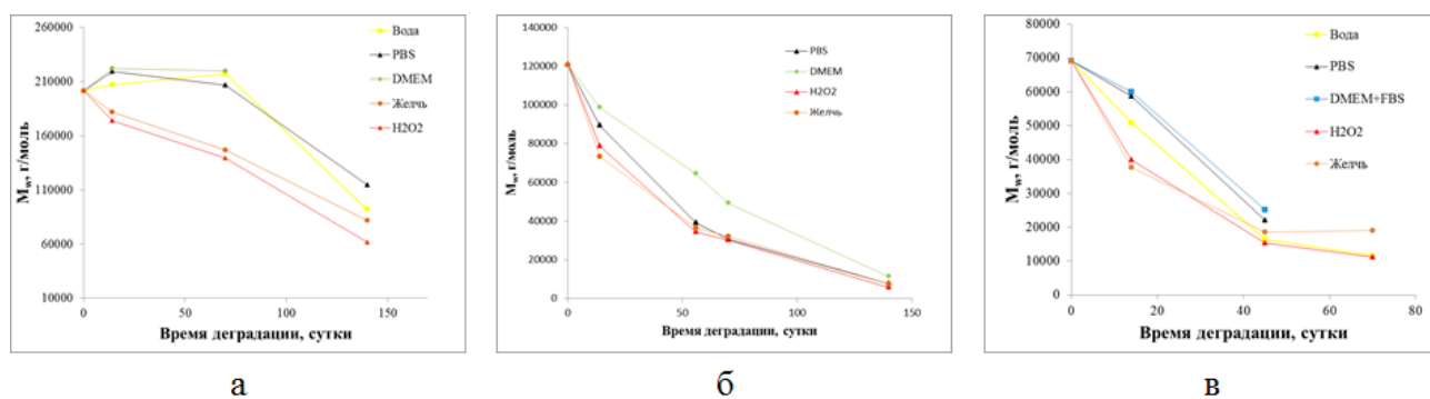
Рисунок 3.25 Изменение молекулярной массы материала каркасов на основе: а – ПКЛ; б – PLCL; в – ПДЛГА
