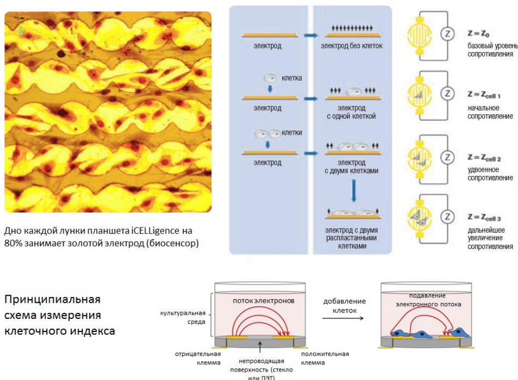
Рисунок 2.10 Принципиальная схема цитометрии в режиме реального времени на основе измерения электрического импеданса
