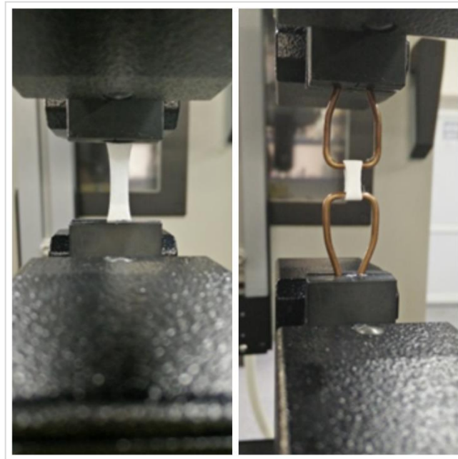
Рисунок 2.5 Образцы синтетических каркасов желчного протока во время испытаний в различных режимах
