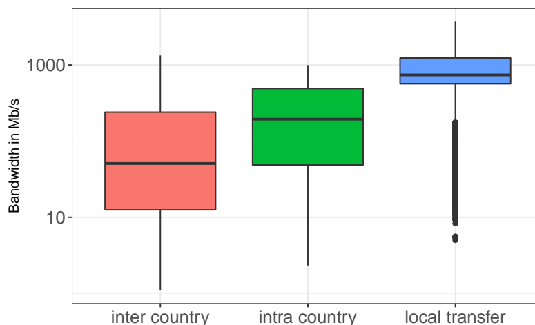
Figure 8.1: Distribution de la bande passante expérimentée par 11 033 transferts de fichiers de release selon différentes catégories de liens.
