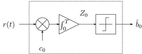
FIGURE 5.2: Récepteur conventionnel par corrélation
