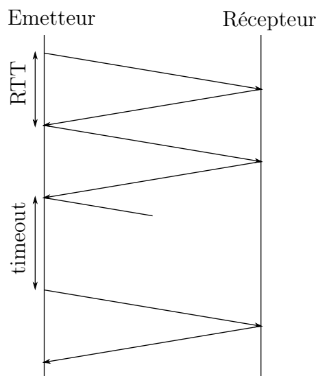
FIGURE 4.1: Chronogramme d'une transmission avec ARQ stop and wait
