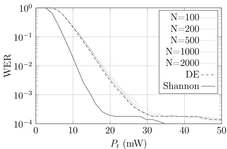
FIGURE 3.8: Performances des codes LDPC pour R = 1/2 et pour différents N sur le canal optique avec R_b = 1 Mb/s
