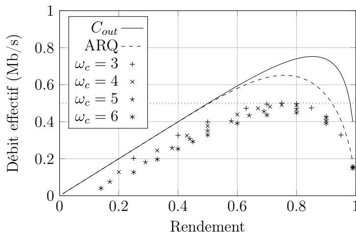
FIGURE 4.10: Débit atteignable avec ARQ (niveau applicatif) et codes LDPC (couche physique) pour P_t = 12.5 mW et R_b = 1 Mb/s
