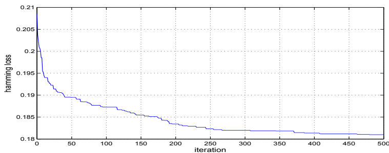
Figure 3.6 – Évolution pour ML-ARP, sur le jeu de données Emotions, de la performance de Hamming loss sur l'ensemble d'apprentissage au cours des itérations (courbe moyenne obtenue sur 10 répétitions)
