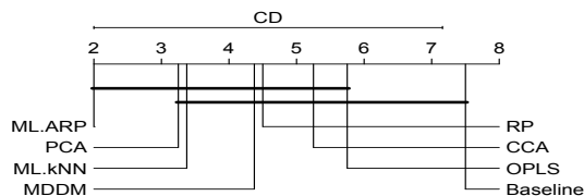
Figure 3.5 – Résultat du test statistique de Nemenyi pour tous les algorithmes sur quatre jeux de données (Yeast, Emotions, Scene, Enron).
