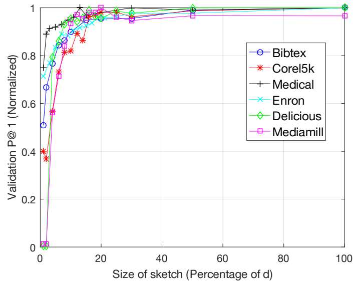
Figure 4.5 – Évolution de la performance en validation P@1 (normalisée par sa valeur maximal) en fonction de la taille m du "count-sketch" (exprimée comme un pourcentage de d ) pour t = 10 .
