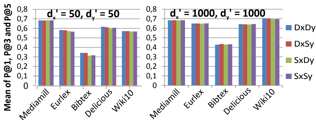
Figure 5.3 – Comparaison des quatre variantes de diversité (SxSy, SxDy, DxSy, DxSy) pour deux valeurs de (d'_x, d'_y) pour une forêt de cinquante arbres.
