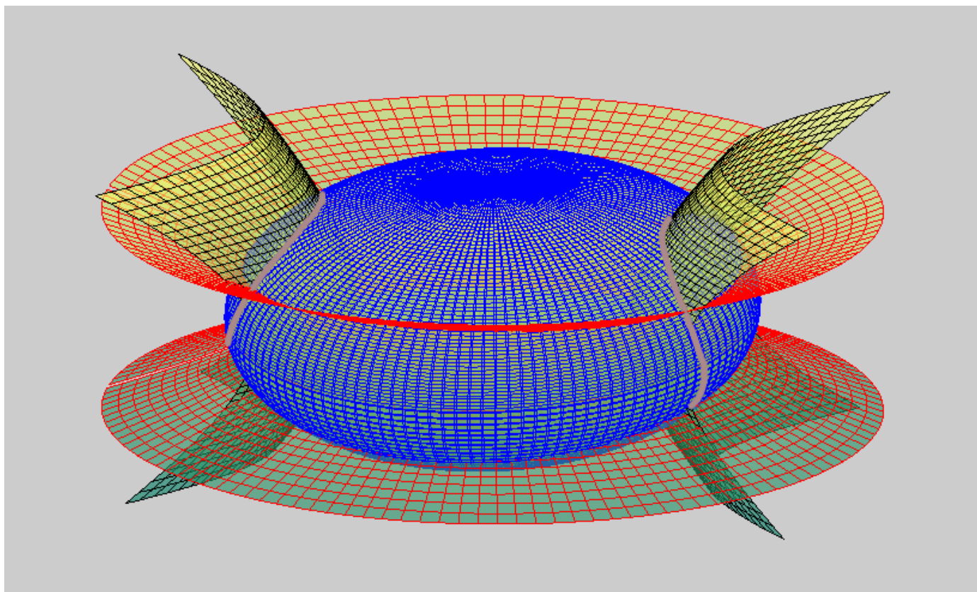
FIGURE 22. Trois surfaces appartenant à un système de "trajectoires orthogonales" 97 se coupent selon leurs lignes de courbure d'après le théorème de Charles Dupin (1813)
