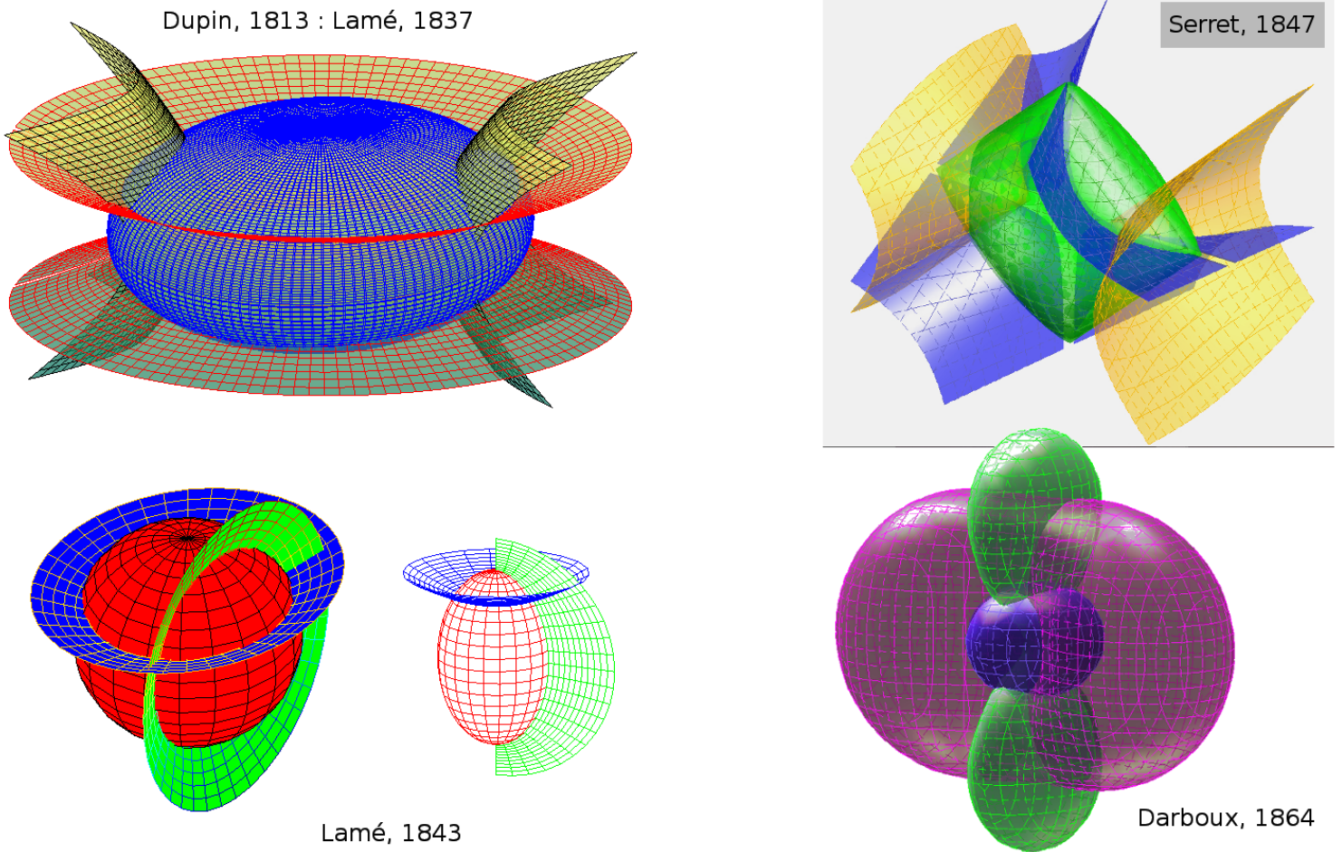
FIGURE 26. Quelques systèmes triples orthogonaux connus au début des années 1870
