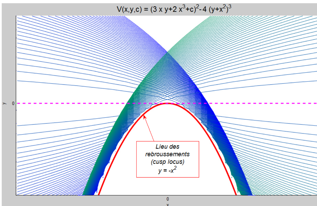
FIGURE 20. Illustration des lieux d'inflexion et de rebroussement
