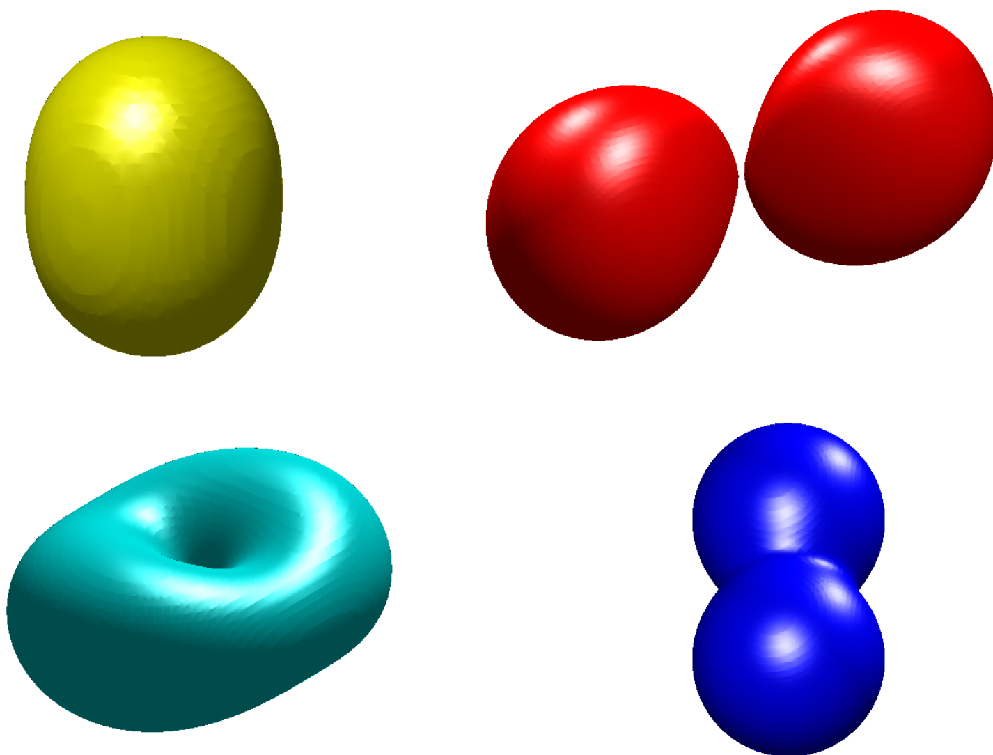
FIGURE 11. Différentes formes des cyclides de Darboux 39
