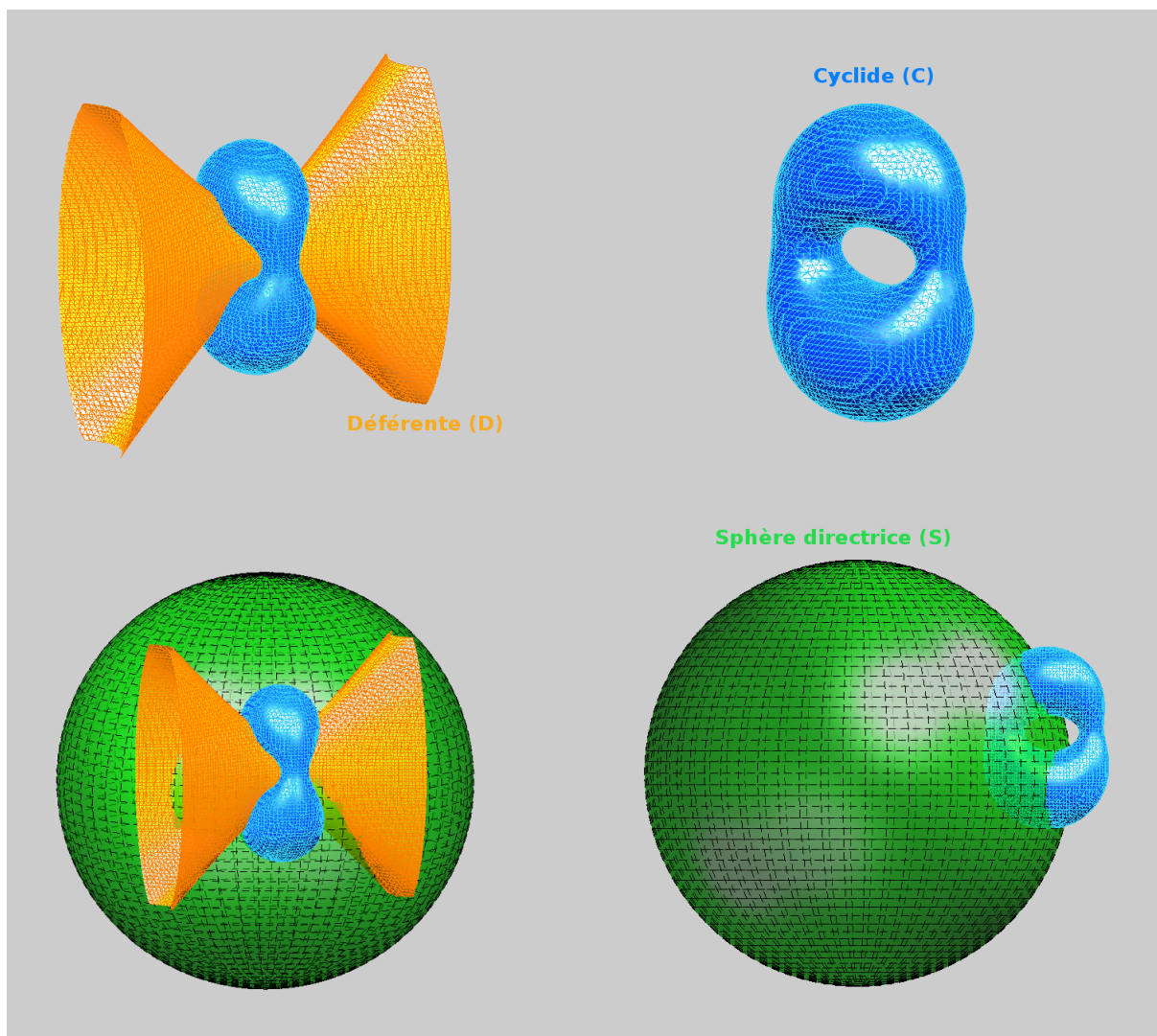
FIGURE 36. Une cyclide à connexion triple ( C ), représentée avec une de ses déférentes ( D ) (un hyperboloïde à une nappe) et la sphère directrice (d'inversion) réelle associée ( S ) 218
