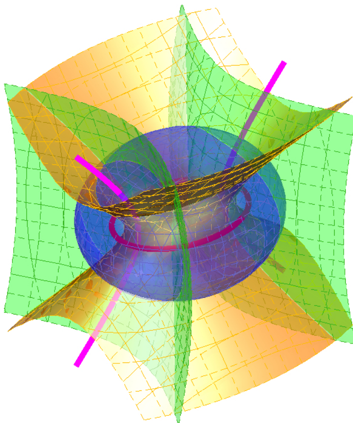
FIGURE 1. Un triplet de surfaces issu du système triple orthogonal de Lamé formé d'ellipsoïdes (en bleu), d'hyperboloïdes à une (en jaune) et à deux (en vert) nappes. 7
