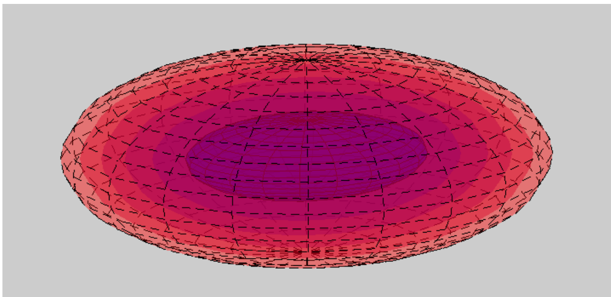
FIGURE 13. Répartition de la chaleur dans un solide délimité par deux ellipsoïdes homofocaux maintenues à deux températures constantes : la famille de surfaces isothermes \mathcal{E} est formée par des ellipsoïdes de même type d'après Lamé.
