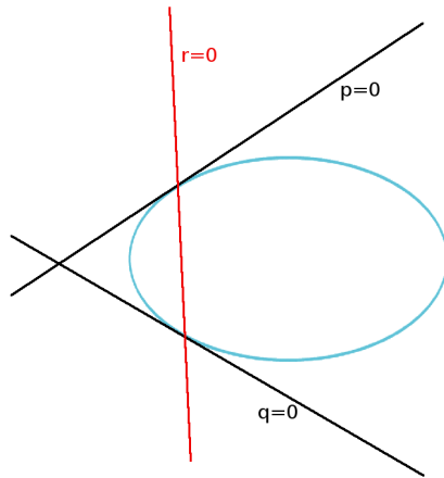
FIGURE 7. Les trois droites (deux tangentes et la sécante de contact) utilisées dans la définition des coordonnées linéaires donnent l'équation de l'ellipse (bleu) suivante : pq + \mu r^2 = 0
