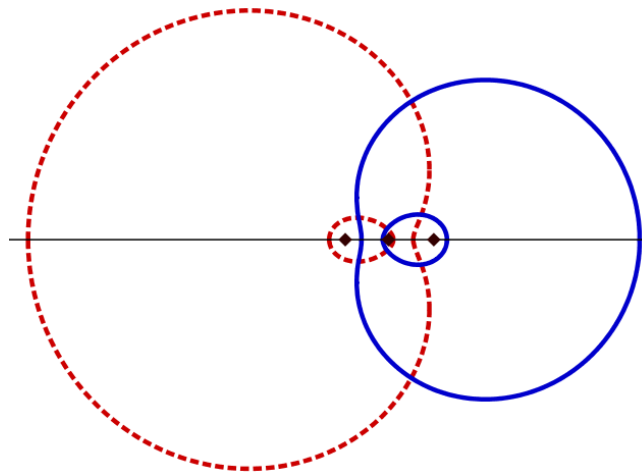
FIGURE 10. Deux ovales de Descartes homofocales orthogonales
