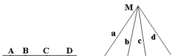
FIGURE 16. Configurations planes pour l'emploi du rapport anharmonique de quatre éléments
