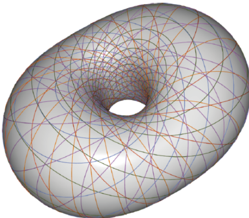
FIGURE 38. Les six séries de sections circulaires d'une cyclide à connexion triple 245
