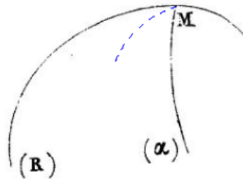
FIGURE 19. Configuration géométrique du raisonnement de [Darboux 1870c]
