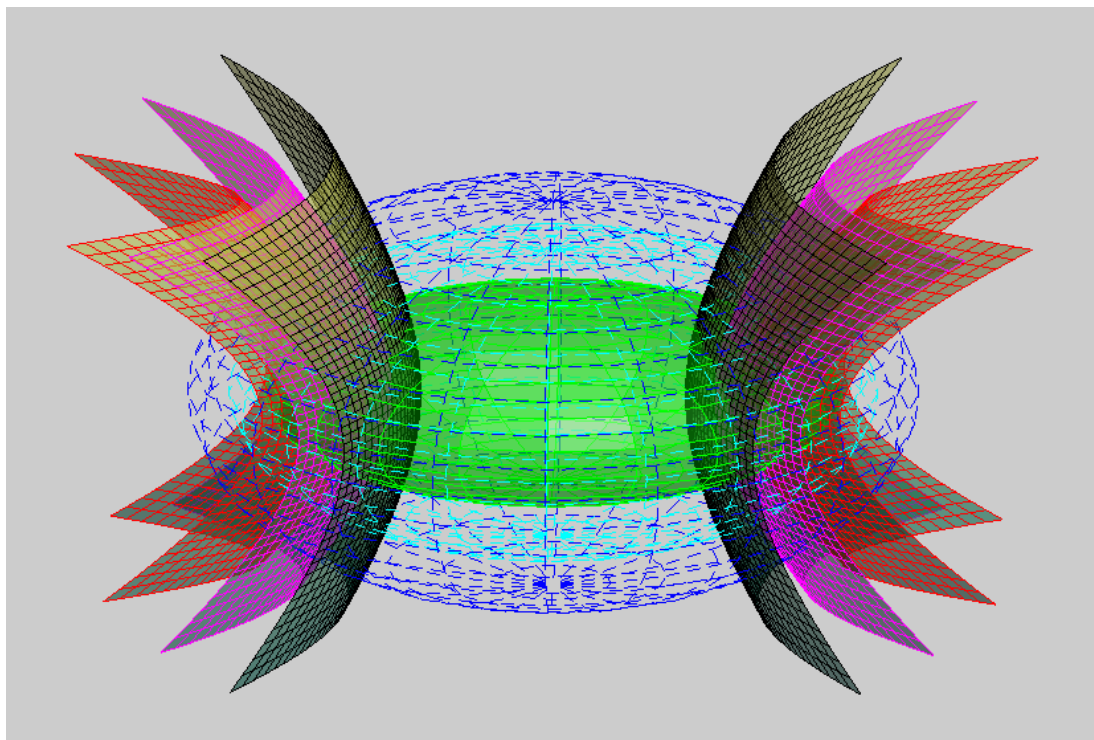
FIGURE 25. D'après l'extension de Darboux du théorème de Dupin, pour que les familles homofocales d'ellipsoïdes et d'hyperboloïdes à deux nappes fassent partie d'un système triple, il faut et il suffit que les surfaces se coupent suivant leurs lignes de courbure.
