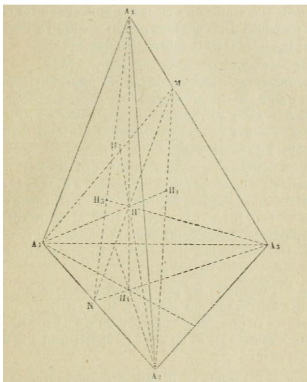
FIGURE 32. Un tétraèdre orthocentrique 187
