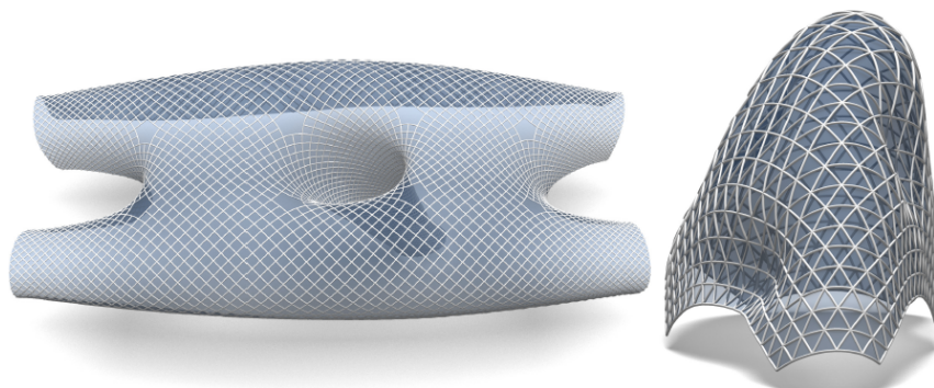
FIGURE 39. Deux structures libres de forme par la méthode des arcs circulaires (CAS) 246
