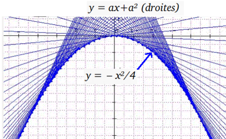
FIGURE 10. Les deux types de solutions déterminées par Clairaut
