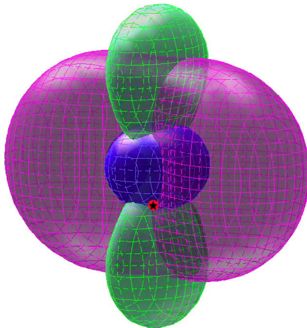
FIGURE 12. Un triplet de surfaces issu du système triple orthogonal des cyclides homofocales de Darboux. Un des douze points de triple orthogonalité est mis en évidence (en rouge)
