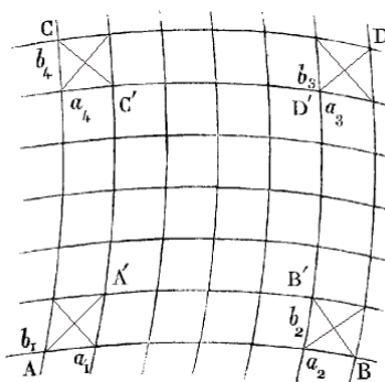
FIGURE 17. Support géométrique pour Bertrand des deux conditions nécessaires à l'isothermie d'un système triple orthogonal ([Bertrand 1844a, 123-125])
