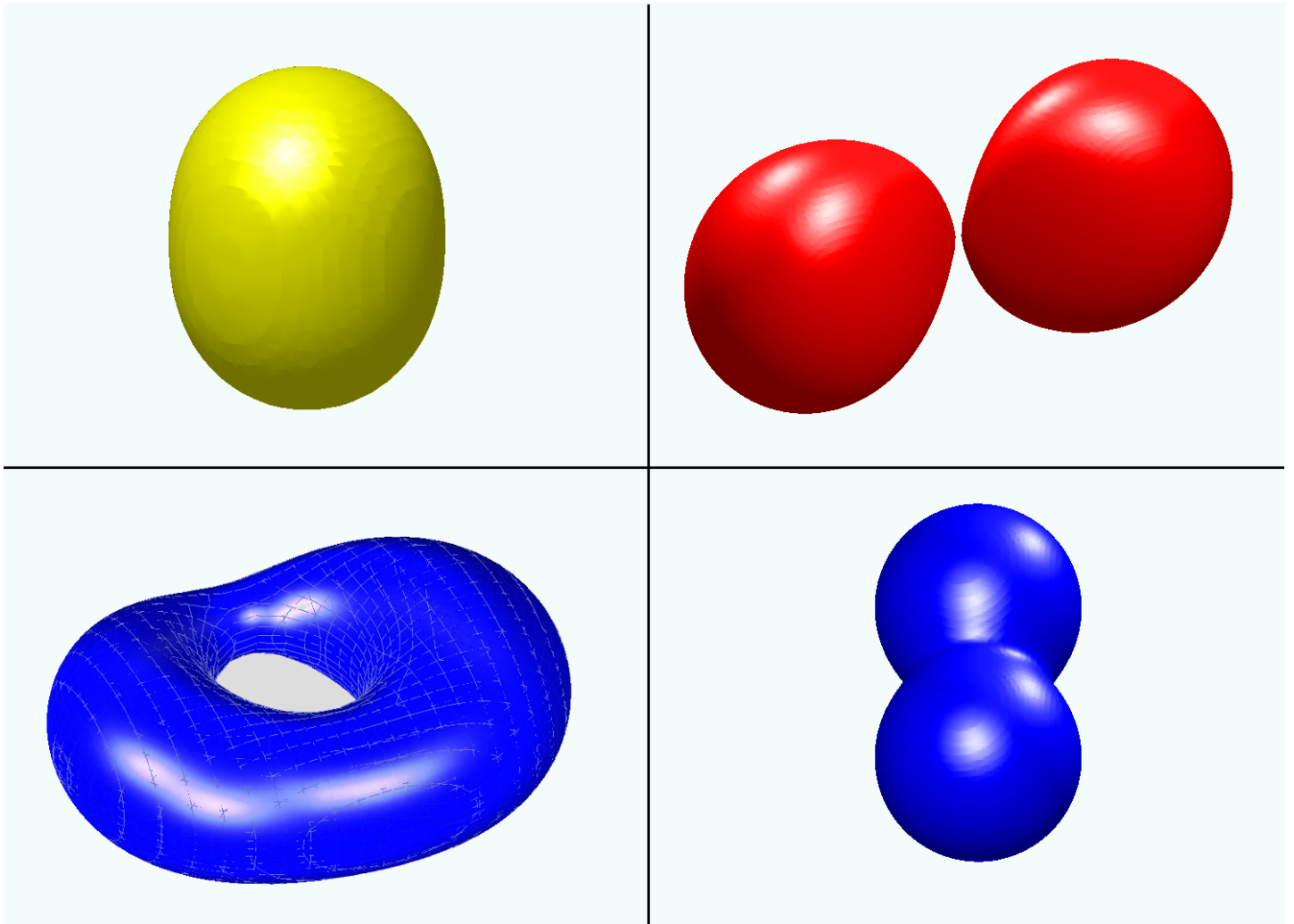
FIGURE 35. Les quatre différentes formes topologiques des cyclides de Darboux
