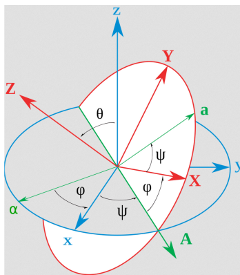
FIGURE 24. Définition des 3 angles d'Euler
