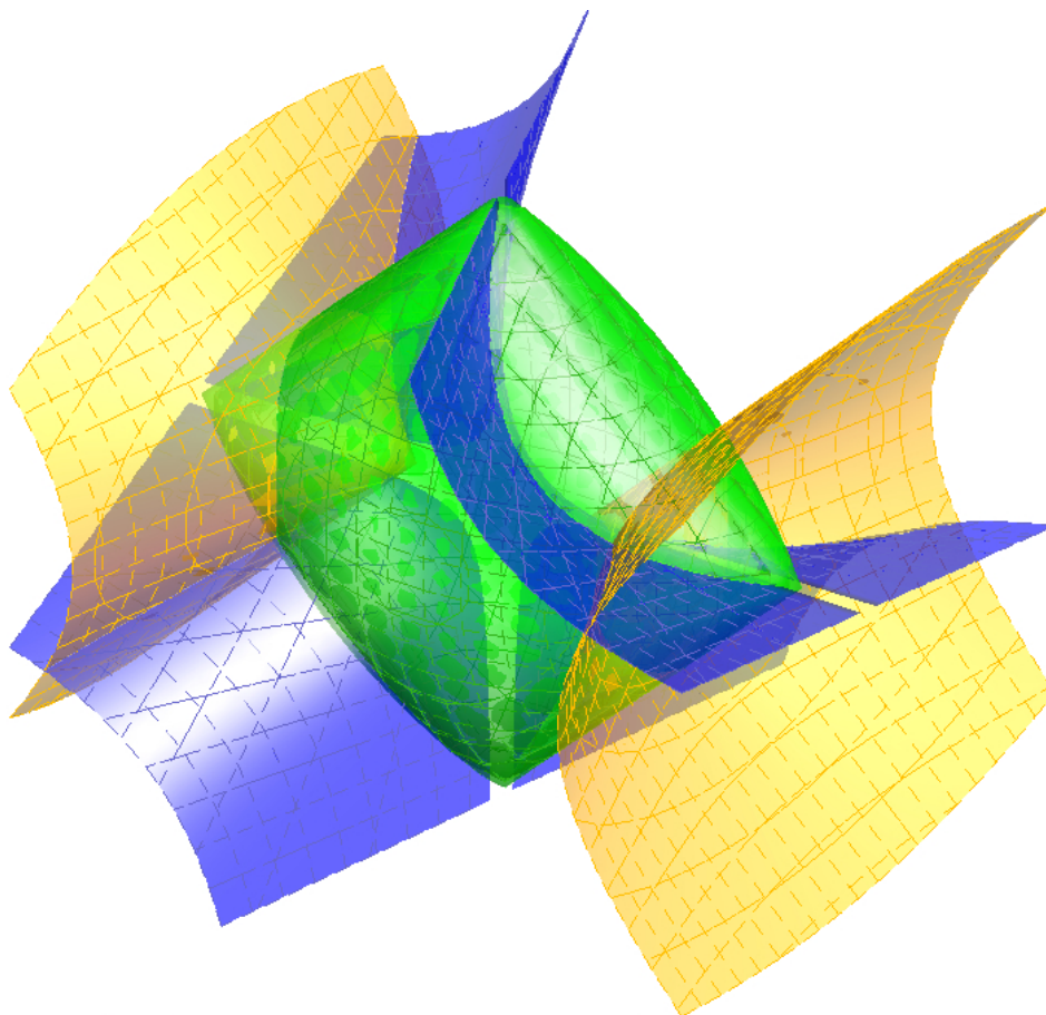
FIGURE 3. Un triplet de surfaces issu du système triple orthogonal de Serret formé d'un parabolôïde hyperbolique (en bleu) et de deux surfaces du quatrième ordre, l'une à une nappe (en vert), l'autre à deux (en jaunes).
