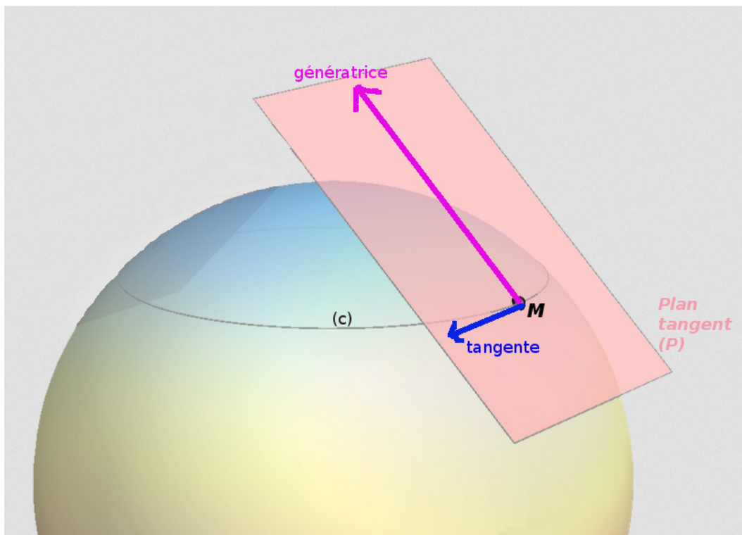
FIGURE 21. Configuration géométrique de la définition des tangentes conjuguées de Charles Dupin
