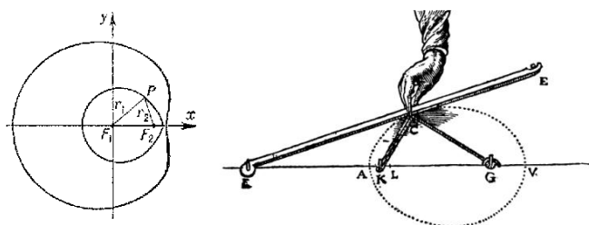
FIGURE 4. Un(e) ovale de Descartes (à gauche), et l'image de la construction "mécanique" de l'ovale donnée par Descartes 15
