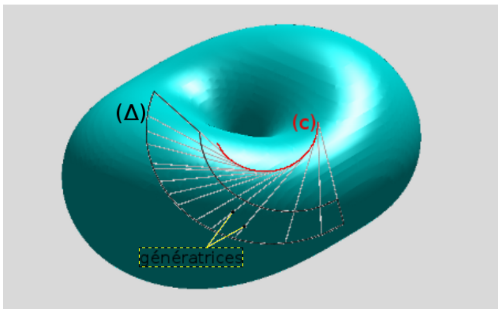
FIGURE 29. Construction d'une surface développable ( \Delta ) tangente à un cyclide le long de l'arête de rebroussement ( c )
