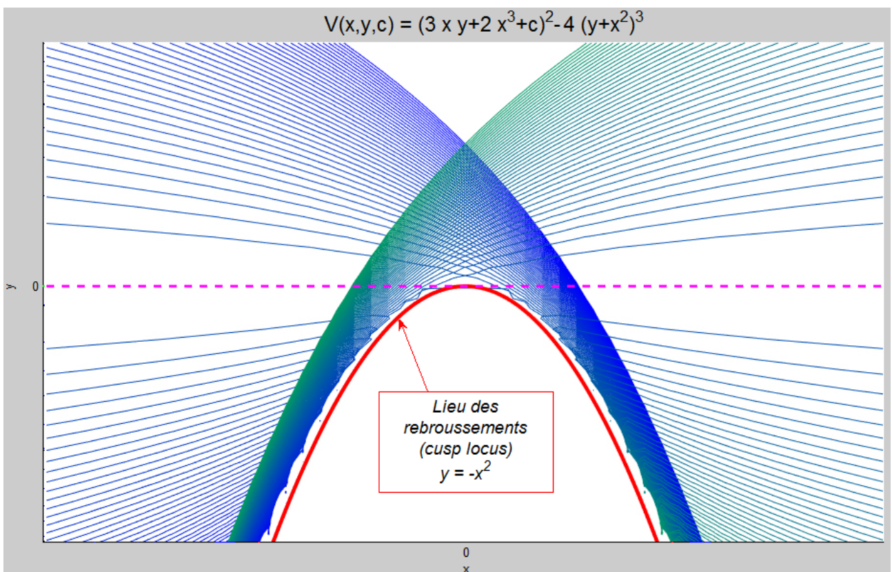
FIGURE 20. Illustration des lieux d'inflexion et de rebroussement
