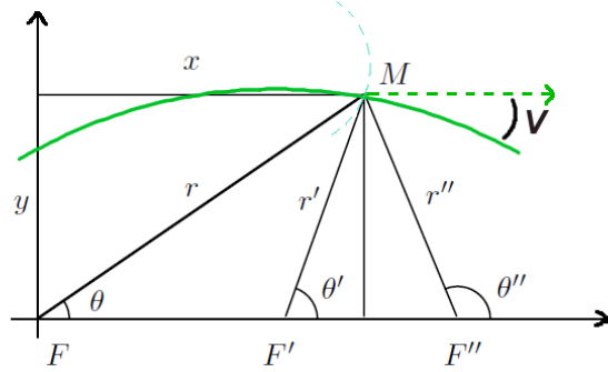
FIGURE 9. Configuration et notations pour la démonstration de Darboux d'orthogonalité des ovals homofocales 36
