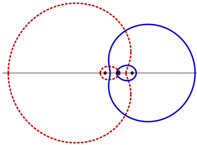
FIGURE 10. Deux ovales de Descartes homofocales orthogonales
