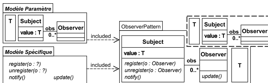
FIGURE 3.5 – Constituants d'un aspectual template : Sous-modèle paramètre et sous-modèle spécifique
