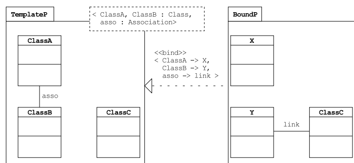
FIGURE 2.35 – Erreur concernant une des propriétés d'une association (Source :Caron et al. [23])
