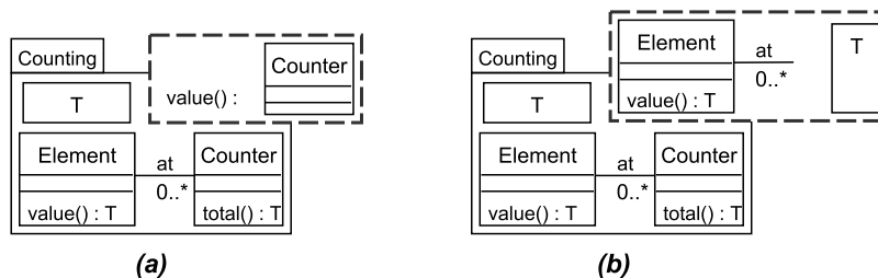
FIGURE 4.18 – Exemples d' aspectual templates mal-formés
