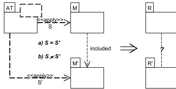
FIGURE 3.52 – Étude de la relation entre R et R' via des applications (a) identiques ( S = S' ) et (b) différentes ( S \neq S' )
