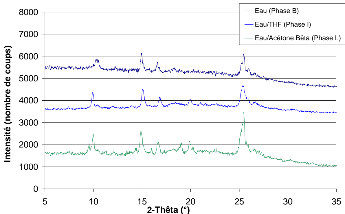
Annexe P : Clichés DRX des phases I, B et L
