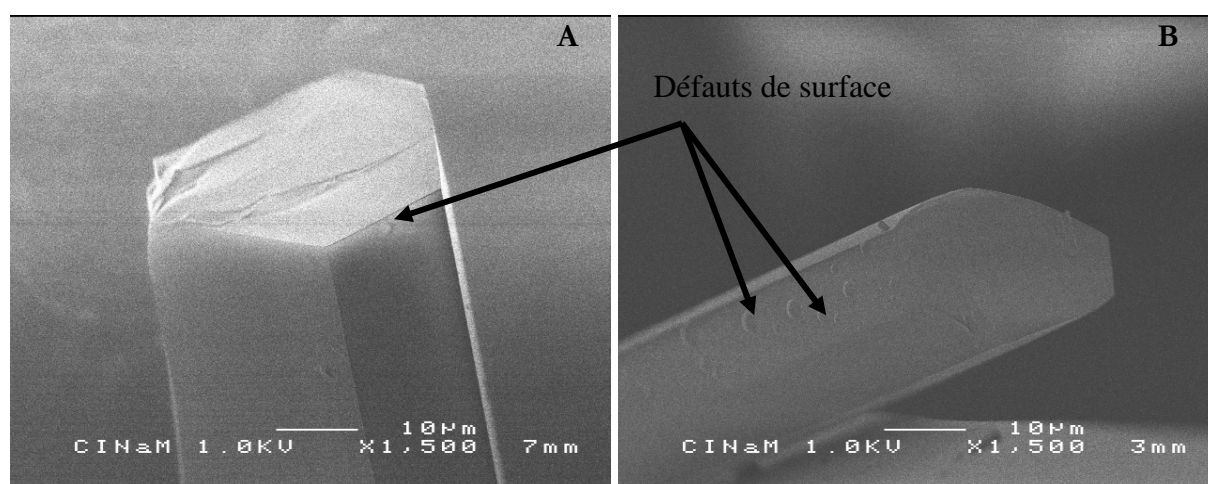
Figures 152 : Images MEB *1500 (A) et *1500 (B) des monocristaux de base
