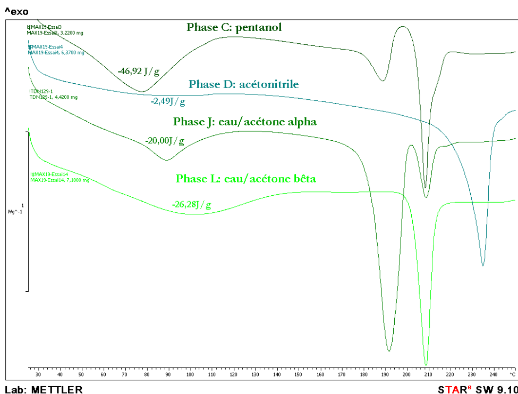
Figure 124 : Enregistrements DSC pour les phases cristallines C, D, J, L
