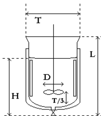
Figure 77 : Schéma d'un réacteur homothétique
