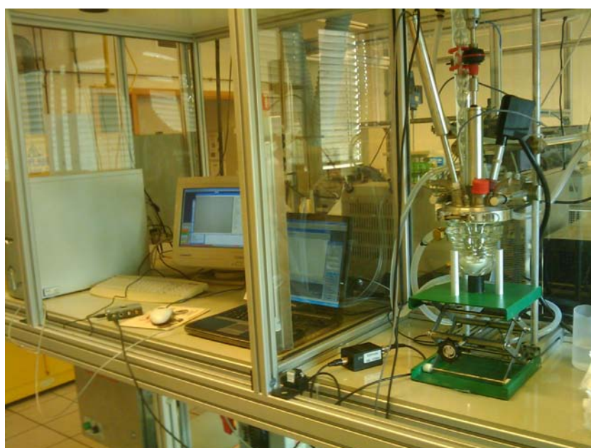
Figure 179 : Montage du LAGEP avec les sondes Pt100, vidéo in situ et FBRM
