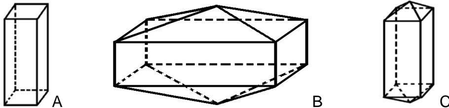
Figure 20 : Monocristaux A B et C
