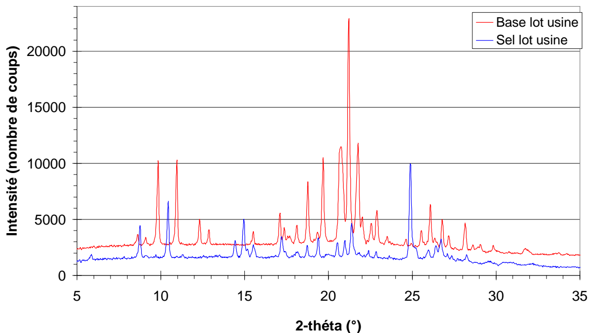
Figure 94 : Clichés DRX de la base et du sel TD901 – lots usine
