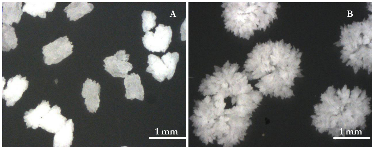
Figures 147 : Photos prises à la binoculaire pour les échantillons obtenus à partir de 24 g/L (A) et 8 g.L -1 (B) de base TD901
