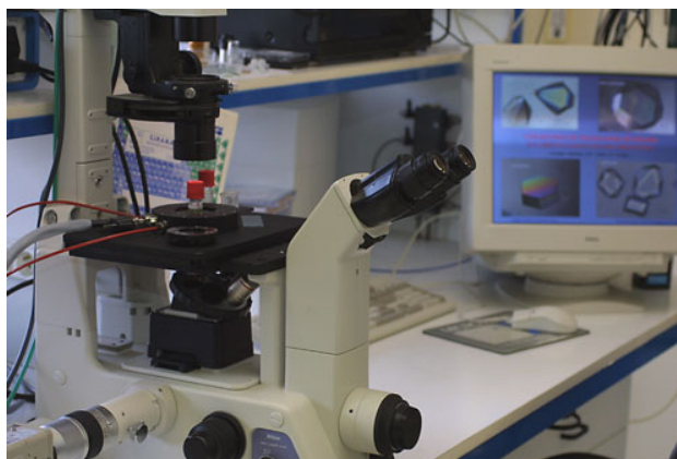
Figure 39 : Microscope optique inversé équipé d'une platine à effet Peltier
