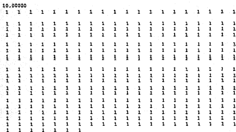
Figure 30 : matrice de niveau 10,0 correspondant à la figure ci-dessus. La matrice des 387 objets présente alors le chiffre 1 pour l'ensemble des objets (rangés dans l'ordre d'apparition du fichier par l'application BIOGÉO).
