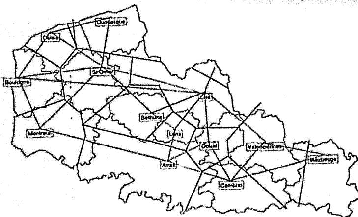
Figure 2 : résultat du modèle. On distingue une trame de base dont les droites relient certains pôles entre eux. À partir de ces droites sont ensuite tracés les points d'équilibre et leur droite (parfois perpendiculaire c'est-à-dire formant un angle droit) pour tracer les aires d'attraction fermant chaque pôle. Source ( Vigneron , 1994, p. 54).
