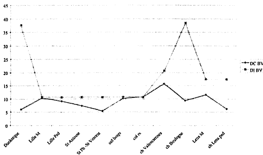
Figure 5 : courbes des valeurs de \bar{D}_c et \bar{D}_i (km) au niveau des bassins de vie. Les valeurs de \bar{D}_i sont dans l'ensemble supérieures elles aussi aux valeurs de \bar{D}_c . Les valeurs de \bar{D}_i sont équivalentes pour les 2 ème au 7 ème établissements. Une forte amplitude est à noter également pour Boulogne-sur-Mer mais aussi pour Dunkerque.
