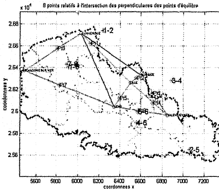
Figure 27 : phase 2 tracé des points d'intersection (selon les plus proches voisins points d'équilibre) du modèle « P » relatifs aux perpendiculaires qui seront tracées depuis les coordonnées des points d'équilibre
