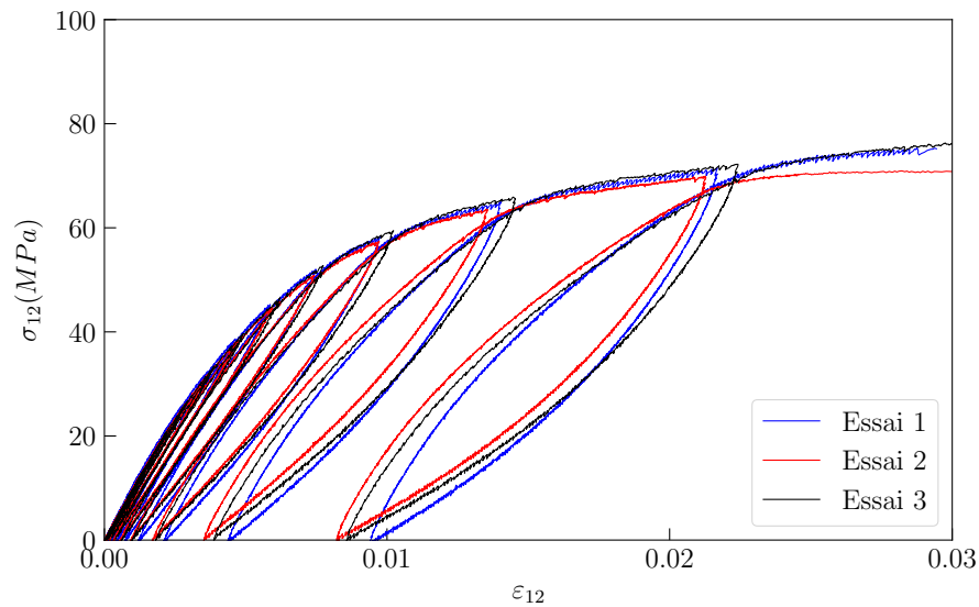
FIGURE 4.9 – Comparaison entre les courbes contrainte / déformation des trois essais réalisés à 5 mm/min et à température ambiante pour le [\pm 45^\circ]_s T700GC/M21.
