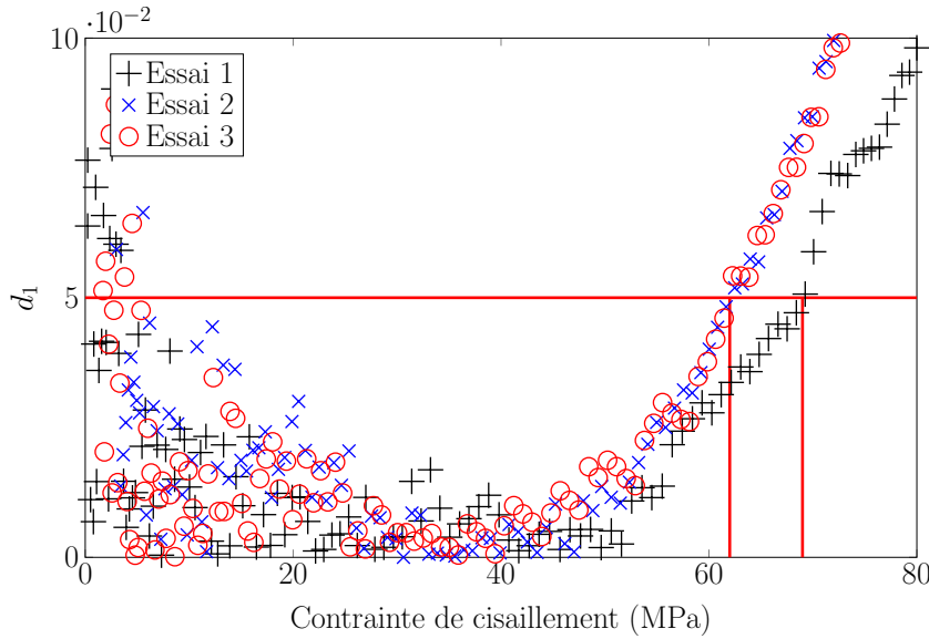
FIGURE 2.12 – Détermination de la contrainte de transition \sigma_{d_{5\%}} pour un essai à 20^{\circ}\text{C} et 50\text{s}^{-1} .
