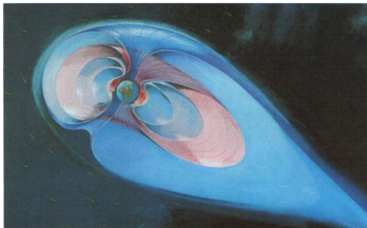
Figure 5- Vue d'artiste de la magnétosphère Les lignes de champ magnétique deviennent, dans cette représentation en trois dimensions, des surfaces qu'on appelle des coquilles magnétiques [Lilensten and Bornarel 2001].
