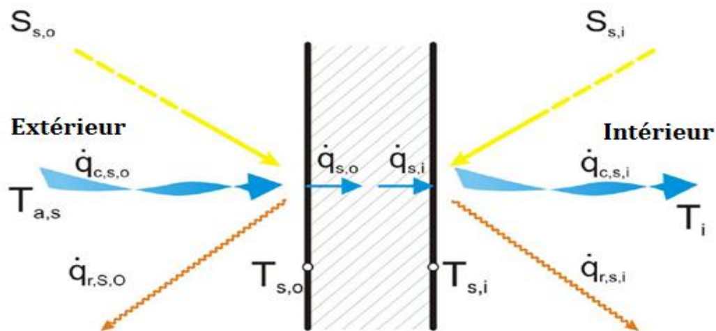
Figure A.1. Flux de chaleur et températures d'une paroi de bâtiment (TRNSYS 2010)
