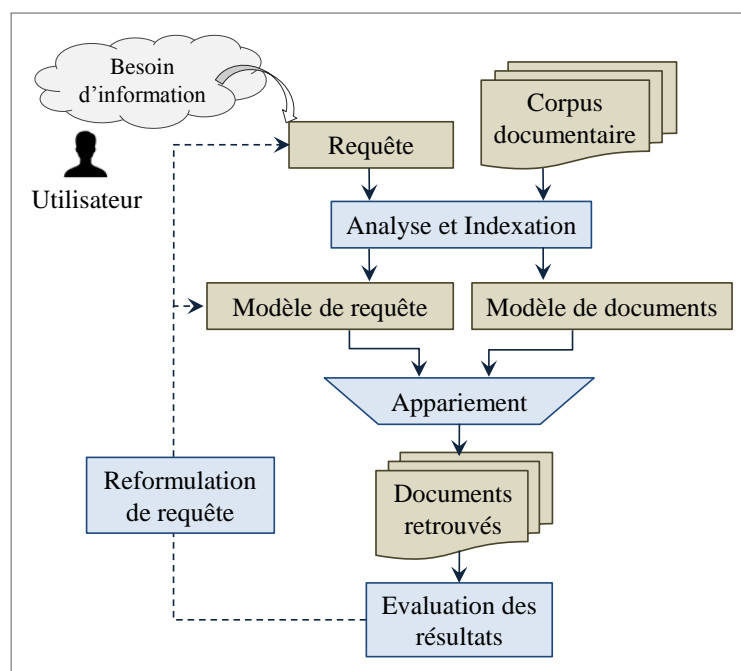
Figure 1.1 – Architecture générale d'un SRI
