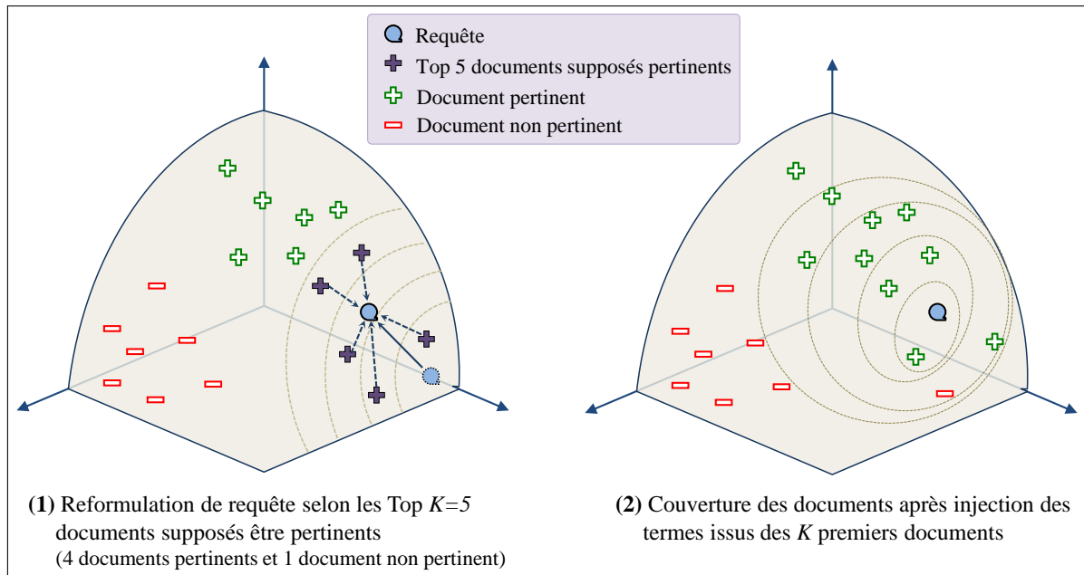
Figure 3.4 – Exemple de modélisation de la pseudo-rétroaction de pertinence avec K=5 top documents [Lavrenko, 2008]
