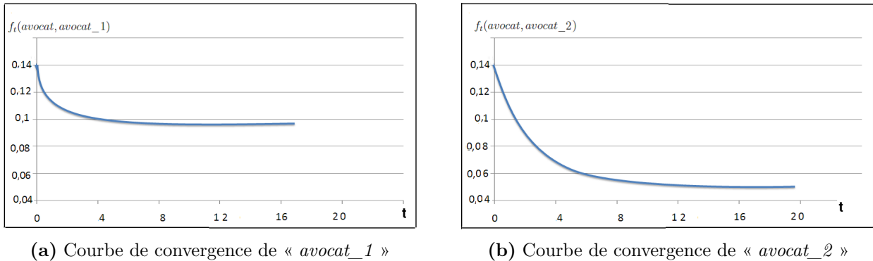
Figure 5.9 – Courbes de convergence des sens « avocat_1 » et « avocat_2 »
