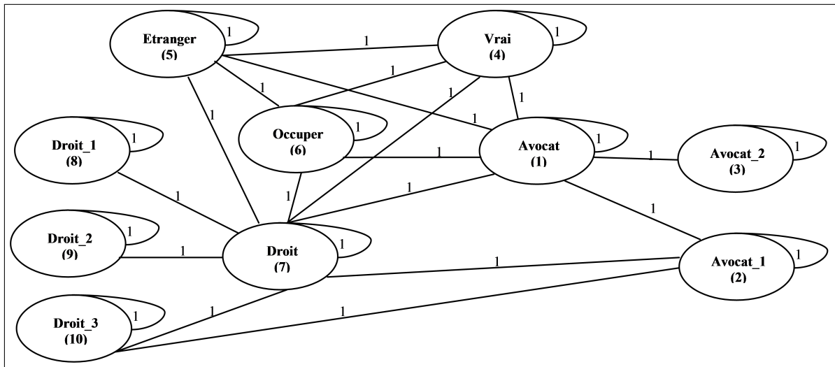
Figure 5.8 – Graphe sémantique de l'exemple PH1
