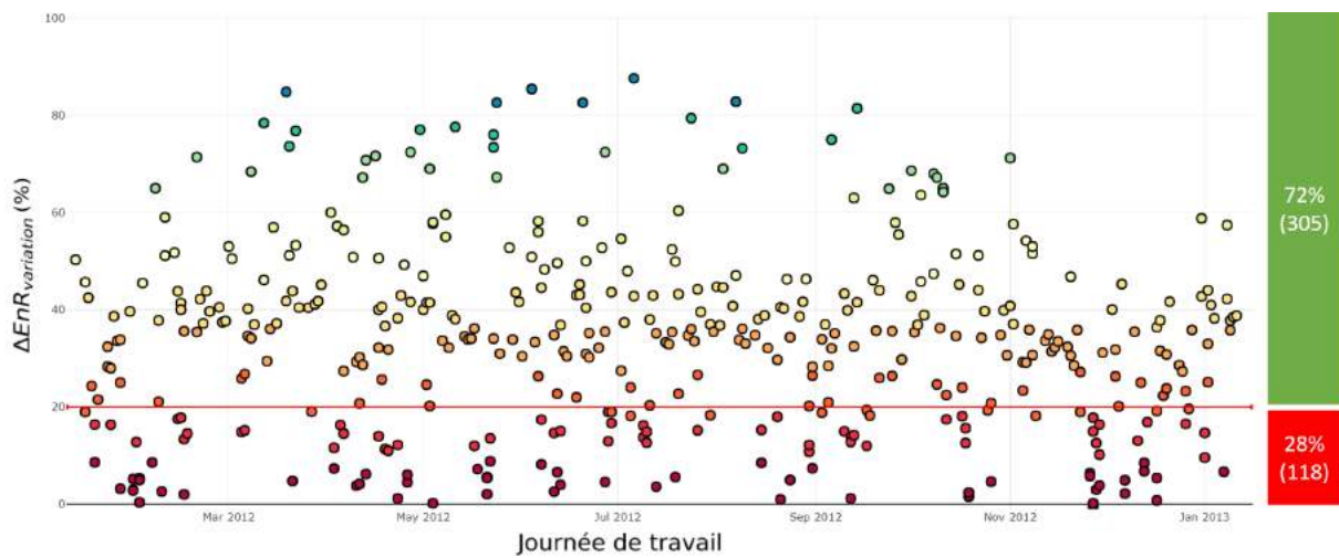
FIGURE 8.15 – Les variations de production d'énergie solaire sur une année de travail en fonction de \Delta EnR_{variation} pour duration_{decharge} = 3h et duration_{charge} = 1h (8h-17h, lundi-vendredi, 13 janvier 2012-12 janvier 2013, installation photovoltaïque ESTIA, Bidart, France).
