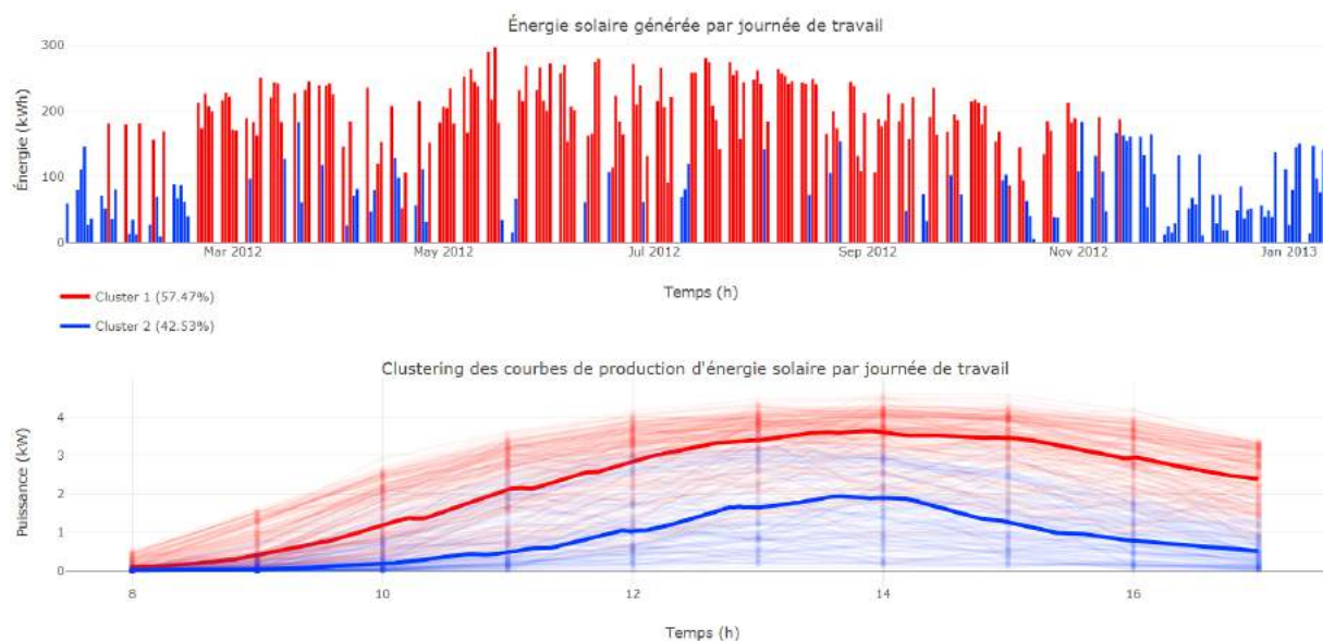
FIGURE 8.9 – Le clustering des courbes de production d'énergie solaire d'une année de travail (8h-17h, lundi-vendredi, 13 janvier 2012-12 janvier 2013, installation photovoltaïque ESTIA, Bidart, France).
