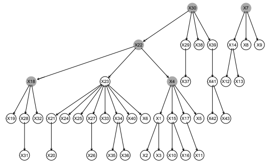
(d) BN learned with ds-BNSL on D_2
