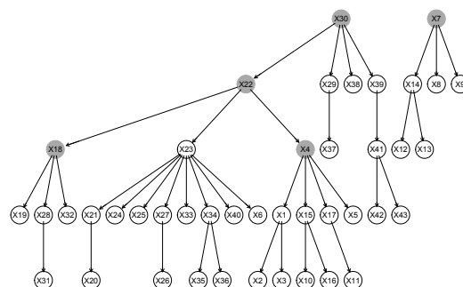
(d) BN learned with ds-BNSL on D_2
