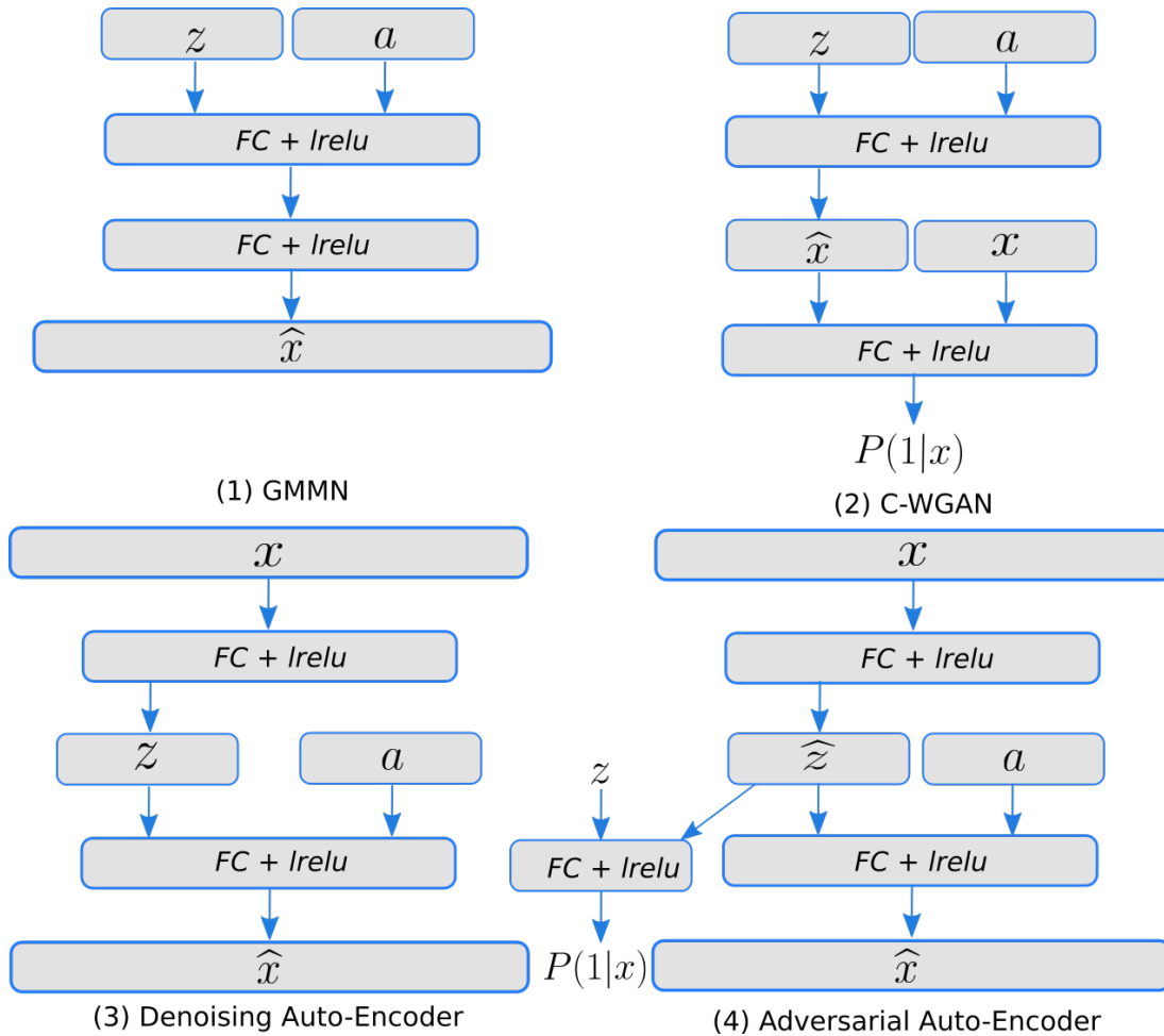
FIGURE 2.6 – Architecture des modèles génératifs proposés. z : bruit gaussien, a : description sémantique, FC + lrelu : couche entièrement connectée suivie d’une fonction non linéaire type «Leaky ReLUs» [99], \hat{x} : caractéristiques visuelles générées.
