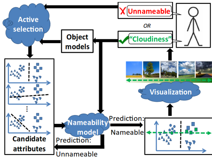
FIGURE 1.5 – Figure extraite de [122] : introduit une approche pour définir un vocabulaire d'attributs à la fois humainement compréhensible et discriminant. Le système prend en entrée des images étiquetées par objet/scène et renvoie en sortie un ensemble d'attributs obtenus par interactions avec un annotateur humain, chargé de distinguer les bons aux mauvais attributs.
