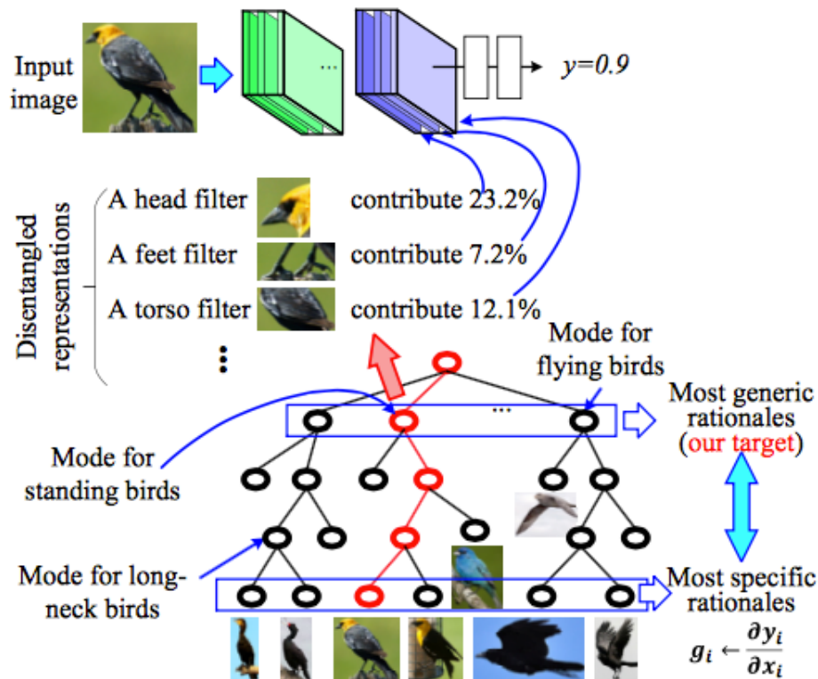
FIGURE 3.3 – Image extraite de [173] : étant donné une image d'entrée, l'arbre de décision analyse quelles parties d'objet sont utilisées dans la prise de décision.
