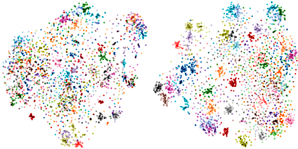
FIGURE 2.4 – Projection t-SNE 2D [100] de la représentation d’attributs (gauche) et des caractéristiques visuelles extraites d’un réseau convolutif ResNet [66] (droite). Cette figure confirme notre intuition, l’espace des caractéristiques visuelles est mieux organisé, plus structuré.
