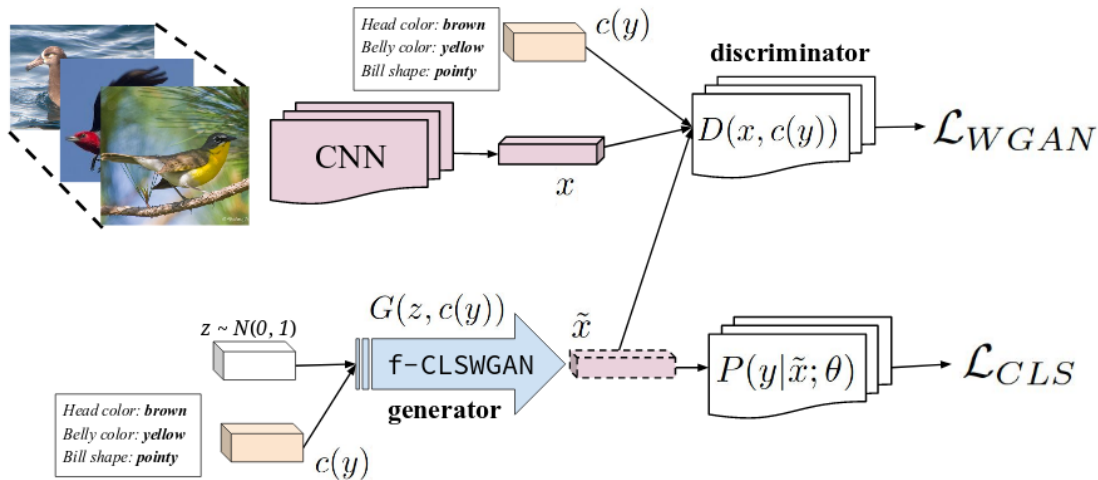
FIGURE 2.1 – Figure extraite de [164] : génération de caractéristiques visuelles pour les classes non vues grâce à un «Generative Adversarial Network», conditionné par une représentation d’attributs. Un critère de classification sur les caractéristiques générées permet d’affiner le résultat.
