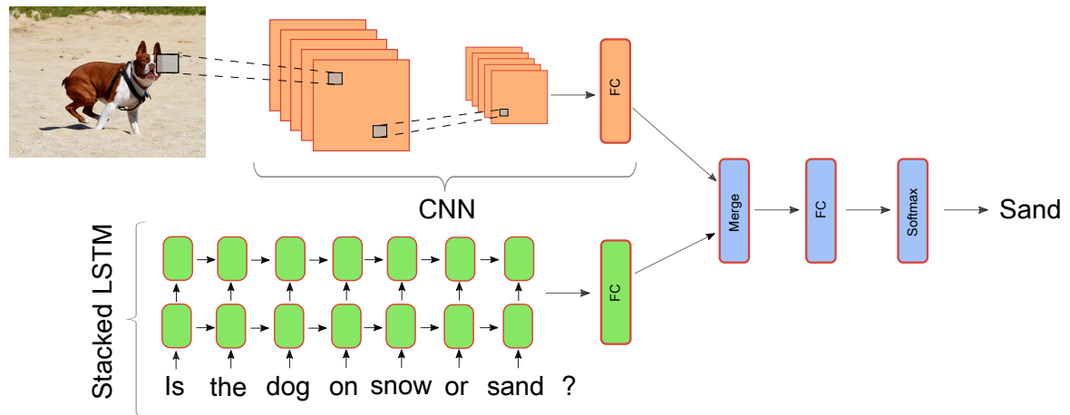
FIGURE 3.6 – «deeper LSTM Q + norm I» : (orange) les images sont représentées par la dernière couche cachée d’un réseau VGG-VeryDeep-19 [144]. (vert) Un LSTM à deux couches code les questions. (bleu) Les représentations de la question et de l’image sont fusionnées via une multiplication élément par élément et utilisées pour la prédiction de la réponse.
