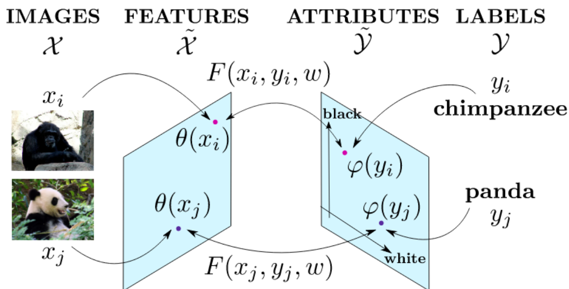
FIGURE 1.7 – Image extraite de [6] : \theta(\mathbf{x}) correspond aux caractéristiques de l'image \mathbf{x} . Les étiquettes de classes y sont représentées par un ensemble d'attributs \phi(y) . La fonction de score est F(\mathbf{x}, y; \mathbf{W}) .
