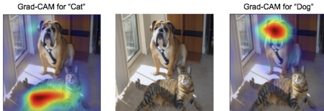
FIGURE 0.5 – Image extraite de [137] : les cartes de saillance générées permettent de visualiser les zones de l'image utilisées pour la prise de décision.
