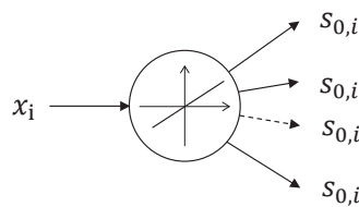
FIGURE 2.3 – Neurone de la couche d'entrée.
