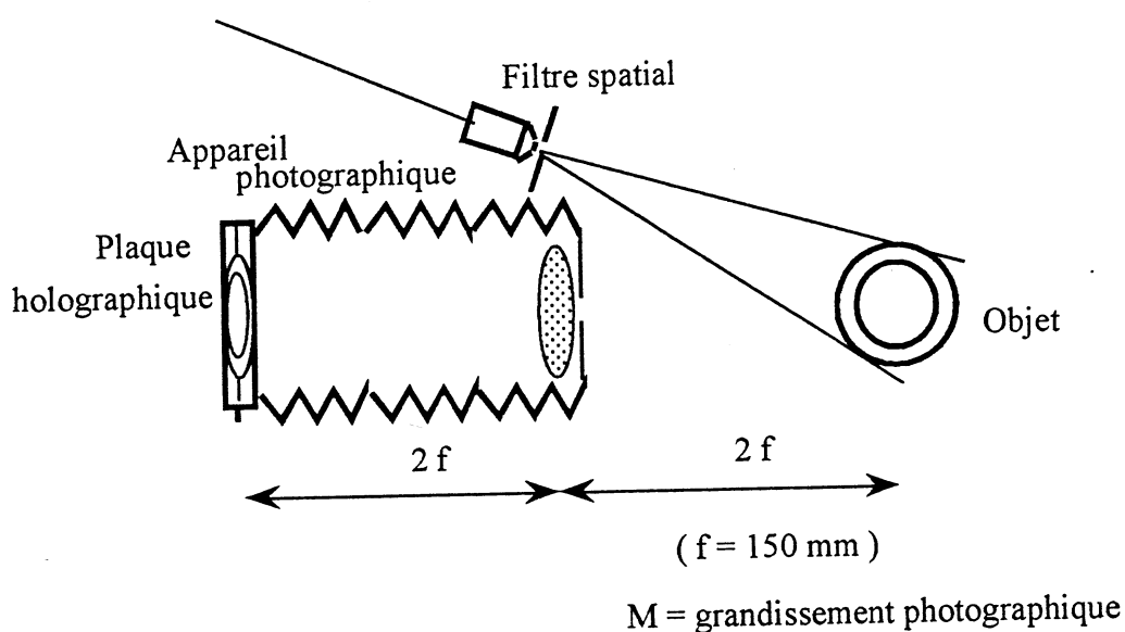
Fig.3.6: Dispositif d'enregistrement.
