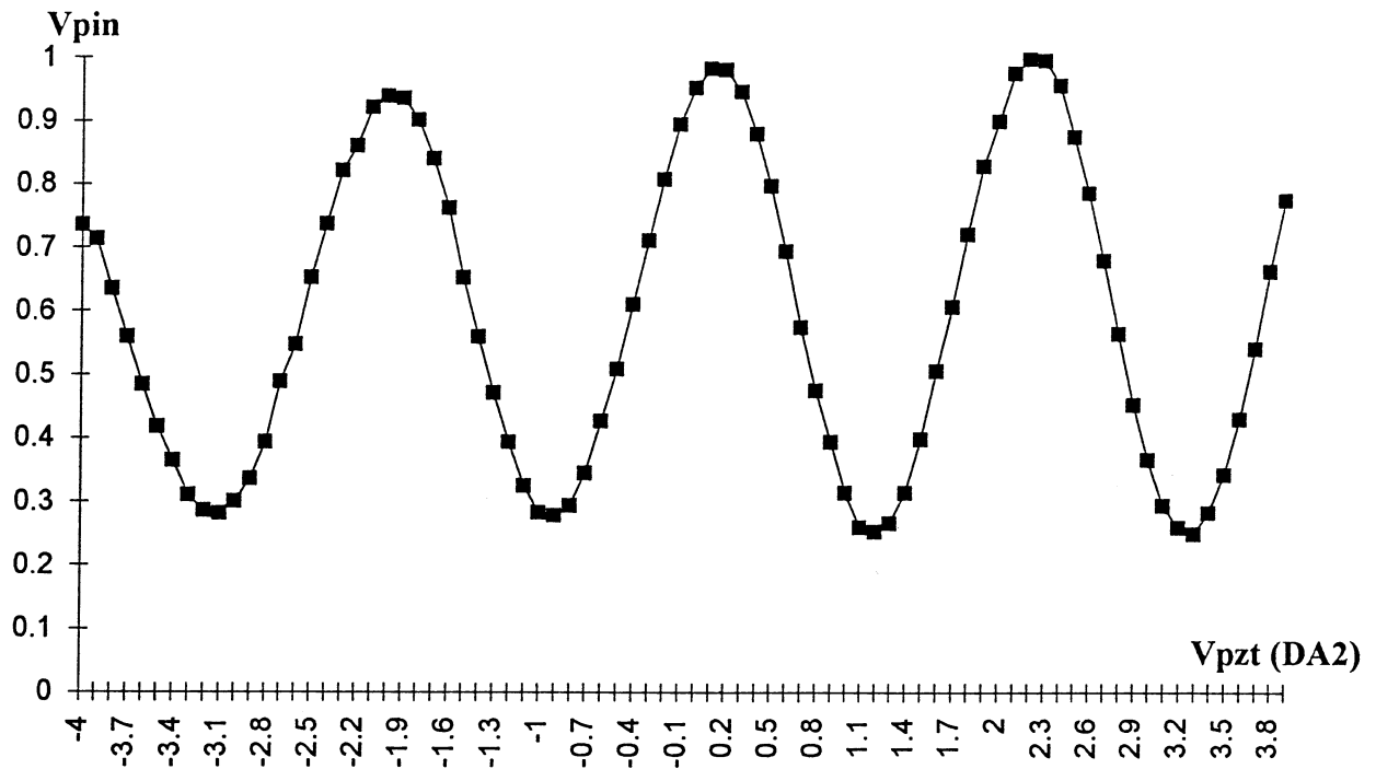
Fig.5.11.b: Tension de sortie de la photodiode: Calibration en tension du PZT DA2 à 633 nm.
