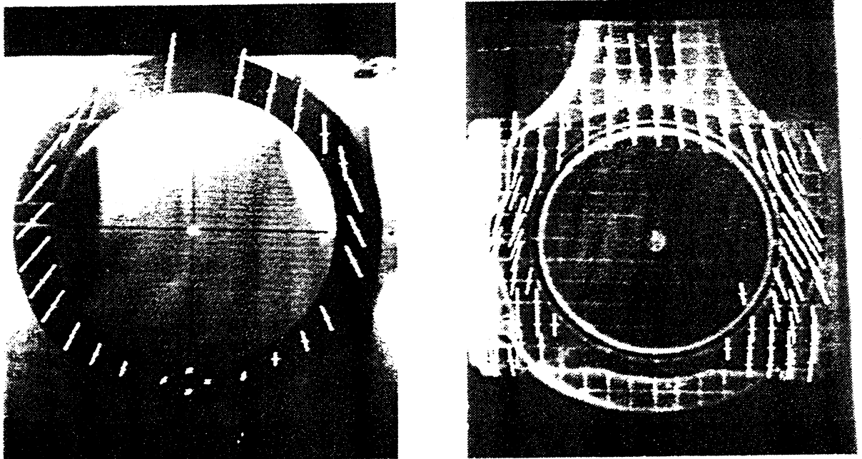
Fig.3.8: Résultat du dépouillement automatisé: Anneau en compression diamétrale Bielle en traction (source J.-L. Guey).
