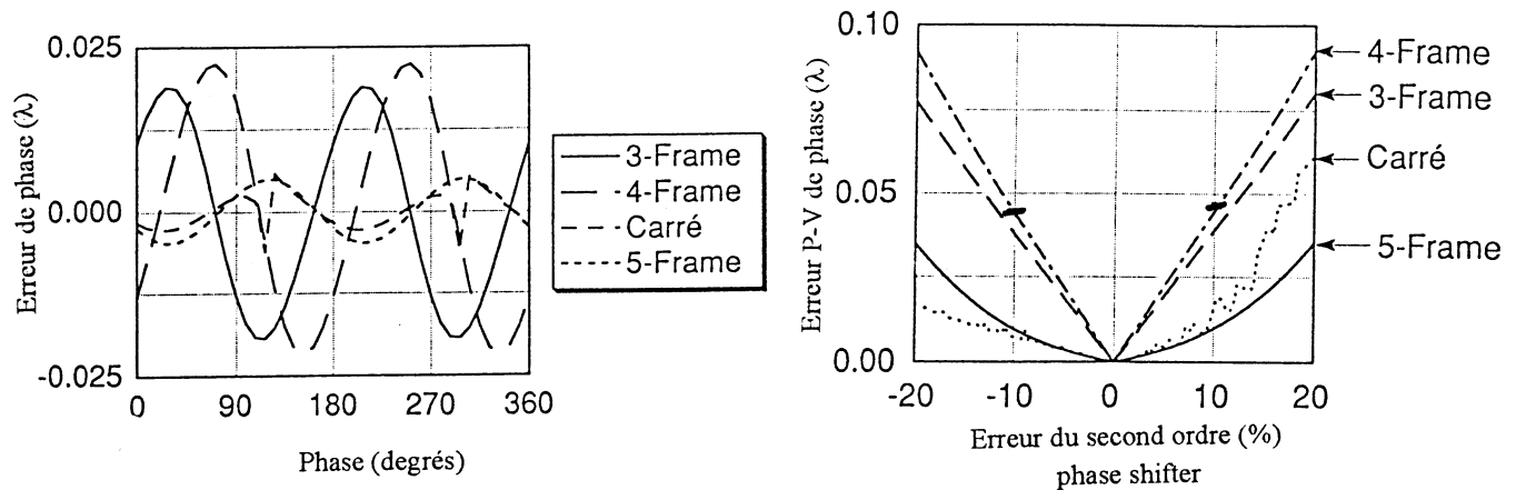
Erreur de phase ( \lambda ) en fonction de la phase initiale ( \epsilon = 10\% ) Erreur P-V en fonction de \epsilon
