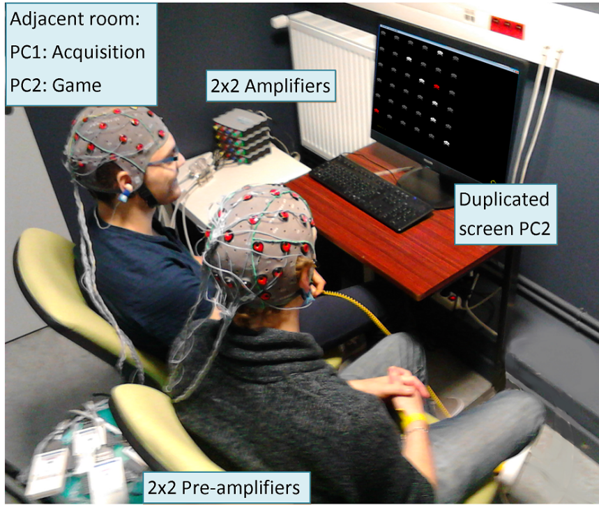
FIGURE 3.5 – Organisation expérimentale de Brain Invaders 2 à deux joueurs. Les deux sujets sont à environ 1,25 mètres d'un écran de 24 pouces de diagonale et sont côte-à-côte durant l'ensemble de l'expérience. Chaque sujet est connecté à un système g.Tec avec 32 électrodes actives dont 16 seront utilisées pour la classification en temps réel (deux pré-amplificateurs et deux amplificateurs par joueurs). L'expérimentateur est situé dans une salle adjacente et il peut observer la bonne tenue de l'expérience au travers d'un miroir sans tain (non visible sur cette image).
