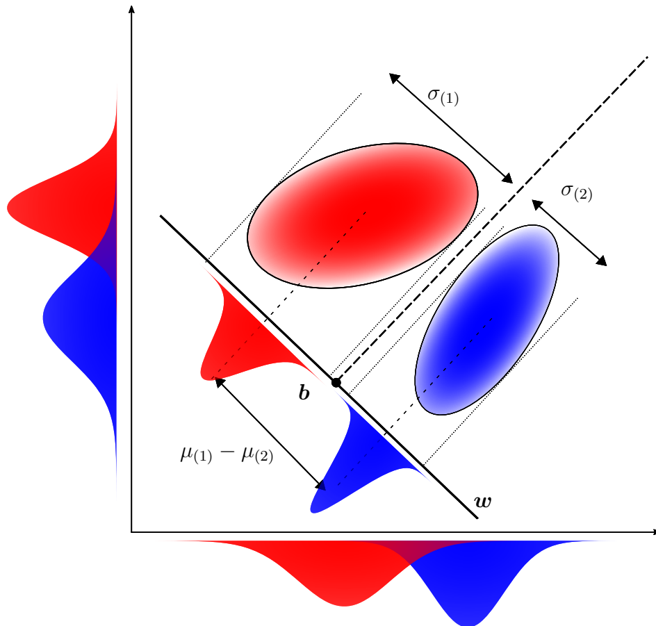
FIGURE 2.7 – Pour deux distributions de données (rouge et bleu), le LDA permet de trouver une séparation linéaire grâce au vecteur perpendiculaire \mathbf{w} (et le seuil \mathbf{b} ) définissant le (hyper)plan (ici la ligne noire hachurée) qui minimise à la fois les variances intra-classe \sigma_{(1)} et \sigma_{(2)} tout en maximisant la distance inter-classe \mu_{(1)} - \mu_{(2)} .
