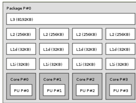
FIGURE 2.1.6 – Topologie d'un microprocesseur multi-cœurs obtenue à l'aide du logiciel hwloc [10].
