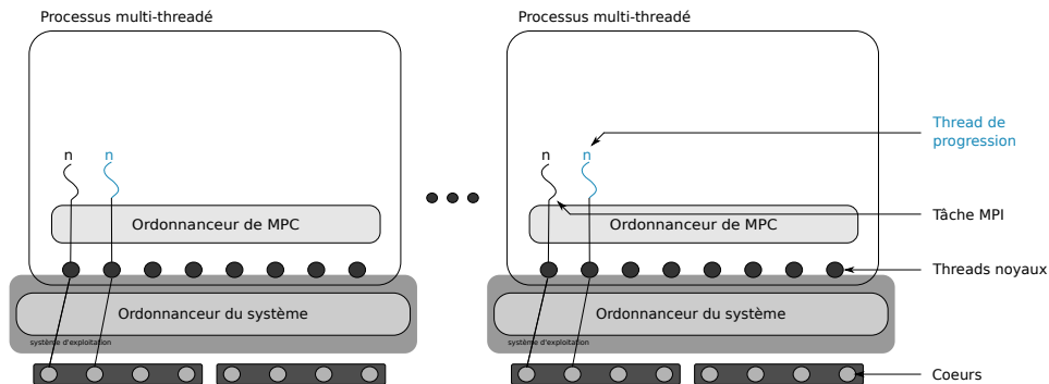
FIGURE 4.3.2 – Placement « dedicated-core »
