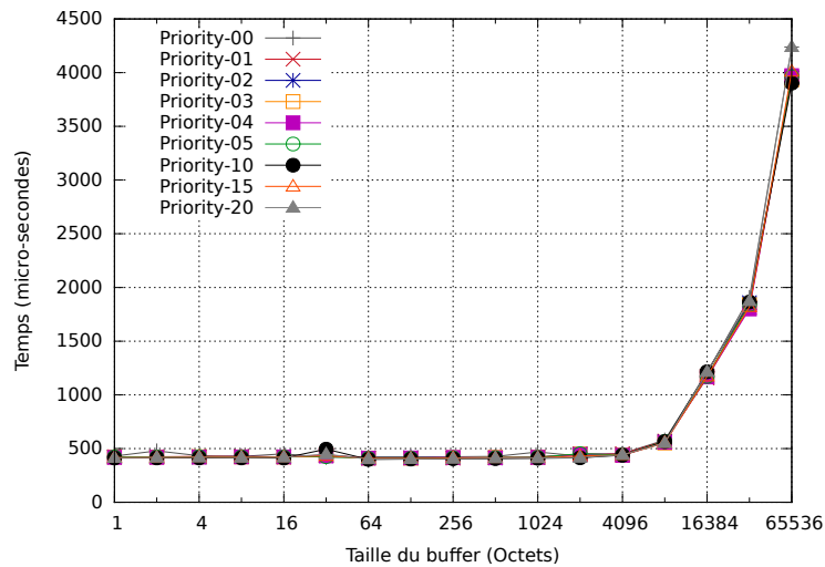
FIGURE 6.4.1 – Temps d'exécution de l'algorithme MPI_Ialltoall avec 64 tâches MPI sur un KNL de 64 cœurs en utilisant le placement « bind »
