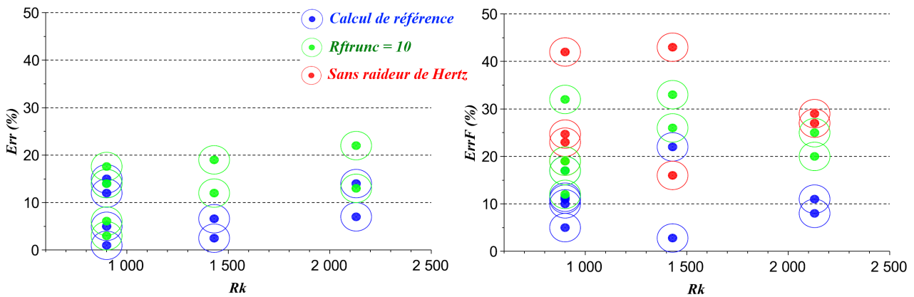
Figure III.22. – Indicateurs Err et Err_F entre les résultats expérimentaux et les calculs éléments finis. En bleu les calculs ont été réalisés avec les valeurs de références, en vert la fréquence de troncature a été abaissée de telle sorte que R_{ftrunc} = 100 et en rouge la loi de contact a été linéarisée
