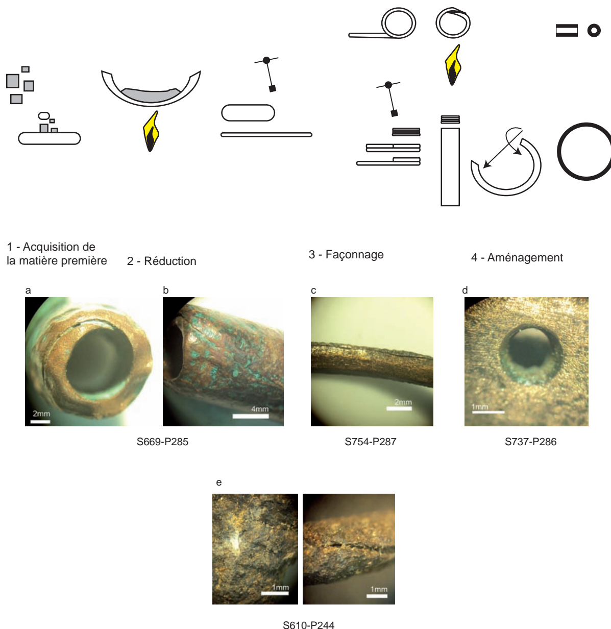
Figure 2.40 : Schéma opératoire des éléments en cuivre
