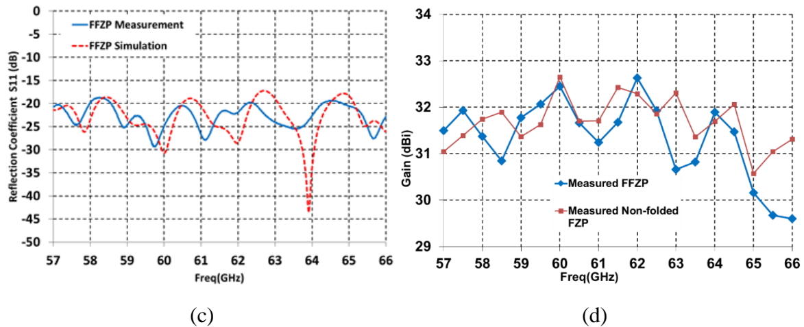
Figure 2: Résultats simulé et mesuré de la lentille de Fresnel repliée (a) diagramme de rayonnement normalise dans plan-E, (b) diagramme de rayonnement normalise dans plan-H, (c) Coefficient de réflexion (S11), et (d) Variation du gain en fonction de la fréquence.
