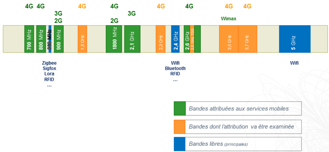
FIGURE 1.2.2 – Répartition des bandes de fréquences pour les différentes technologies de communications sans fil (source : ARCEP)
