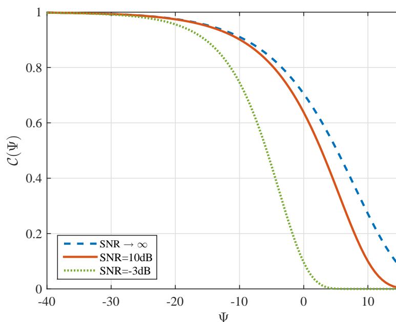
Figure 3.5.4 – Probabilité de couverture théorique pour les DUE en Overlay In-band
