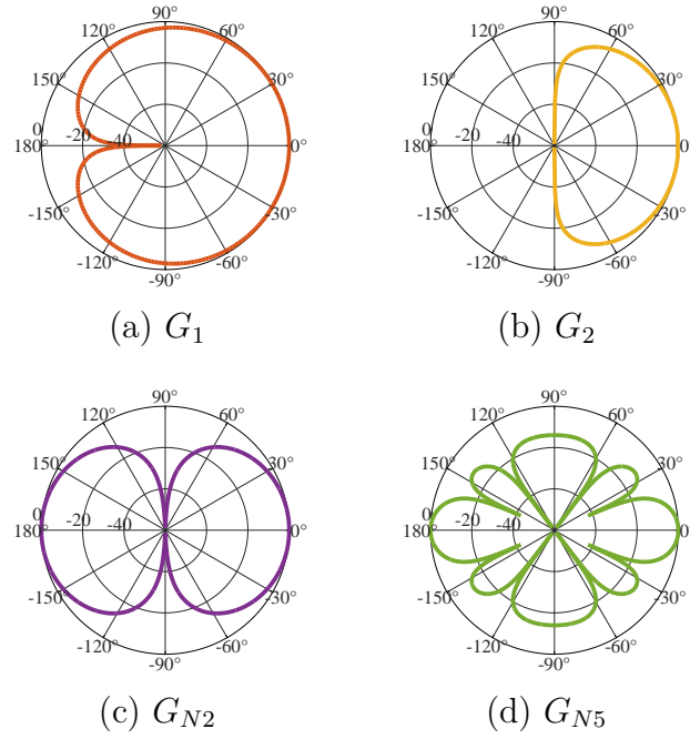
Figure 4.4.1 – Diagramme de rayonnement normalisé des antennes directionnelles (en dB)
