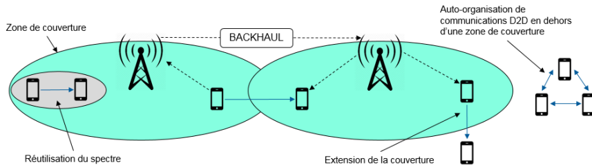
FIGURE 1.1.1 – Illustration de cas possibles d'utilisation du D2D
