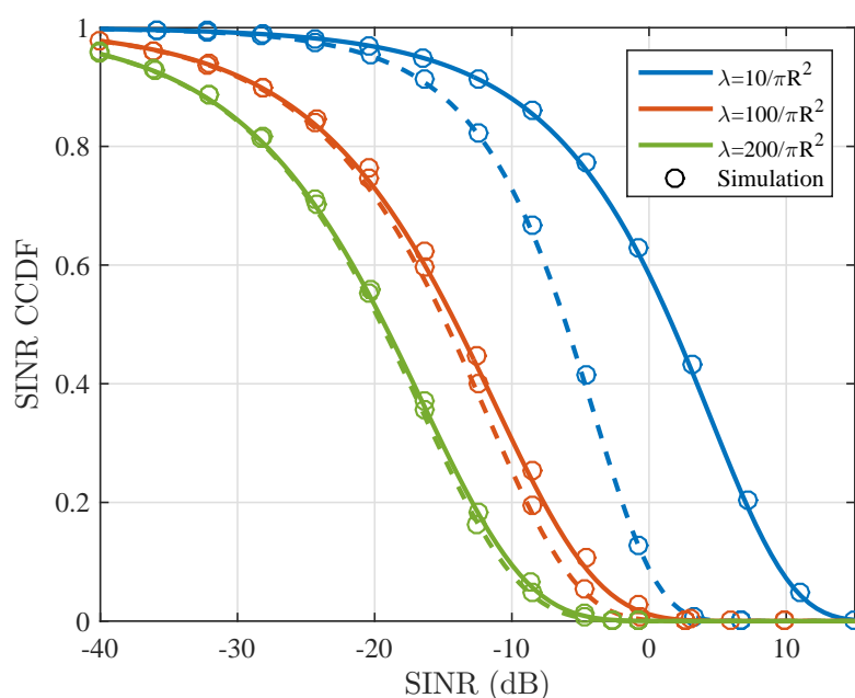
Figure 3.6.1 – CCDF de SINR pour les communications D2D en Inband Overlay avec SNR = 10 dB (ligne pleine) et SNR = -3 dB (ligne pointillée)
