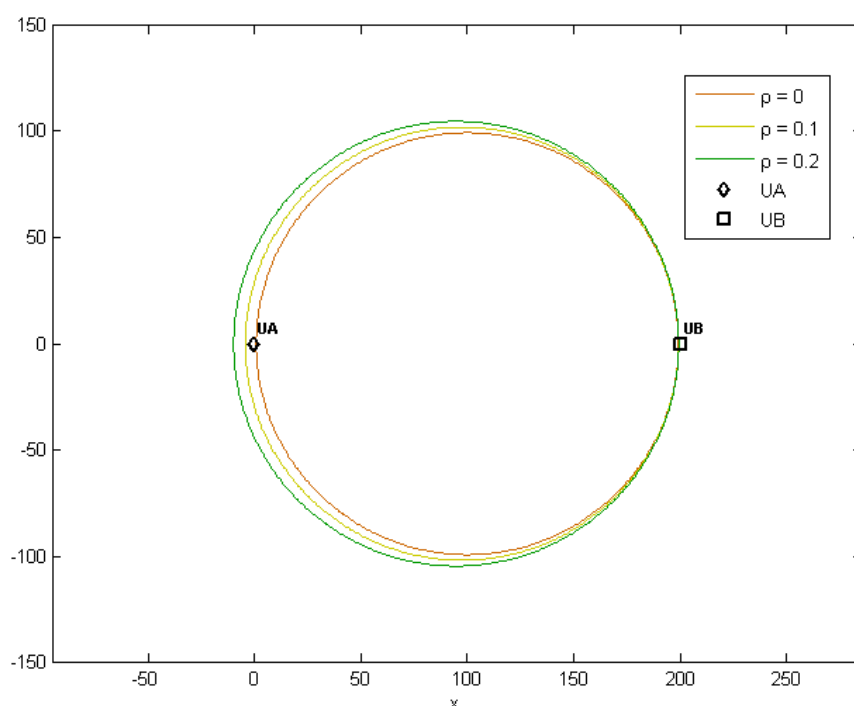
FIGURE 2.4.3 – Influence de la corrélation \rho sur la différence entre E_{DC-DC} et E_{EB-DR-DC} avec \alpha = 2
