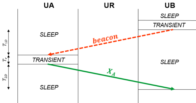
Figure 2.3.1 – Processus temporels des transmissions en topologie DC-DC
