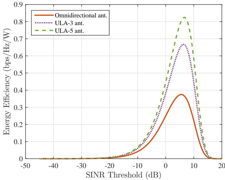
Figure 4.3.4 – Efficacité énergétique pour des liens D2D avec des ULA millimétriques dans un réseau clairsemé, avec \lambda_D = 2 \times (\pi 100^2)^{-1} \text{ m}^{-2} , pour N_A = 1 , N_A = 3 et N_A = 5
