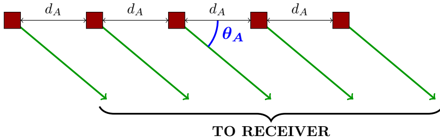
Figure 4.2.1 – ULA. Les carrés rouges et les lignes vertes désignent respectivement les antennes élémentaires et les rayons
