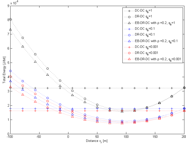
FIGURE 2.6.1 – Consommation énergétique totale pour les topologies DC-DC, DR-DC et EB-DR-DC et en faisant varier x_r , avec \rho = 0.2 , q_b = 1 , q_b = 0.1 et q_b = 0.001
