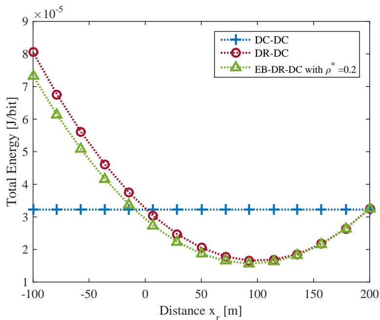
FIGURE 2.5.1 – Consommation totale d'énergie pour les topologies DC-DC, DR-DC et EB-DR-DC avec \rho = 0.2 en faisant varier x_r
