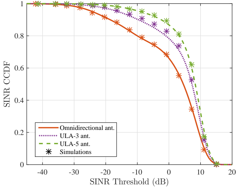
Figure 4.3.2 – Valeurs analytiques et de simulation du CCDF du SINR pour des liens D2D avec des ULA en ondes millimétriques dans un réseau clairsemé, avec \lambda_D = 2 \times (\pi 100^2)^{-1} \text{ m}^{-2} pour N_A = 1 , N_A = 3 et N_A = 5
