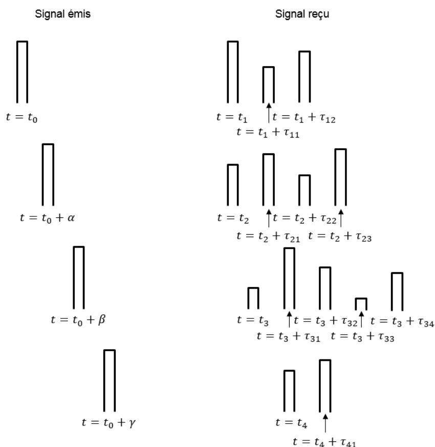
Figure 3.1.1 – Processus temporels des transmissions en topologie DC-DC
