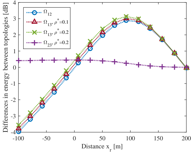
FIGURE 2.5.3 – Différences des consommations totales énergétiques pour les topologies DC-DC, DR-DC et EB-DR-DC en faisant varier la valeur de x_r ( d = 5m )
