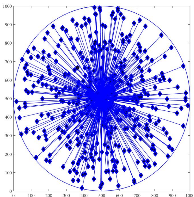
Figure 2.7.1 – Illustration du modèle de réseau pour la configuration CoA. Les diamants bleus sont les UE et les lignes bleues représentent les liens cellulaires
