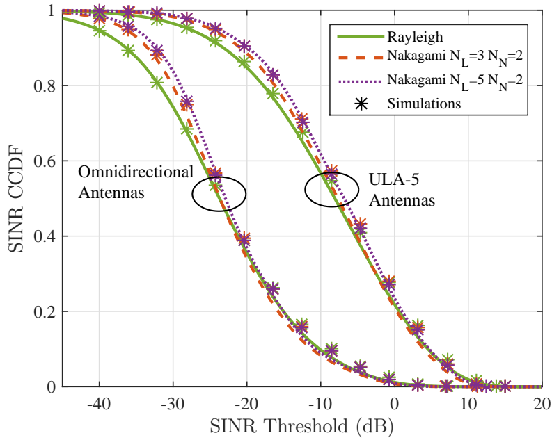
Figure 4.3.6 – Comparaison de la probabilité de couverture pour un canal de Rayleigh et un canal de Nakagami avec N_L = 3 et N_L = 5 ( N_N fixé à 2)
