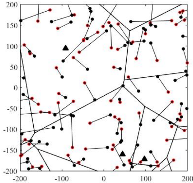
FIGURE 3.2.2 – Modélisation spatiale d'un réseau avec des cellules de Voronoi
