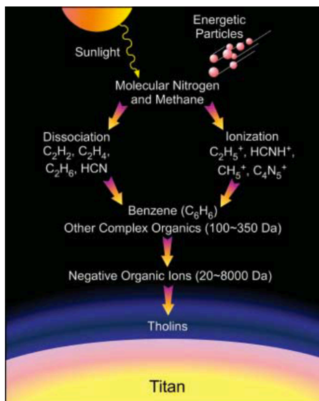
FIGURE B.2: Schéma résumant l'évolution chimique de la haute atmosphère de Titan, qui commence par la dissociation et l'ionisation des deux composés majoritaires, N_2 et CH_4 . Les réactions chimiques se poursuivent plus bas dans l'atmosphère jusqu'à la formation d'aérosols, aussi nommés tholins .
