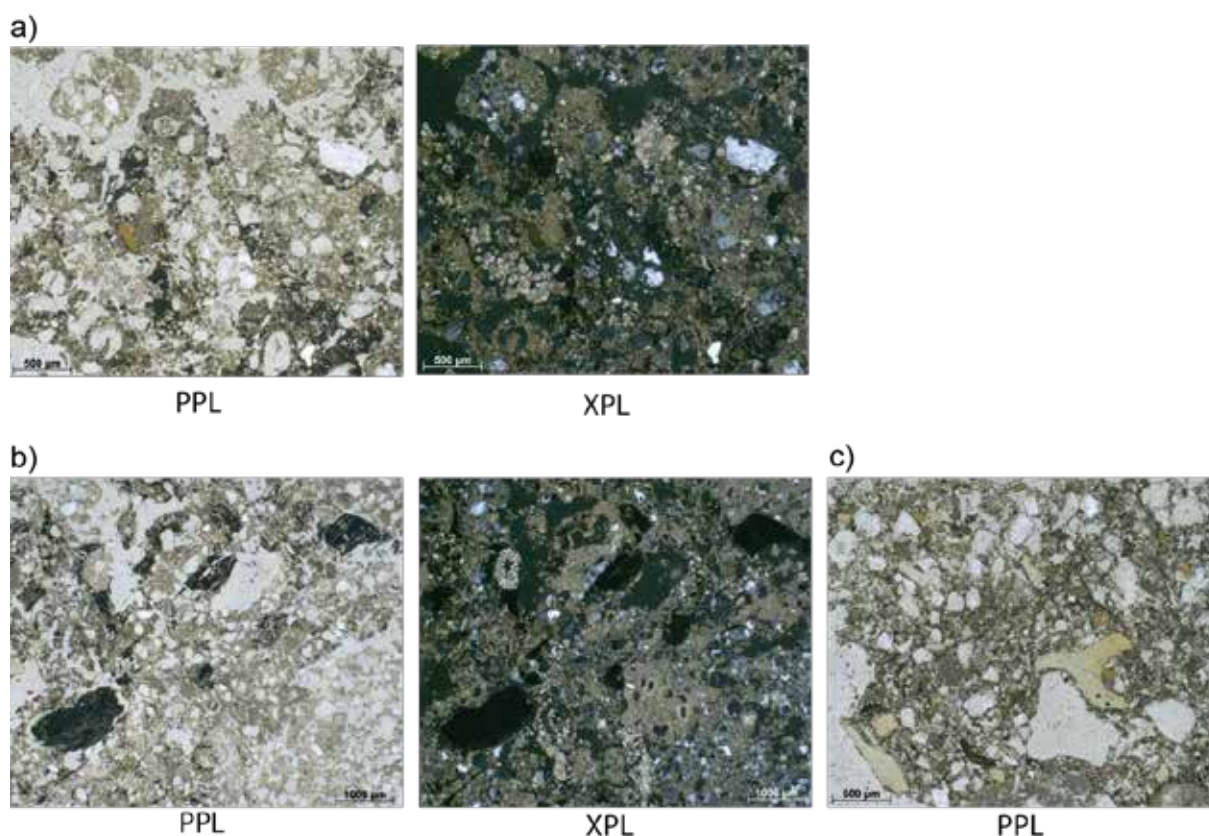
Figure VI.62: Les Bossats, lame mince ORM15 C29. Faciès [2]. a) Microstructure et assemblage du faciès. Noter l'intégration de microcharbons à la micromasse. b) Charbons de bois et calcitisations cytomorphiques dans les chenaux. c) Fragments d'os brûlés à des degrés divers.
