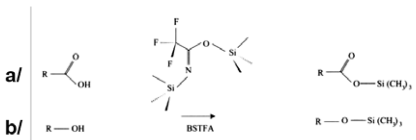
Figure III.29: Exemple de dérivation par silylation appliquée à a/ un acide gras (R-COOH) et b/ un alcool (R-OH) (d'après Pollard et al. , 2007).
