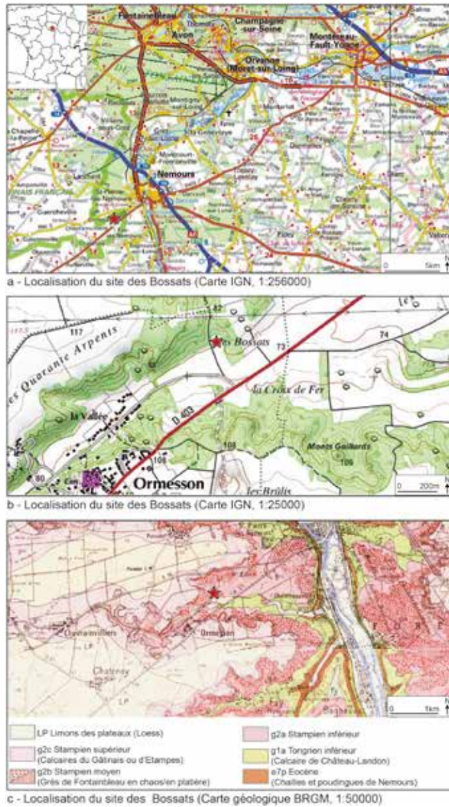
Figure VI.6: Localisation et contexte géologique du site des Bossats (étoile rouge)
