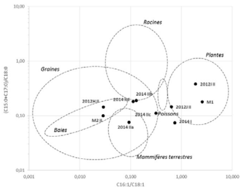
Figure IV.86: Biplot des ratios C_{16:1}/C_{18:1} et (C_{15:0}+C_{17:0})/C_{18:0} (ellipses d'après Eerkens, 2005).
