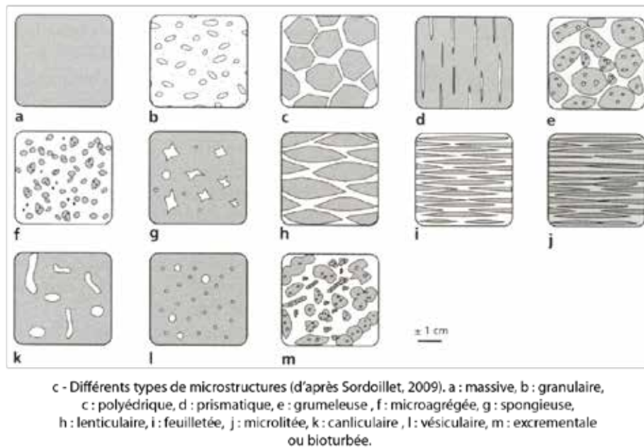
Figure III.5: Différents types de microstructure (d'après Sordoillet, 2009).
