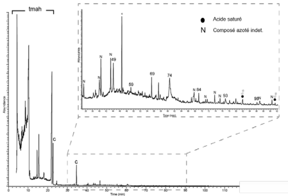
Figure IV.105: Pyrochromatogramme de l'échantillon 2014 I (les numéros renvoient au Tabl. Ann. G.1 ; p, dérivés de plastique et polluants, c, colonne, tmah : dérivés du TMAH ; C x indique le nombre de carbones sur la chaîne linéaire pour les composés les plus courts, les plus longs et les principaux contributeurs de chaque série).
