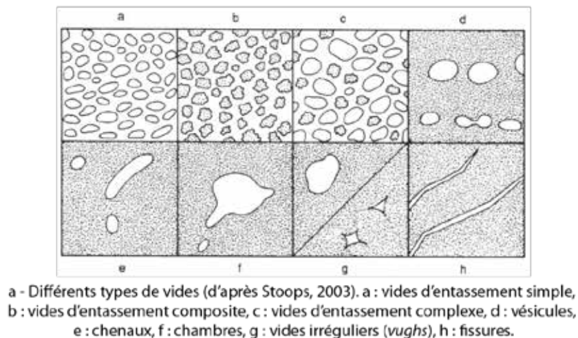
Figure III.3: Différents types de vide (d'après Stoops, 2003).
