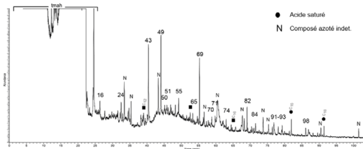
Figure V.112: Pyrochromatogramme de l'échantillon F XII 3 (les numéros renvoient au Tabl. Ann. G.1 ; p, dérivés de plastique et polluants, c, colonne, tmah : dérivés du TMAH ; C_x indique le nombre de carbones sur la chaîne linéaire pour les composés les plus courts, les plus longs et les principaux contributeurs de chaque série).
