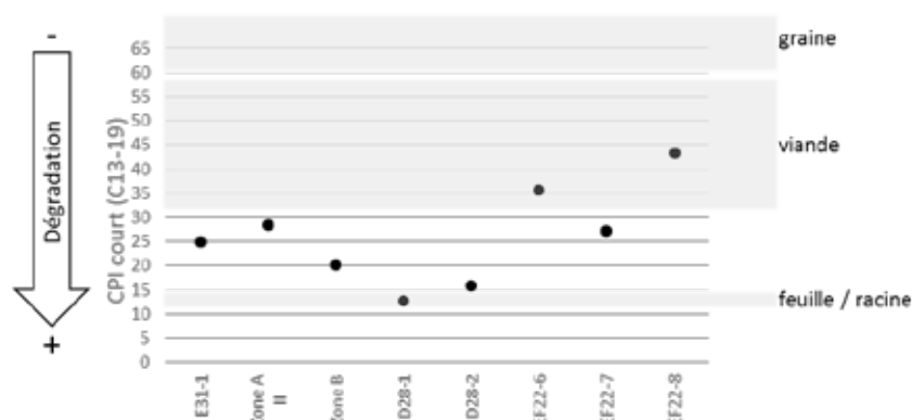
Figure VI.83: Carbon Preference Index des acides courts ( C_{13-19} ) des extraits lipidiques des Bossats. La flèche indique la tendance attendue pour la dégradation (Cooper et Bray, 1963) et les zones grisées les propositions d'attribution d'origine de Lucquin (2007) à partir de son corpus expérimental.
