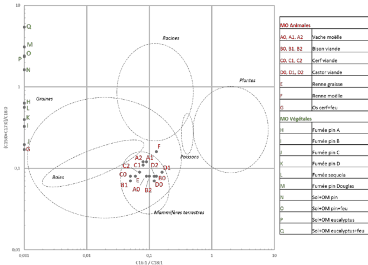
Figure IV.97: Biplot des ratios C_{16:1}/C_{18:1} et (C_{15:0}+C_{17:0})/C_{18:0} des échantillons de référence de MO animales et végétales (ellipses d'après Eerkens, 2005).
