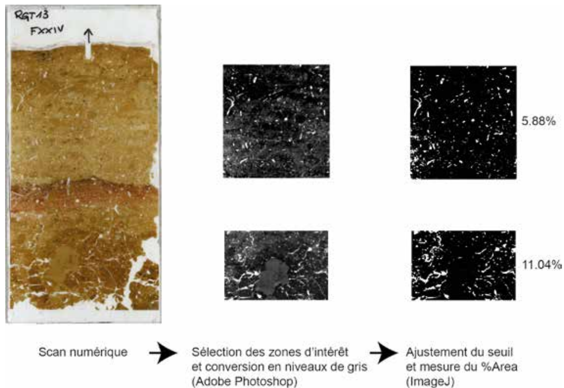
Figure III.4: Mesure approximative de la porosité à partir d'un scan numérique et des logiciels Photoshop et ImageJ.
