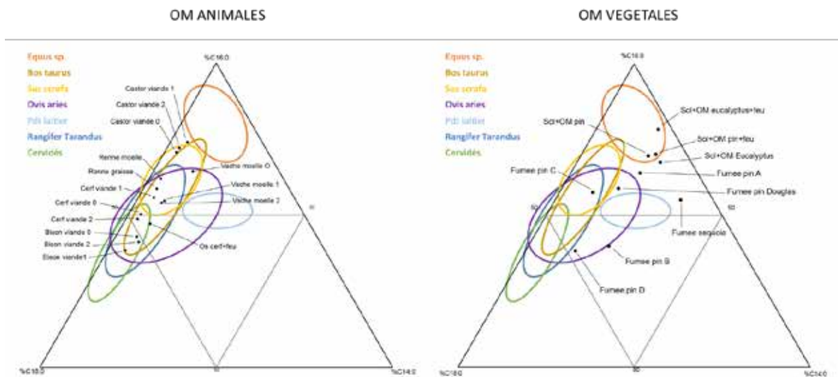
Figure IV.99: Diagramme ternaire des proportions relatives des acides C_{14:0} , C_{16:0} et C_{18:0} des échantillons de référence de MO animales et végétales (ellipses d'après Lucquin, 2007 : compilation des Figures 78 à 83).
