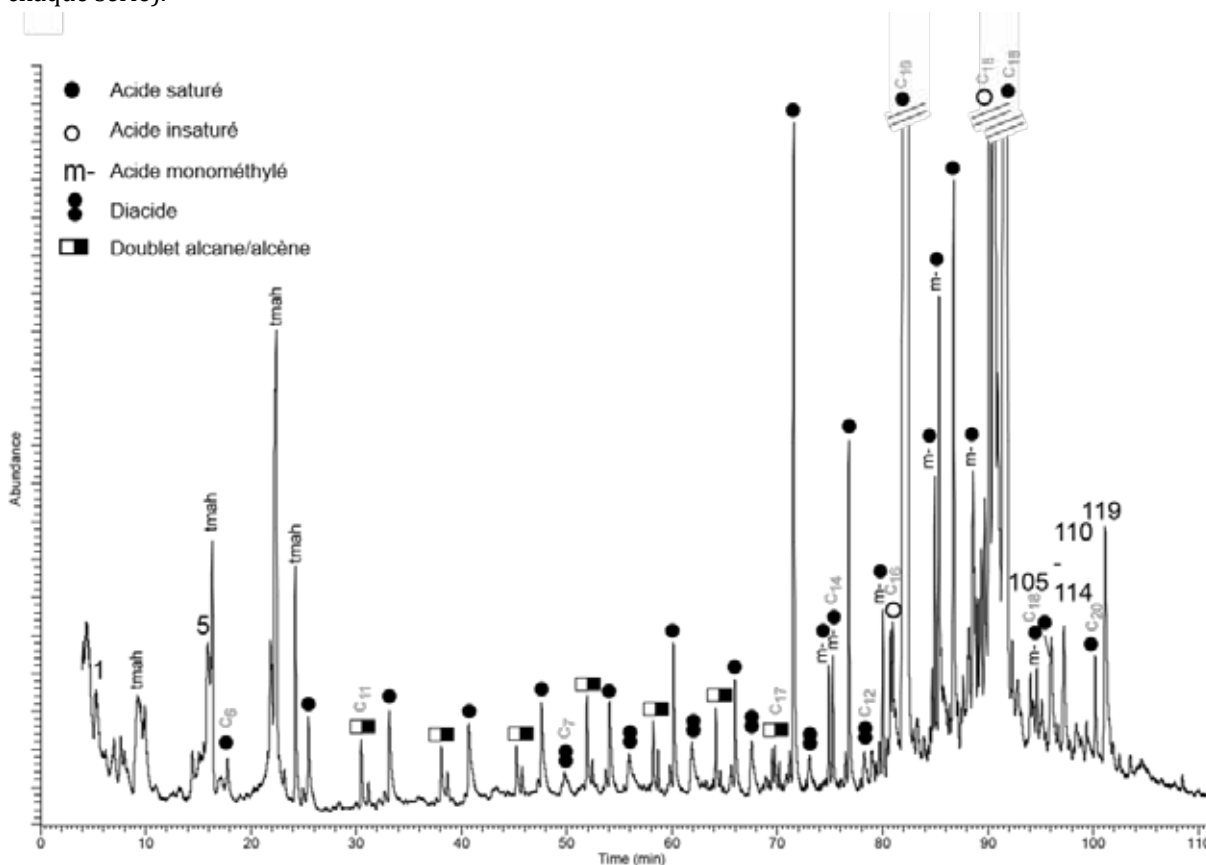
Figure IV.103: Pyrochromatogramme de l'échantillon 2012H II (les numéros renvoient au Tabl. Ann. G.1 ; p, dérivés de plastique et polluants, c, colonne, tmah : dérivés du TMAH ; C x indique le nombre de carbones sur la chaîne linéaire pour les composés les plus courts, les plus longs et les principaux contributeurs de chaque série).
