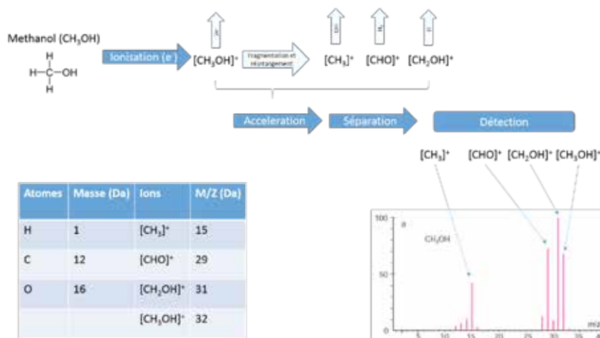
Figure III.33: Exemple de l'ionisation et de la fragmentation du méthanol (d'après Rouessac et Rouessac, 2004 et Silverstein, 2005).
