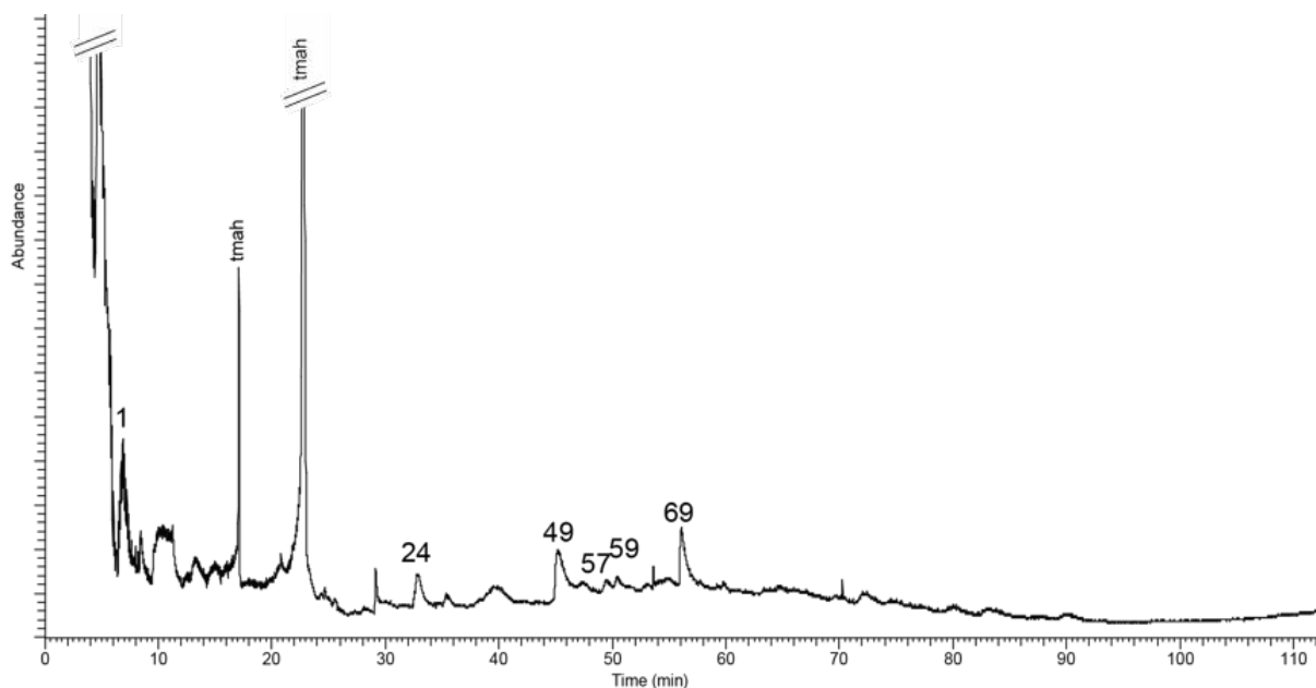
Figure IV.102: Pyrochromatogramme de l'échantillon 2012J II (les numéros renvoient au Tabl. Ann. G.1 ; p, dérivés de plastique et polluants, c, colonne, tmah : dérivés du TMAH ; C x indique le nombre de carbones sur la chaîne linéaire pour les composés les plus courts, les plus longs et les principaux contributeurs de chaque série).
