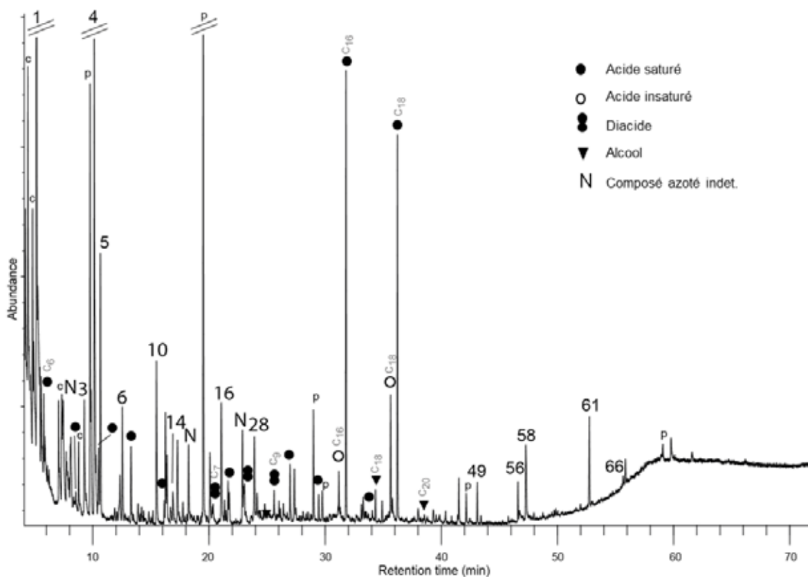
Figure IV.75: TIC de l'échantillon 2014 IIC (les numéros renvoient au Tabl. Ann. F.1; p, dérivés de plastique et polluants, c, colonne ; C x indique le nombre de carbones sur la chaîne linéaire pour les composés les plus courts, les plus longs et les principaux contributeurs de chaque série).
