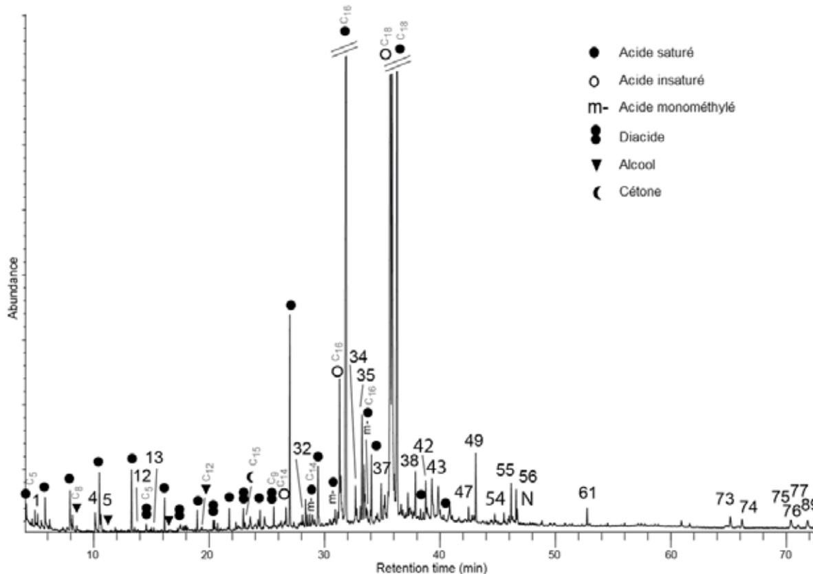
Figure IV.76: TIC de l'échantillon 2014 IID (les numéros renvoient au Tabl. Ann. F.1 ; p, dérivés de plastique et polluants, c, colonne ; C x indique le nombre de carbones sur la chaîne linéaire pour les composés les plus courts, les plus longs et les principaux contributeurs de chaque série).
