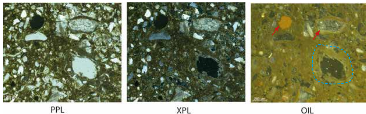
Figure IV.49: Expérimentations, lame mince RGT12 2012G ; faible oxydation d'un hyporevêtement calcitique par rapport à la micromasse argilocalcarbonatée (tirets bleus). Noter, à l'inverse, celle des deux grains calcaires en haut des images (flèches rouges).
