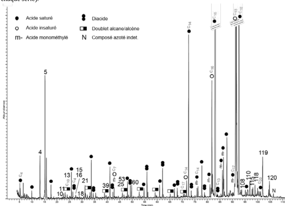
Figure IV.107: Pyrochromatogramme de l'échantillon 2014 I Ib (les numéros renvoient au Tabl. Ann. G.1 ; p, dérivés de plastique et polluants, c, colonne, tmah : dérivés du TMAH ; C x indique le nombre de carbones sur la chaîne linéaire pour les composés les plus courts, les plus longs et les principaux contributeurs de chaque série).
