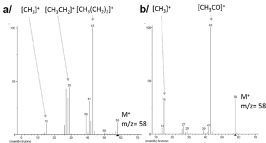
Figure III.34: Exemple de fragmentogrammes pour un ion moléculaire de m/z = 58 . a/ butane ( C_4H_{10} ). b/ Acétone ( C_3H_6O ).
